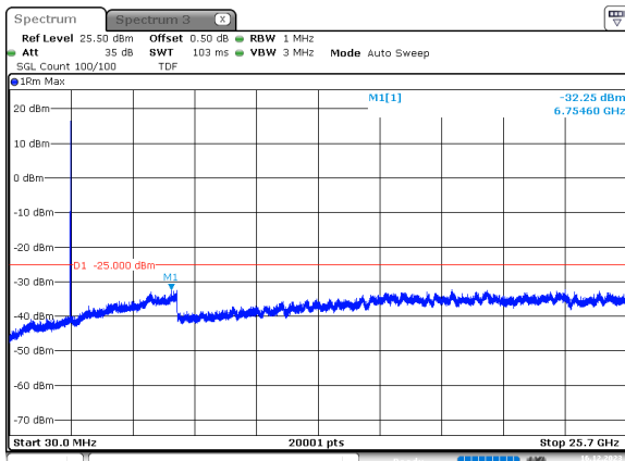
20MHz_15kHz_2560MHz_DFT-s-OFDM QPSK_RB1@0 -32.25 dBm
