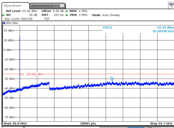
5MHz_15kHz_2535MHz_DFT-s-OFDM QPSK_RB25@0 -32.25 dBm
