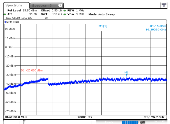
20MHz_15kHz_2535MHz_DFT-s-OFDM QPSK_RB1@0 -31.15 dBm
