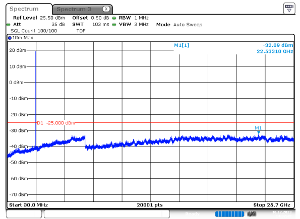
20MHz_15kHz_2510MHz_DFT-s-OFDM QPSK_RB1@105 -32.09 dBm
