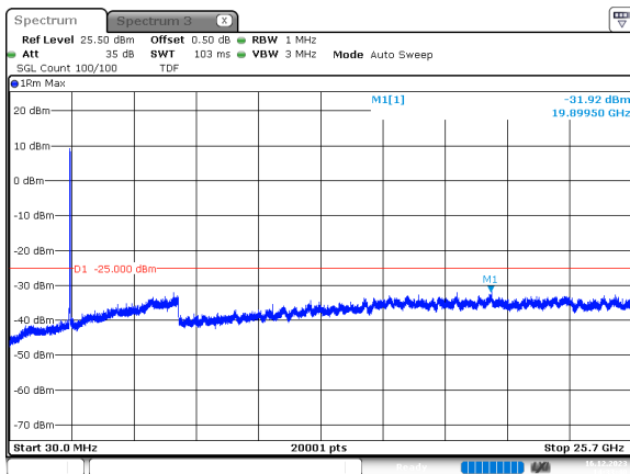
20MHz_15kHz_2510MHz_DFT-s-OFDM QPSK_RB100@0 -31.92 dBm
