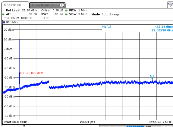
20MHz_15kHz_2560MHz_DFT-s-OFDM QPSK_RB100@0 -32.34 dBm
