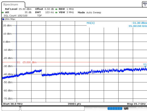
20MHz_15kHz_2510MHz_DFT-s-OFDM QPSK_RB1@0 -31.30 dBm
