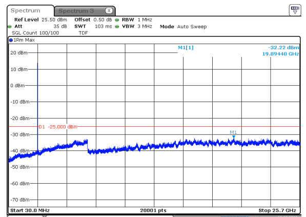
5MHz_15kHz_2567.5MHz_DFT-s-OFDM QPSK_RB25@0 -32.22 dBm
