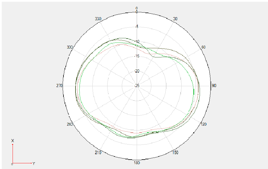
WCDMA B1/LTE B1/N1 \Theta=90^\circ
