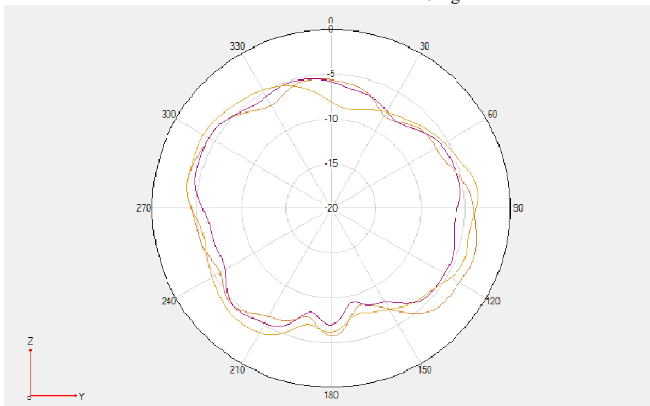
WCDMA B1/LTE B1/N1 \Phi=90^\circ
