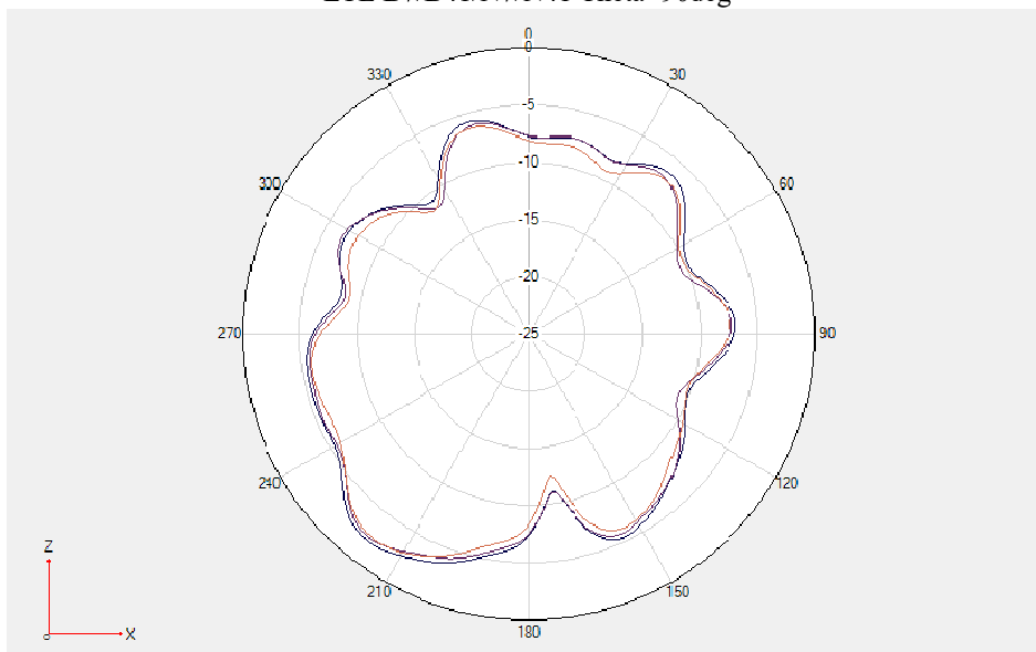
LTE B38/N38 \Phi=0^\circ
