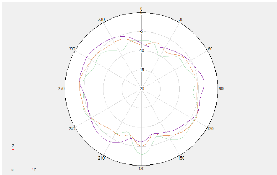
WCDMA B4/LTE B4/B66/N66 \Phi=90^\circ
