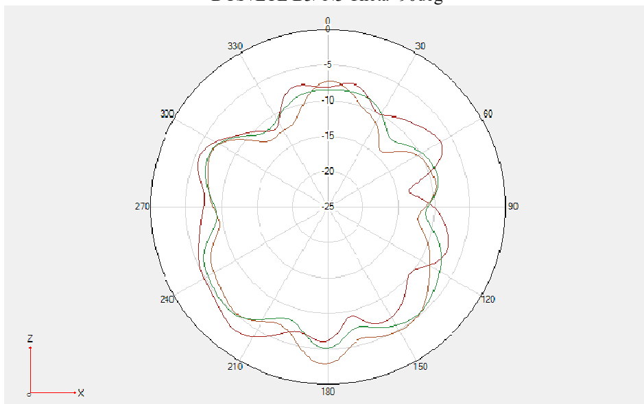
WCDMA B4/LTE B4/B66/N66 \Phi = 0^\circ
