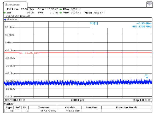
40MHz_15kHz_3960MHz_DFT-s-OFDM QPSK_RB1@215&-46.55 dBm
