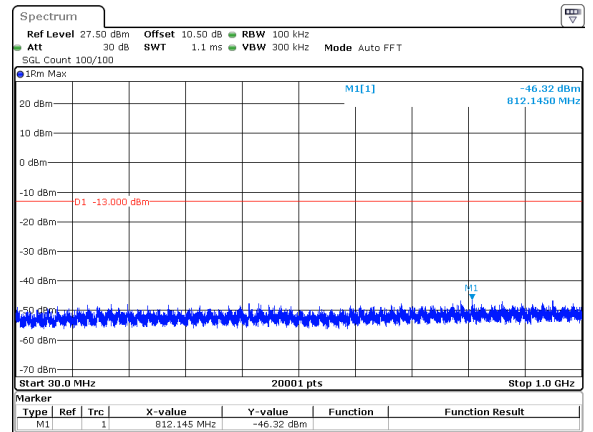
10MHz_30kHz_3455MHz_DFT-s-OFDM QPSK_RB1@0&-46.32 dBm
