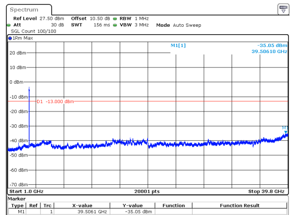
60MHz_30kHz_3950MHz_DFT-s-OFDM QPSK_RB162@0&-35.05 dBm
