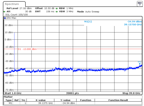
20MHz_30kHz_3970MHz_DFT-s-OFDM QPSK_RB1@0&-34.94 dBm
