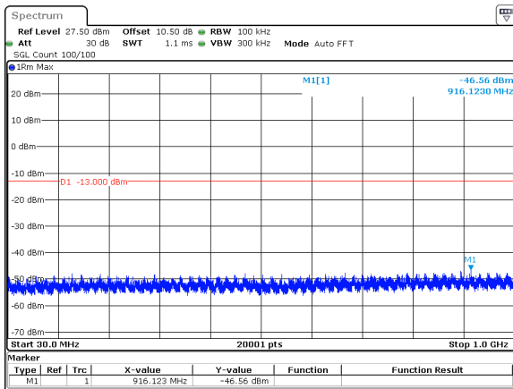
40MHz_15kHz_3720MHz_DFT-s-OFDM QPSK_RB1@215&-46.56 dBm
