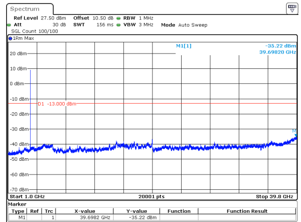
20MHz_30kHz_3970MHz_DFT-s-OFDM QPSK_RB1@50&-35.22 dBm
