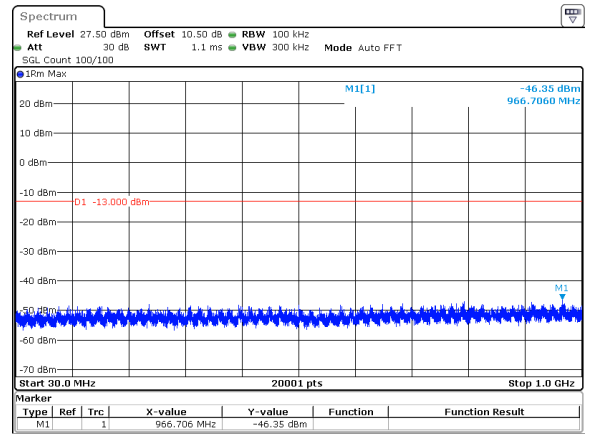
30MHz_15kHz_3965MHz_DFT-s-OFDM QPSK_RB1@0&-46.35 dBm
