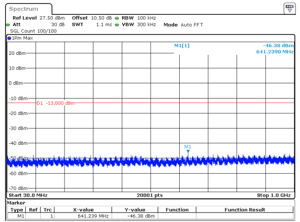
100MHz_30kHz_3750MHz_DFT-s-OFDM QPSK_RB1@0&-46.38 dBm
