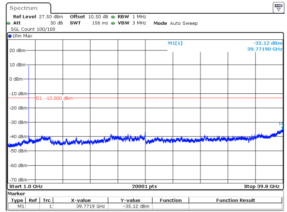
50MHz_15kHz_3955MHz_DFT-s-OFDM QPSK_RB1@0&-35.12 dBm
