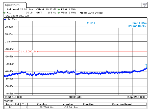
40MHz_15kHz_3960MHz_DFT-s-OFDM QPSK_RB216@0&-35.34 dBm
