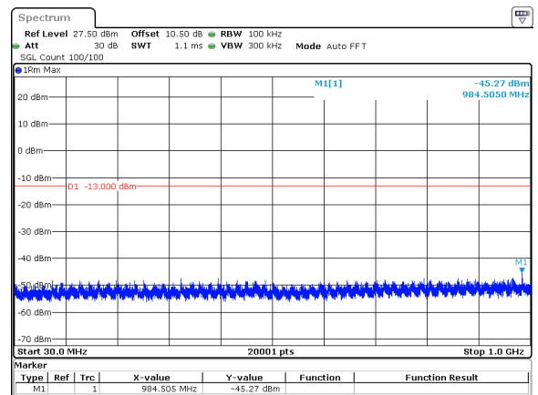
80MHz_30kHz_3940MHz_DFT-s-OFDM QPSK_RB216@0&-45.27 dBm
