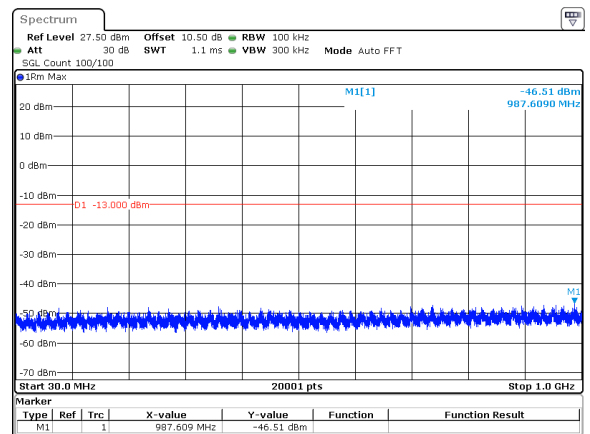
50MHz_15kHz_3955MHz_DFT-s-OFDM QPSK_RB270@0&-46.51 dBm
