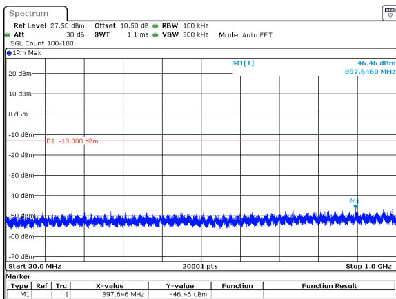
40MHz_15kHz_3960MHz_DFT-s-OFDM QPSK_RB216@0&-46.46 dBm
