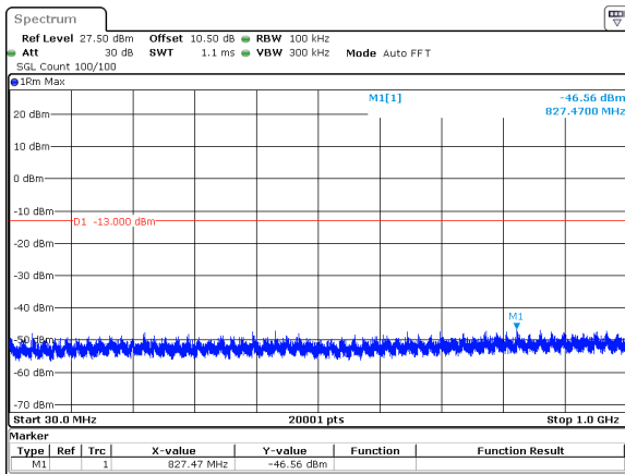
50MHz_30kHz_3955MHz_DFT-s-OFDM QPSK_RB1@132&-46.56 dBm
