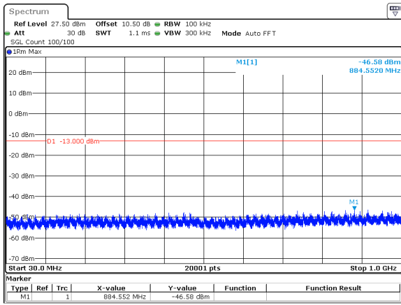
70MHz_30kHz_3945MHz_DFT-s-OFDM QPSK_RB1@0&-46.58 dBm
