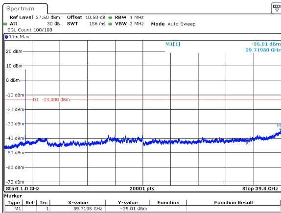
90MHz_30kHz_3935MHz_DFT-s-OFDM QPSK_RB1@244&-35.01 dBm
