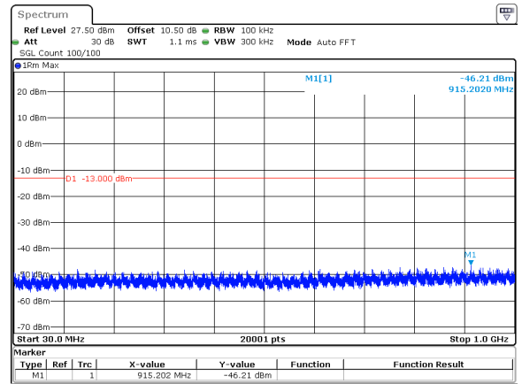
20MHz_30kHz_3840MHz_DFT-s-OFDM QPSK_RB1@0&-46.21 dBm
