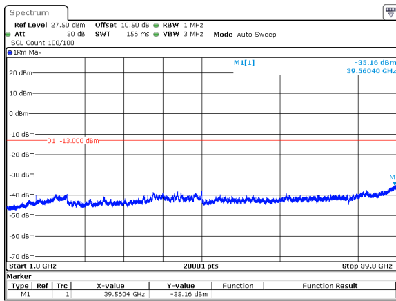
100MHz_30kHz_3930MHz_DFT-s-OFDM QPSK_RB1@272&-35.16 dBm
