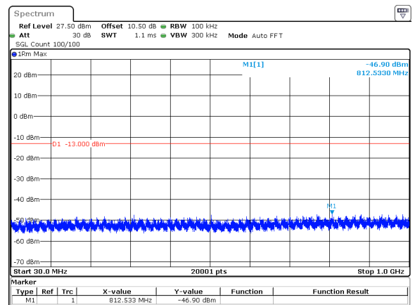
90MHz_30kHz_3935MHz_DFT-s-OFDM QPSK_RB243@0&-46.90 dBm
