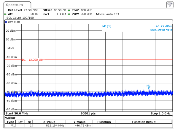
60MHz_30kHz_3950MHz_DFT-s-OFDM QPSK_RB1@0&-46.79 dBm
