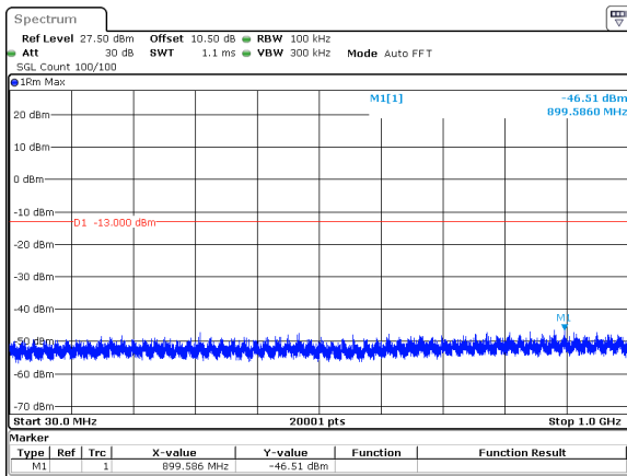
20MHz_30kHz_3840MHz_DFT-s-OFDM QPSK_RB1@50&-46.51 dBm
