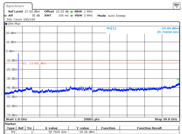
30MHz_15kHz_3965MHz_DFT-s-OFDM QPSK_RB160@0&-35.06 dBm
