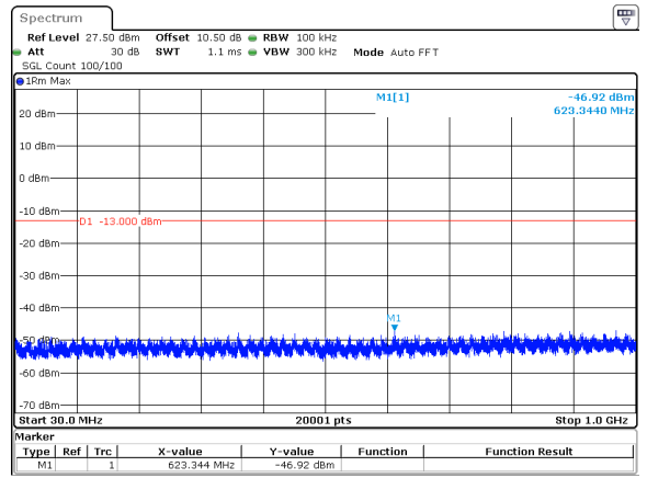
70MHz_30kHz_3735MHz_DFT-s-OFDM QPSK_RB1@0&-46.92 dBm
