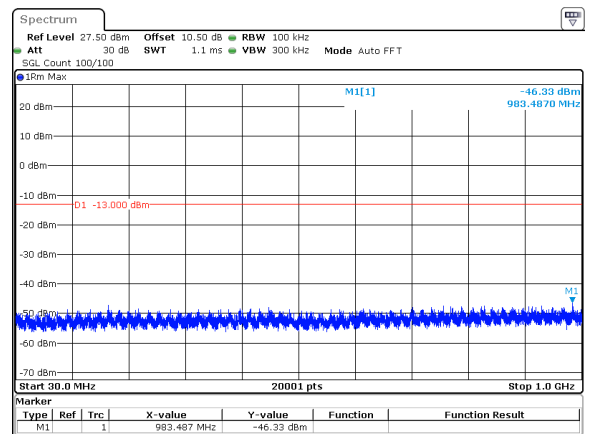
90MHz_30kHz_3745MHz_DFT-s-OFDM QPSK_RB243@0&-46.33 dBm
