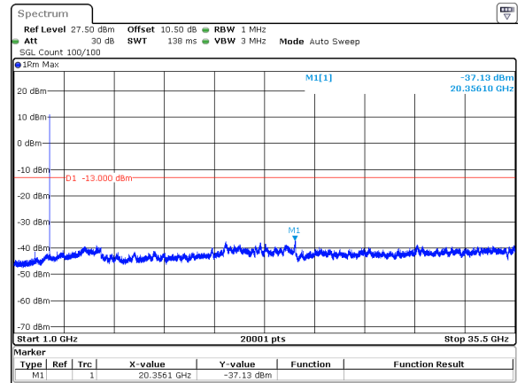
10MHz_30kHz_3455MHz_DFT-s-OFDM QPSK_RB1@23&-37.13 dBm
