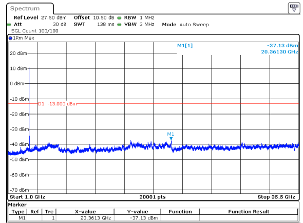
10MHz_30kHz_3500MHz_DFT-s-OFDM QPSK_RB1@0&-37.13 dBm
