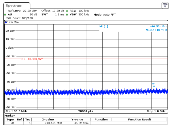
10MHz_30kHz_3500MHz_DFT-s-OFDM QPSK_RB24@0&-46.52 dBm
