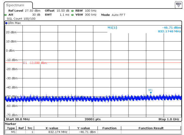
40MHz_15kHz_3960MHz_DFT-s-OFDM QPSK_RB1@0&-46.71 dBm
