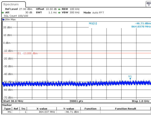
60MHz_30kHz_3730MHz_DFT-s-OFDM QPSK_RB1@0&-46.71 dBm
