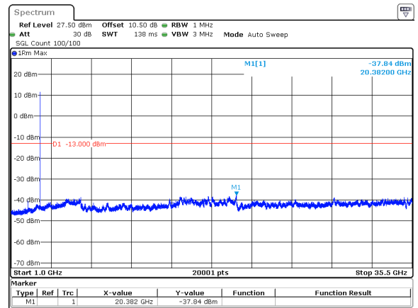
10MHz_30kHz_3500MHz_DFT-s-OFDM QPSK_RB1@23&-37.84 dBm
