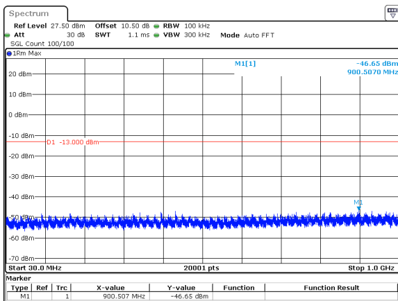
40MHz_15kHz_3720MHz_DFT-s-OFDM QPSK_RB216@0&-46.65 dBm
