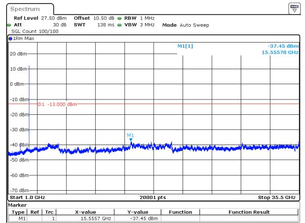
10MHz_30kHz_3500MHz_DFT-s-OFDM QPSK_RB1@23&-37.45 dBm
