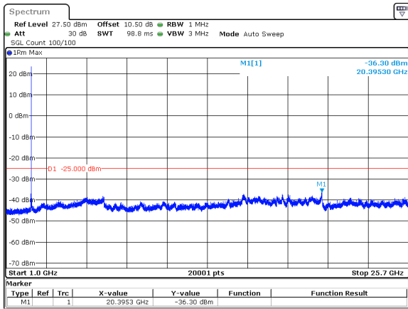
20MHz_15kHz_2535MHz_DFT-s-OFDM QPSK_RB1@0&-36.30 dBm
