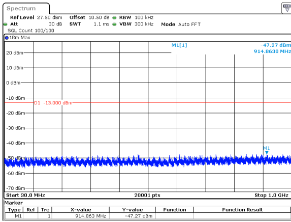
20MHz_30kHz_3500MHz_DFT-s-OFDM QPSK_RB1@0&-47.27 dBm
