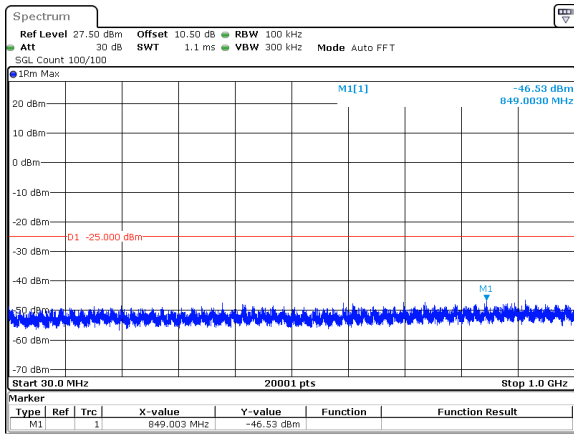
10MHz_15kHz_2535MHz_DFT-s-OFDM QPSK_RB1@0&-46.53 dBm
