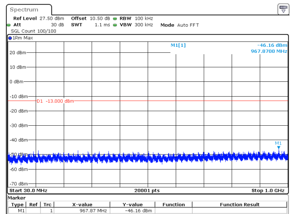
10MHz_15kHz_3500MHz_DFT-s-OFDM QPSK_RB50@0&-46.16 dBm
