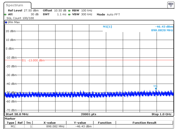
20MHz_30kHz_3460MHz_DFT-s-OFDM QPSK_RB1@50&-46.43 dBm
