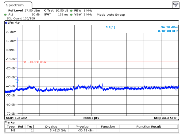
10MHz_30kHz_3455MHz_DFT-s-OFDM QPSK_RB1@0&-36.78 dBm
