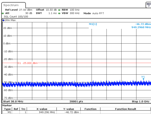
10MHz_15kHz_2535MHz_DFT-s-OFDM QPSK_RB50@0&-46.72 dBm
