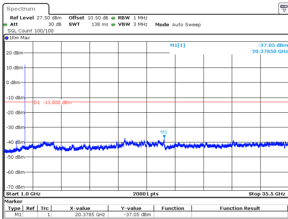
10MHz_15kHz_3500MHz_DFT-s-OFDM QPSK_RB1@51&-37.05 dBm
