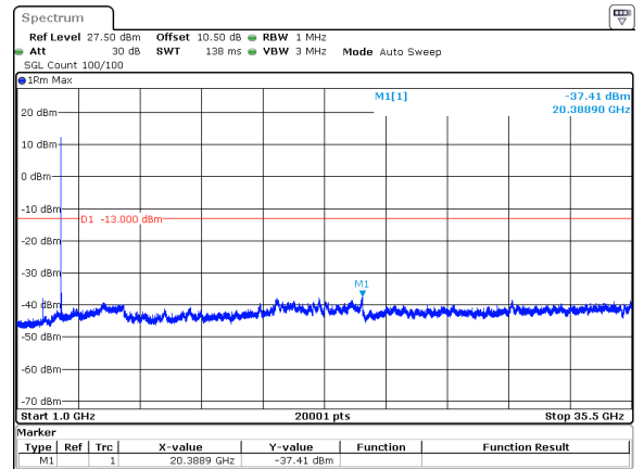
10MHz_15kHz_3455MHz_DFT-s-OFDM QPSK_RB1@0&-37.41 dBm
