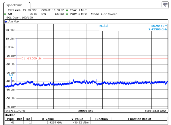
10MHz_15kHz_3455MHz_DFT-s-OFDM QPSK_RB1@51&-36.92 dBm
