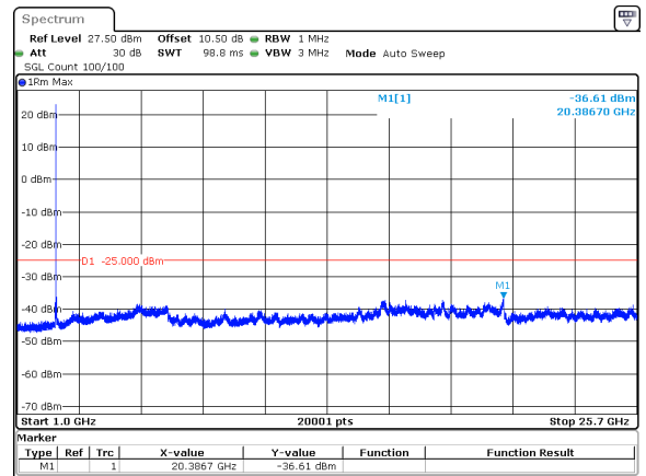
20MHz_15kHz_2535MHz_DFT-s-OFDM QPSK_RB1@105&-36.61 dBm
