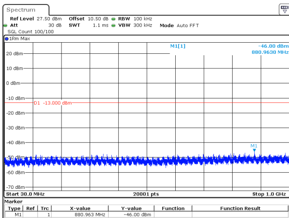
40MHz_15kHz_3470MHz_DFT-s-OFDM QPSK_RB216@0&-46.00 dBm
