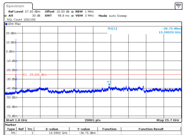
20MHz_15kHz_2535MHz_DFT-s-OFDM QPSK_RB100@0&-36.75 dBm
