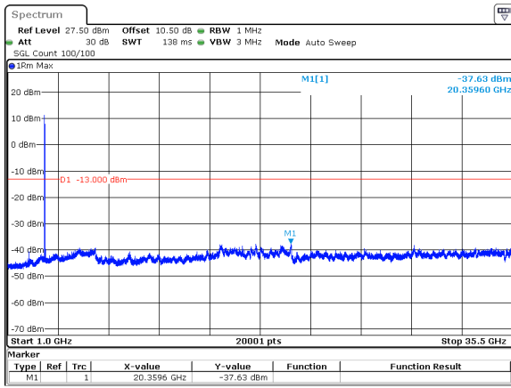
40MHz_30kHz_3530MHz_DFT-s-OFDM QPSK_RB1@0&-37.63 dBm
