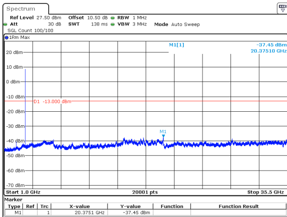
20MHz_30kHz_3540MHz_DFT-s-OFDM QPSK_RB1@50&-37.45 dBm
