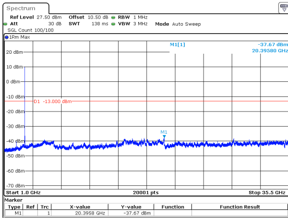
20MHz_30kHz_3460MHz_DFT-s-OFDM QPSK_RB1@0&-37.67 dBm
