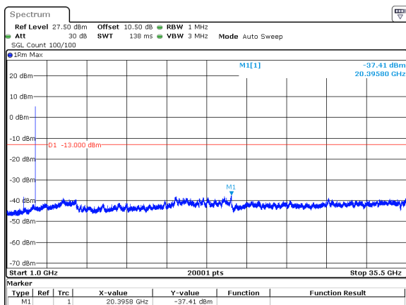
10MHz_15kHz_3455MHz_DFT-s-OFDM QPSK_RB50@0&-37.41 dBm
