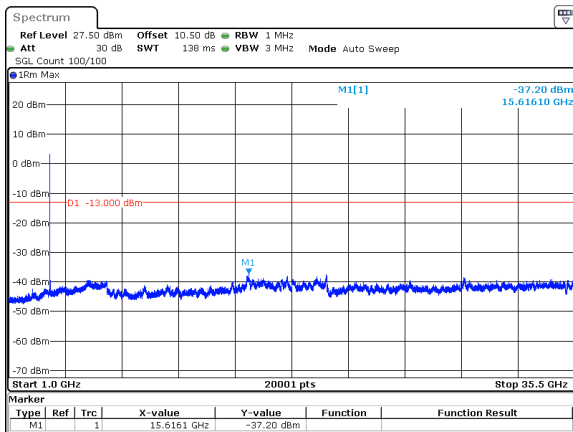
20MHz_15kHz_3500MHz_DFT-s-OFDM QPSK_RB100@0&-37.20 dBm
