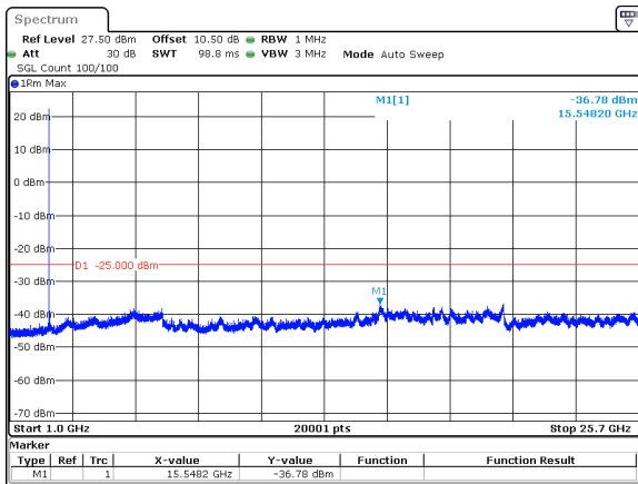
10MHz_15kHz_2535MHz_DFT-s-OFDM QPSK_RB1@51&-36.78 dBm
