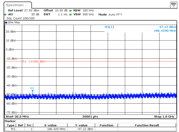
20MHz_30kHz_3460MHz_DFT-s-OFDM QPSK_RB1@0&-47.12 dBm
