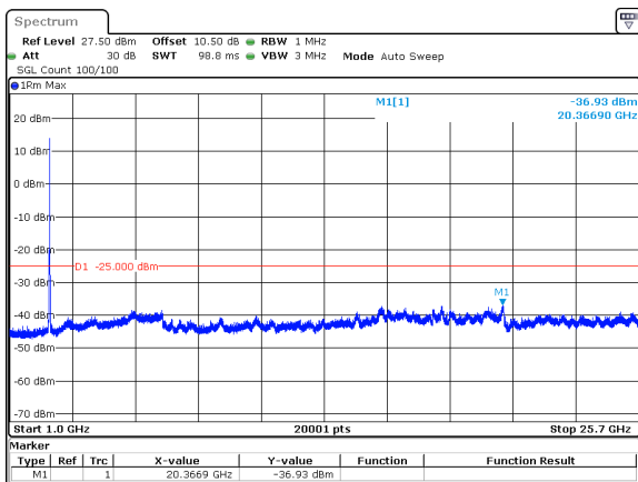
20MHz_15kHz_2560MHz_DFT-s-OFDM QPSK_RB100@0&-36.93 dBm
