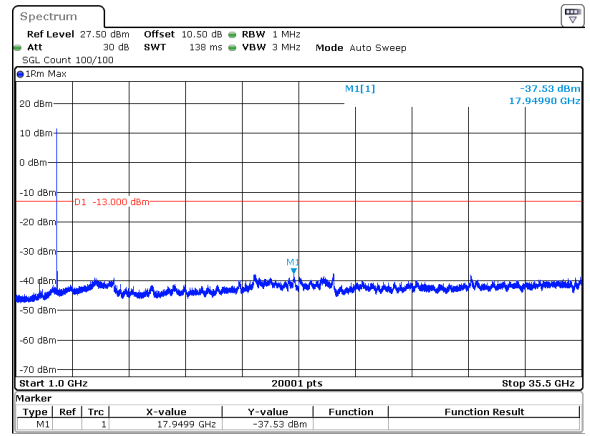
20MHz_30kHz_3500MHz_DFT-s-OFDM QPSK_RB1@0&-37.53 dBm
