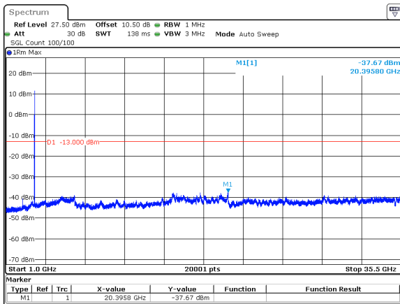
20MHz_30kHz_3460MHz_DFT-s-OFDM QPSK_RB1@50&-37.67 dBm
