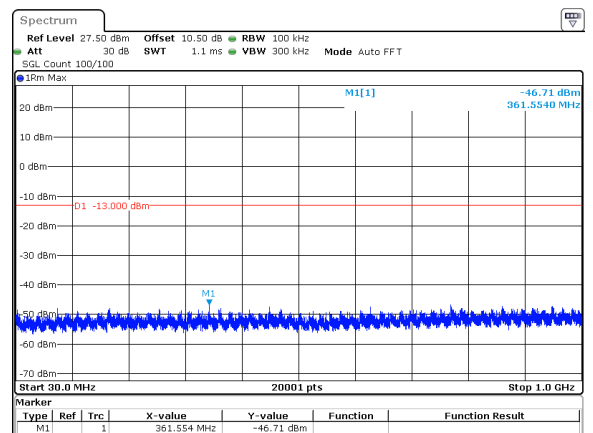
10MHz_15kHz_3455MHz_DFT-s-OFDM QPSK_RB50@0&-46.71 dBm
