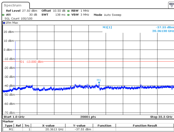
30MHz_15kHz_3535MHz_DFT-s-OFDM QPSK_RB1@159&-37.55 dBm
