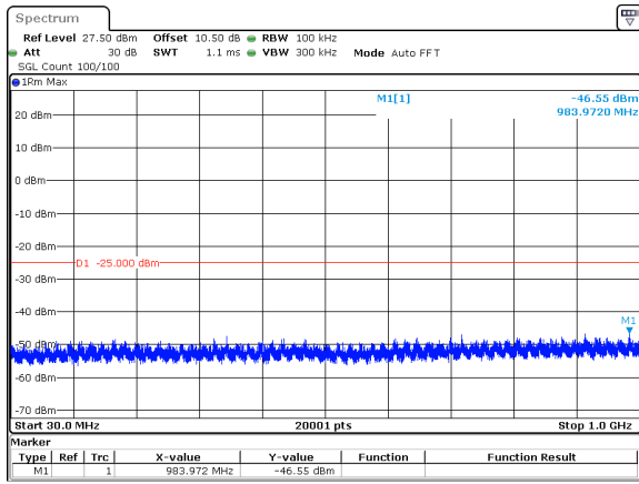
10MHz_15kHz_2565MHz_DFT-s-OFDM QPSK_RB1@0&-46.55 dBm
