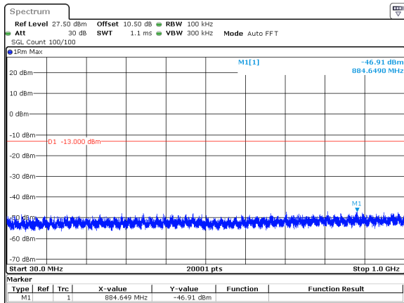
10MHz_15kHz_3455MHz_DFT-s-OFDM QPSK_RB1@0&-46.91 dBm
