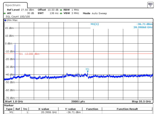
40MHz_15kHz_3530MHz_DFT-s-OFDM QPSK_RB216@0&-36.71 dBm
