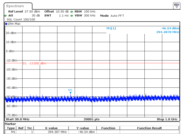
20MHz_15kHz_3460MHz_DFT-s-OFDM QPSK_RB100@0&-46.54 dBm
