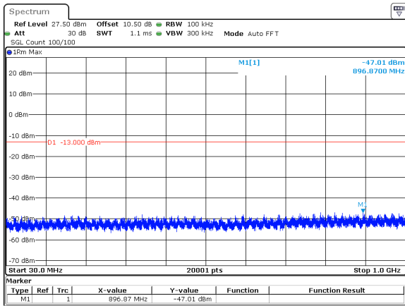
40MHz_15kHz_3470MHz_DFT-s-OFDM QPSK_RB1@0&-47.01 dBm
