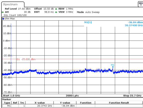
20MHz_15kHz_2510MHz_DFT-s-OFDM QPSK_RB1@105&-36.84 dBm
