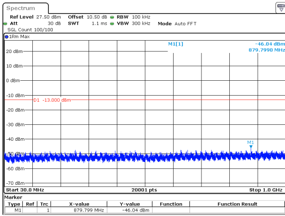
40MHz_30kHz_3470MHz_DFT-s-OFDM QPSK_RB1@0&-46.04 dBm
