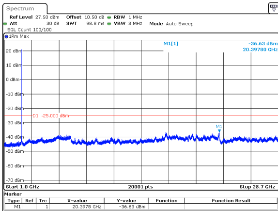
20MHz_15kHz_2560MHz_DFT-s-OFDM QPSK_RB1@105&-36.63 dBm
