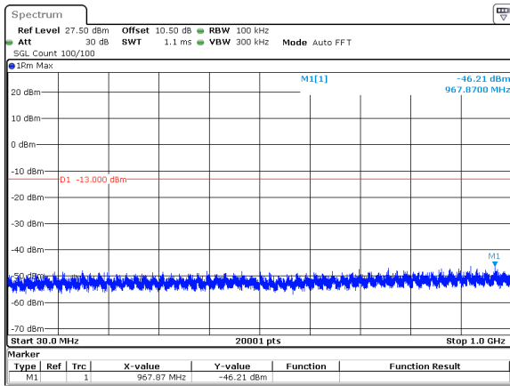
20MHz_15kHz_3500MHz_DFT-s-OFDM QPSK_RB1@0&-46.21 dBm
