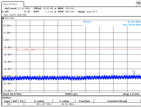
10MHz_30kHz_3455MHz_DFT-s-OFDM QPSK_RB1@0&-46.95 dBm
