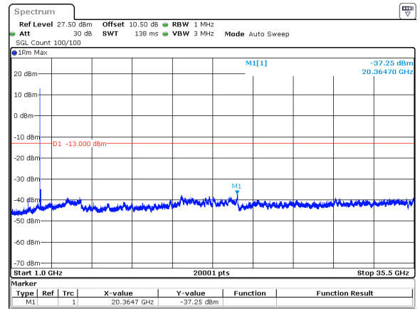
40MHz_15kHz_3470MHz_DFT-s-OFDM QPSK_RB1@0&-37.25 dBm
