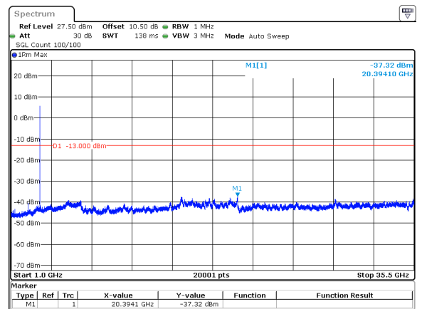
10MHz_30kHz_3455MHz_DFT-s-OFDM QPSK_RB24@0&-37.32 dBm
