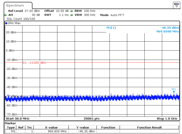
40MHz_15kHz_3470MHz_DFT-s-OFDM QPSK_RB1@215&-46.35 dBm
