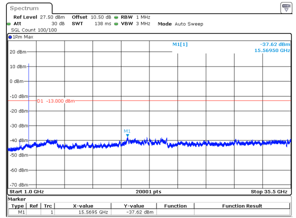
20MHz_30kHz_3540MHz_DFT-s-OFDM QPSK_RB1@0&-37.62 dBm
