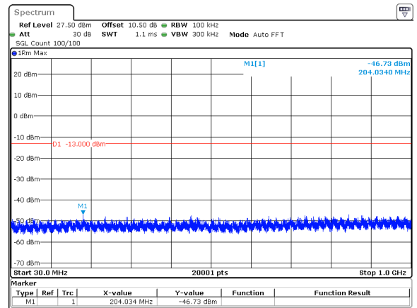
20MHz_30kHz_3500MHz_DFT-s-OFDM QPSK_RB1@50&-46.73 dBm
