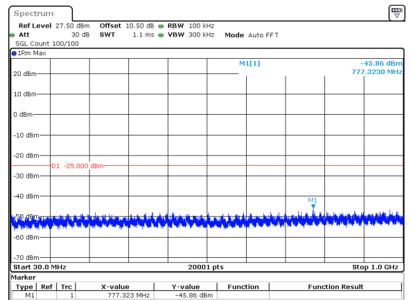
10MHz_15kHz_2565MHz_DFT-s-OFDM QPSK_RB50@0&-45.86 dBm
