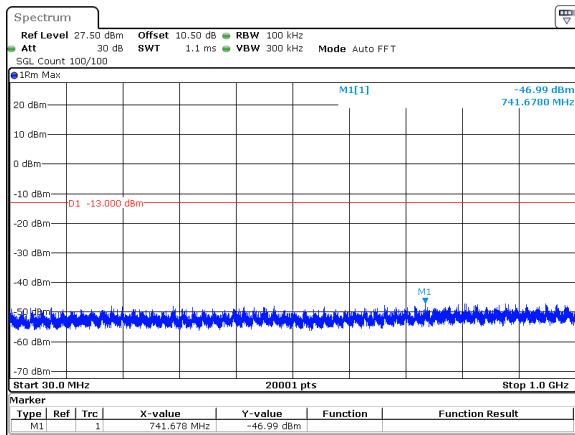
10MHz_30kHz_3500MHz_DFT-s-OFDM QPSK_RB1@23&-46.99 dBm
