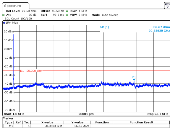
10MHz_15kHz_2565MHz_DFT-s-OFDM QPSK_RB50@0&-36.67 dBm
