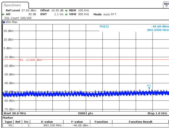
10MHz_30kHz_3455MHz_DFT-s-OFDM QPSK_RB1@23&-46.68 dBm
