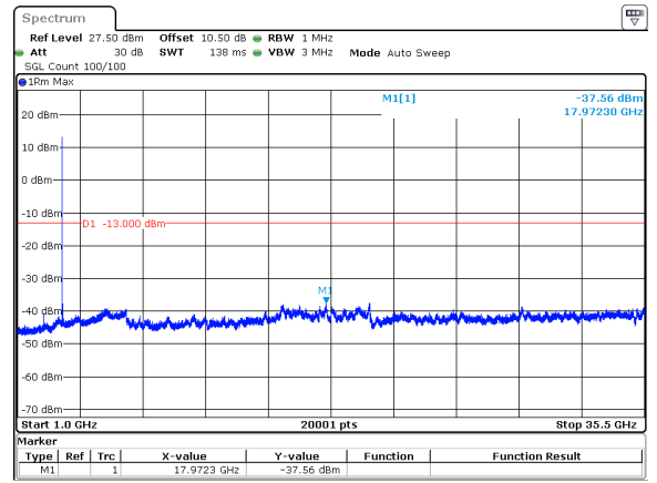
20MHz_15kHz_3460MHz_DFT-s-OFDM QPSK_RB1@0&-37.56 dBm
