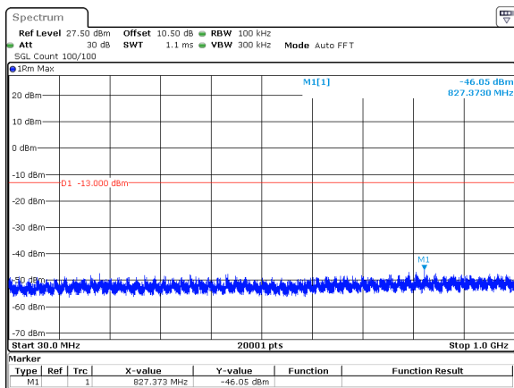
10MHz_30kHz_3500MHz_DFT-s-OFDM QPSK_RB24@0&-46.05 dBm
