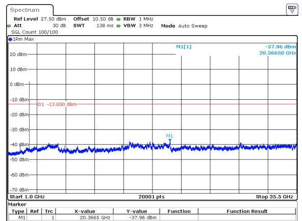
20MHz_30kHz_3540MHz_DFT-s-OFDM QPSK_RB50@0&-37.96 dBm
