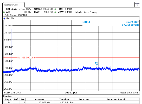
10MHz_15kHz_2535MHz_DFT-s-OFDM QPSK_RB50@0&-36.89 dBm
