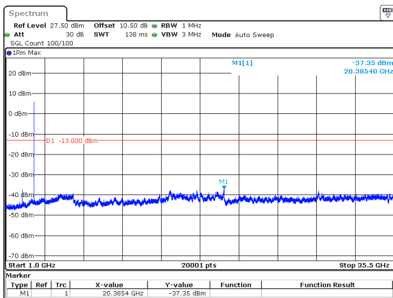
10MHz_15kHz_3500MHz_DFT-s-OFDM QPSK_RB50@0&-37.35 dBm
