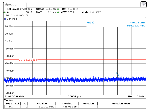
20MHz_15kHz_2560MHz_DFT-s-OFDM QPSK_RB1@105&-46.95 dBm
