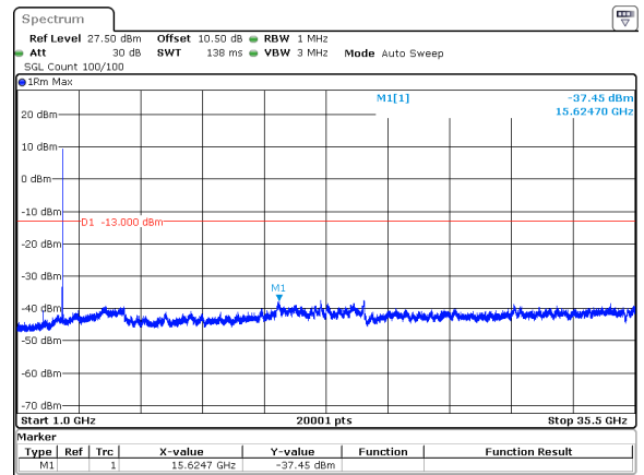
40MHz_15kHz_3530MHz_DFT-s-OFDM QPSK_RB1@215&-37.45 dBm
