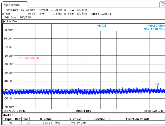
10MHz_15kHz_3500MHz_DFT-s-OFDM QPSK_RB1@0&-46.89 dBm
