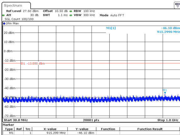
20MHz_30kHz_3500MHz_DFT-s-OFDM QPSK_RB50@0&-46.10 dBm
