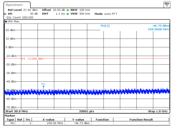
30MHz_15kHz_3465MHz_DFT-s-OFDM QPSK_RB1@0&-46.73 dBm
