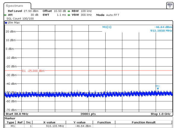
20MHz_15kHz_2560MHz_DFT-s-OFDM QPSK_RB100@0&-46.64 dBm
