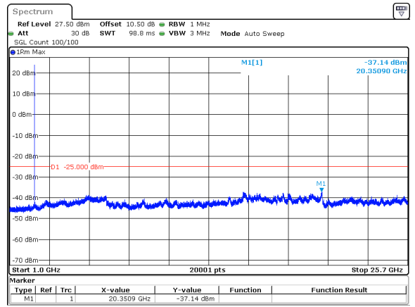
10MHz_15kHz_2535MHz_DFT-s-OFDM QPSK_RB1@0&-37.14 dBm
