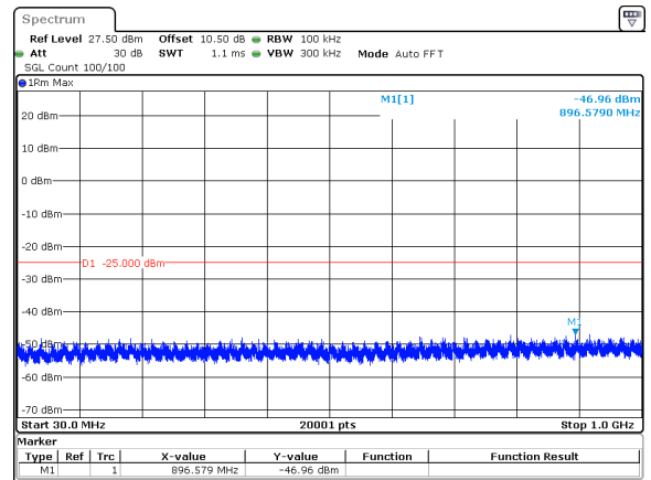
20MHz_15kHz_2510MHz_DFT-s-OFDM QPSK_RB1@105&-46.96 dBm
