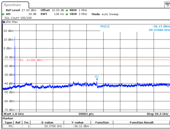
40MHz_15kHz_3530MHz_DFT-s-OFDM QPSK_RB1@0&-36.12 dBm
