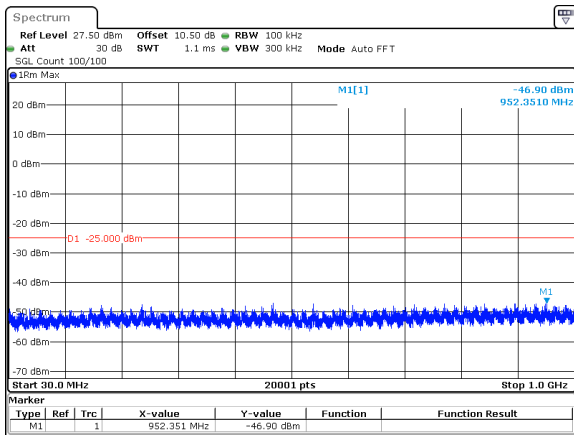
20MHz_15kHz_2535MHz_DFT-s-OFDM QPSK_RB1@105&-46.90 dBm
