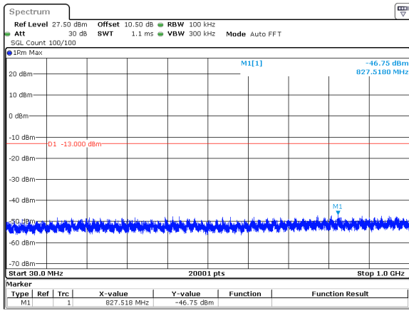
20MHz_30kHz_3540MHz_DFT-s-OFDM QPSK_RB1@0&-46.75 dBm
