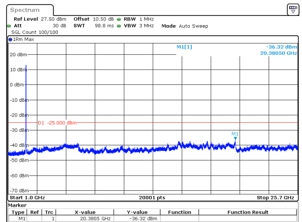
20MHz_15kHz_2510MHz_DFT-s-OFDM QPSK_RB100@0&-36.32 dBm
