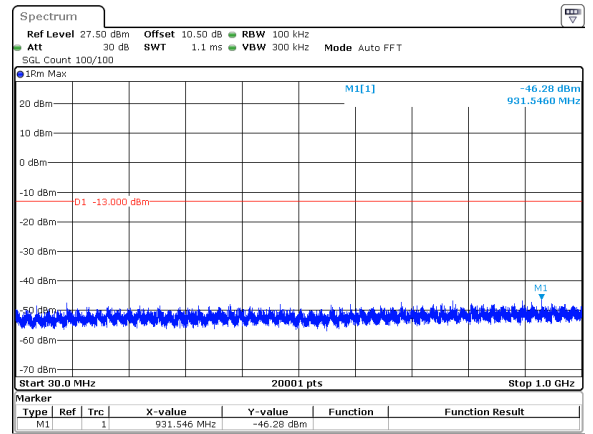
10MHz_30kHz_3500MHz_DFT-s-OFDM QPSK_RB1@0&-46.28 dBm
