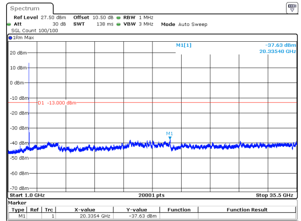
20MHz_15kHz_3500MHz_DFT-s-OFDM QPSK_RB1@0&-37.63 dBm
