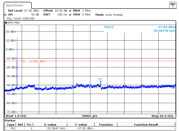
20MHz_15kHz_3460MHz_DFT-s-OFDM QPSK_RB1@105&-37.02 dBm
