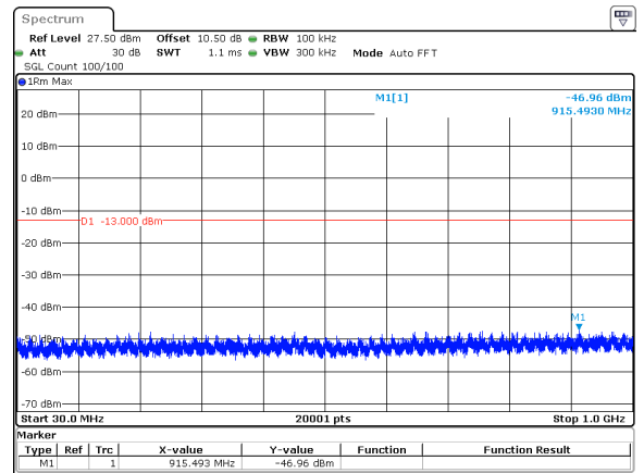
20MHz_30kHz_3540MHz_DFT-s-OFDM QPSK_RB1@50&-46.96 dBm
