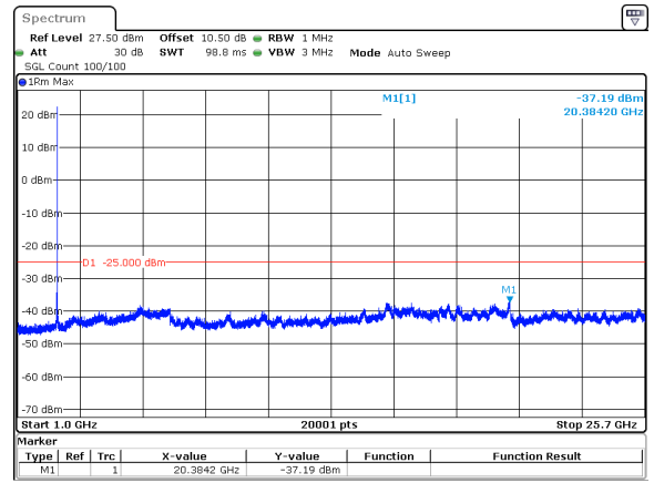
20MHz_15kHz_2560MHz_DFT-s-OFDM QPSK_RB1@0&-37.19 dBm
