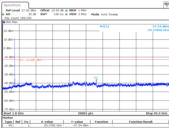
20MHz_15kHz_3500MHz_DFT-s-OFDM QPSK_RB1@105&-37.54 dBm
