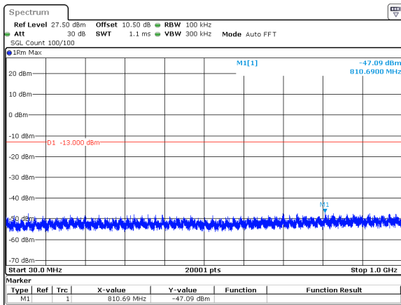
40MHz_15kHz_3530MHz_DFT-s-OFDM QPSK_RB1@215&-47.09 dBm
