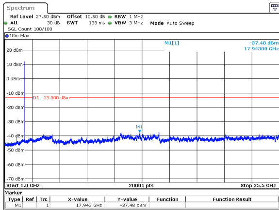
10MHz_30kHz_3500MHz_DFT-s-OFDM QPSK_RB1@0&-37.48 dBm
