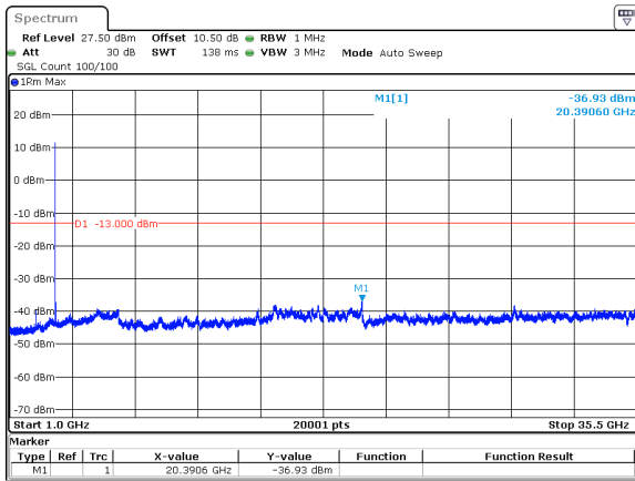
30MHz_15kHz_3500MHz_DFT-s-OFDM QPSK_RB1@0&-36.93 dBm
