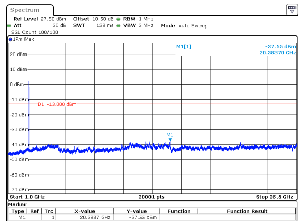
20MHz_30kHz_3460MHz_DFT-s-OFDM QPSK_RB50@0&-37.55 dBm
