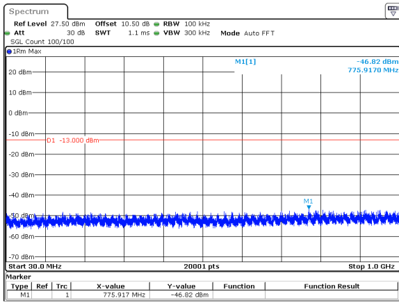
20MHz_15kHz_3460MHz_DFT-s-OFDM QPSK_RB1@0&-46.82 dBm
