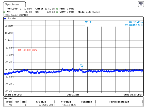
10MHz_30kHz_3455MHz_DFT-s-OFDM QPSK_RB1@23&-37.19 dBm
