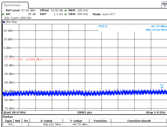
40MHz_15kHz_3500MHz_DFT-s-OFDM QPSK_RB1@215&-46.79 dBm
