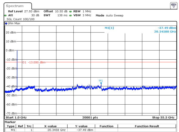
40MHz_15kHz_3470MHz_DFT-s-OFDM QPSK_RB216@0&-37.49 dBm
