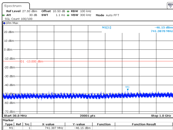
10MHz_15kHz_3545MHz_DFT-s-OFDM QPSK_RB50@0&-46.15 dBm
