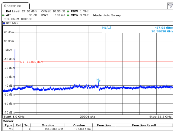
40MHz_30kHz_3470MHz_DFT-s-OFDM QPSK_RB100@0&-37.03 dBm
