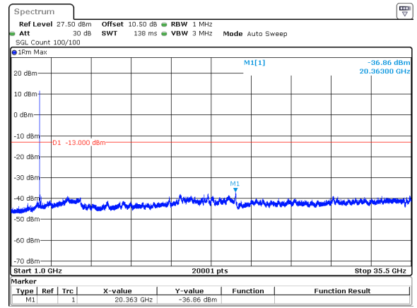
40MHz_30kHz_3470MHz_DFT-s-OFDM QPSK_RB1@0&-36.86 dBm
