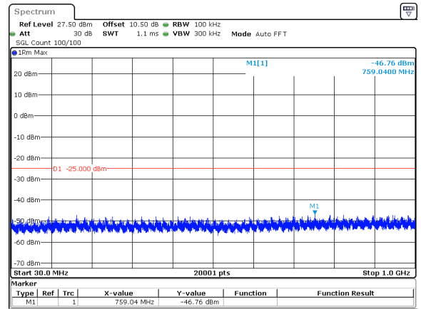
20MHz_15kHz_2535MHz_DFT-s-OFDM QPSK_RB1@0&-46.76 dBm
