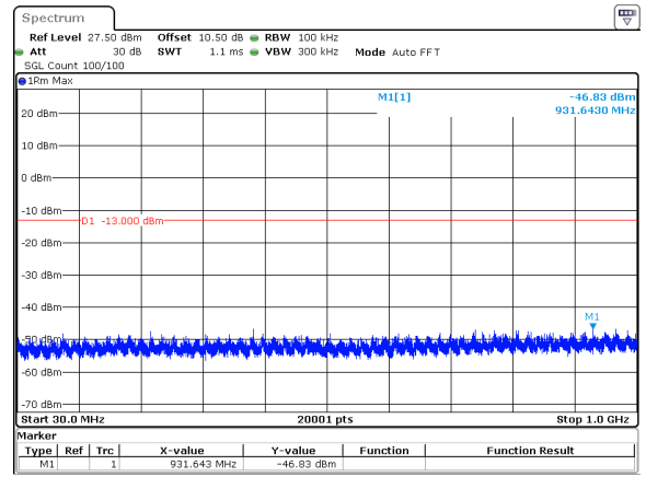
40MHz_30kHz_3530MHz_DFT-s-OFDM QPSK_RB1@0&-46.83 dBm
