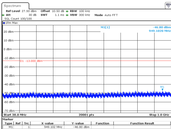
10MHz_30kHz_3455MHz_DFT-s-OFDM QPSK_RB24@0&-46.80 dBm
