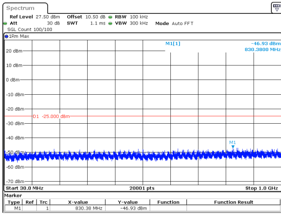
20MHz_15kHz_2510MHz_DFT-s-OFDM QPSK_RB1@0&-46.93 dBm
