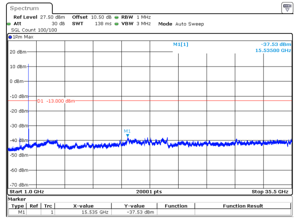
10MHz_15kHz_3500MHz_DFT-s-OFDM QPSK_RB1@0&-37.53 dBm
