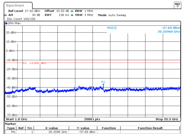
20MHz_30kHz_3500MHz_DFT-s-OFDM QPSK_RB50@0&-37.69 dBm
