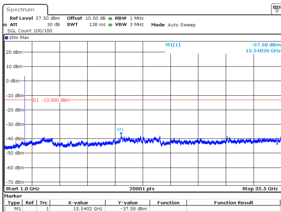
20MHz_15kHz_3540MHz_DFT-s-OFDM QPSK_RB100@0&-37.58 dBm
