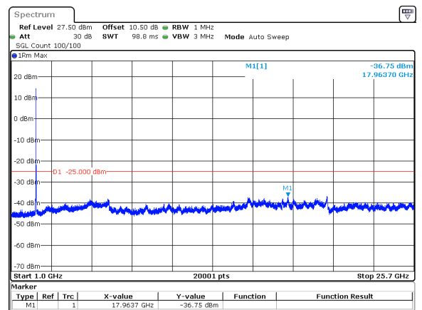
15MHz_15kHz_2507.5MHz_DFT-s-OFDM QPSK_RB75@0&-36.75 dBm
