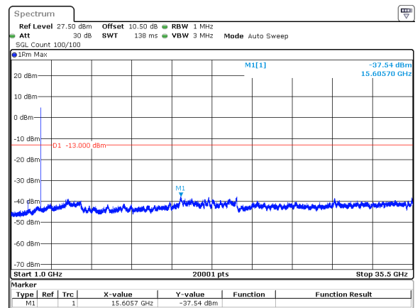
10MHz_15kHz_3545MHz_DFT-s-OFDM QPSK_RB50@0&-37.54 dBm
