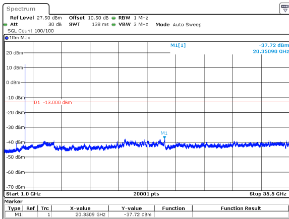
20MHz_30kHz_3500MHz_DFT-s-OFDM QPSK_RB1@50&-37.72 dBm
