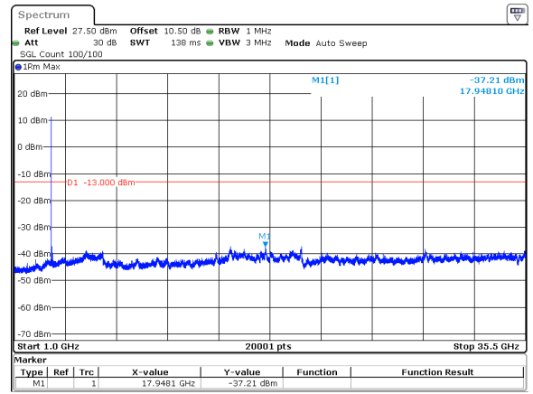
40MHz_30kHz_3500MHz_DFT-s-OFDM QPSK_RB1@0&-37.21 dBm
