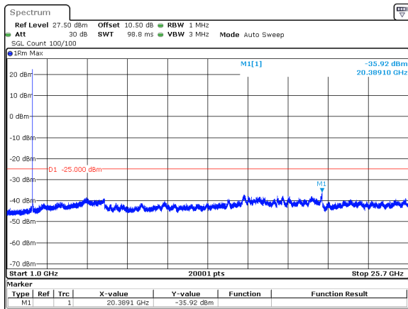
10MHz_15kHz_2565MHz_DFT-s-OFDM QPSK_RB1@51&-35.92 dBm
