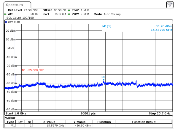
20MHz_15kHz_2510MHz_DFT-s-OFDM QPSK_RB1@0&-36.90 dBm
