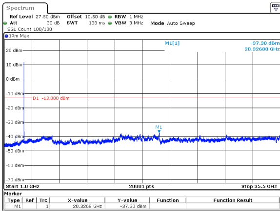
30MHz_15kHz_3465MHz_DFT-s-OFDM QPSK_RB1@0&-37.30 dBm
