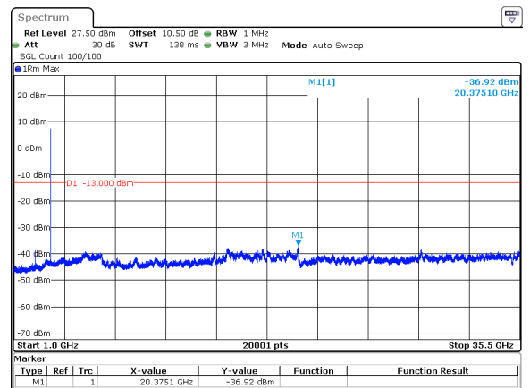
10MHz_30kHz_3500MHz_DFT-s-OFDM QPSK_RB24@0&-36.92 dBm
