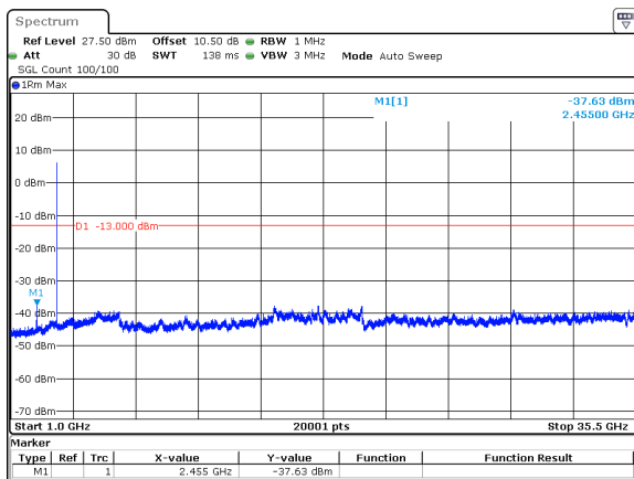
10MHz_30kHz_3545MHz_DFT-s-OFDM QPSK_RB24@0&-37.63 dBm
