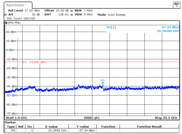
30MHz_15kHz_3535MHz_DFT-s-OFDM QPSK_RB1@0&-37.34 dBm
