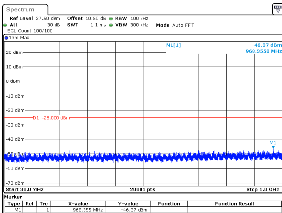
20MHz_15kHz_2510MHz_DFT-s-OFDM QPSK_RB100@0&-46.37 dBm
