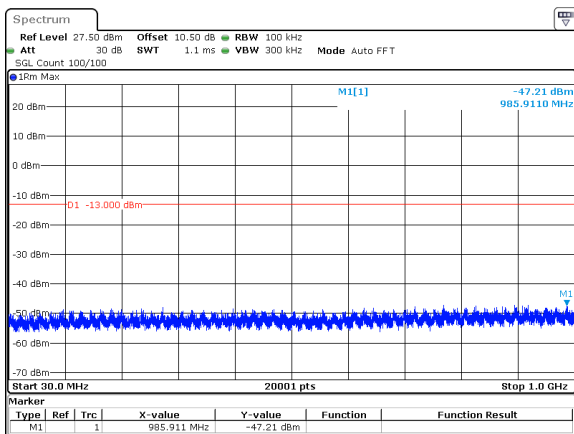
20MHz_30kHz_3540MHz_DFT-s-OFDM QPSK_RB50@0&-47.21 dBm
