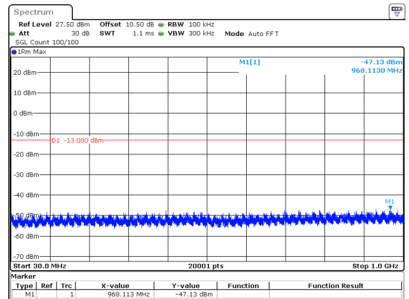
20MHz_15kHz_3500MHz_DFT-s-OFDM QPSK_RB100@0&-47.13 dBm
