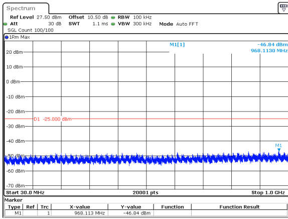
20MHz_15kHz_2560MHz_DFT-s-OFDM QPSK_RB1@0&-46.84 dBm
