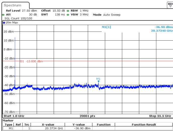
40MHz_15kHz_3470MHz_DFT-s-OFDM QPSK_RB1@215&-36.90 dBm
