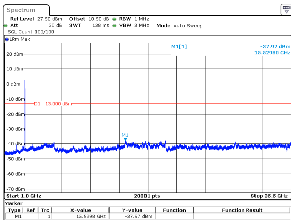
20MHz_15kHz_3460MHz_DFT-s-OFDM QPSK_RB100@0&-37.97 dBm
