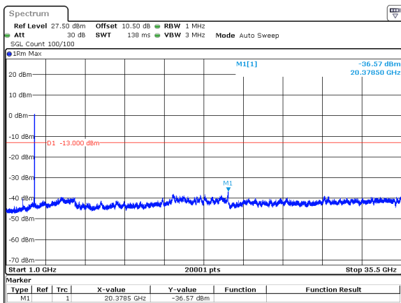
30MHz_15kHz_3465MHz_DFT-s-OFDM QPSK_RB160@0&-36.57 dBm
