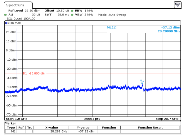
10MHz_15kHz_2565MHz_DFT-s-OFDM QPSK_RB1@0&-37.12 dBm
