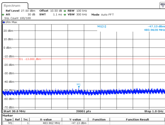
20MHz_30kHz_3460MHz_DFT-s-OFDM QPSK_RB50@0&-47.13 dBm
