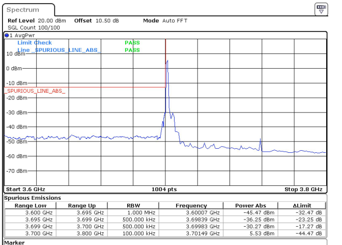
60MHz_30kHz_3730MHz_DFT-s-OFDM QPSK_RB1@0 -30.27 dBm
