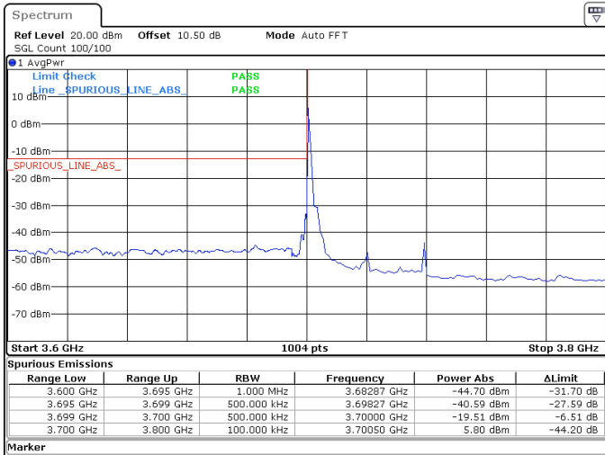
40MHz_15kHz_3720MHz_DFT-s-OFDM QPSK_RB1@0 -19.51 dBm
