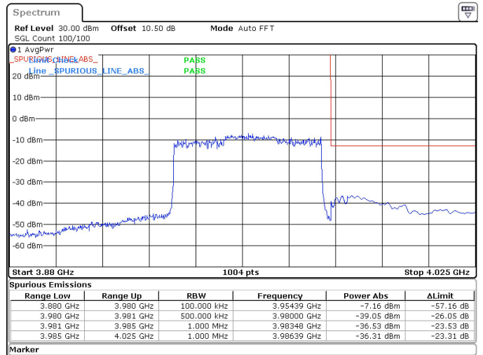
50MHz_30kHz_3955MHz_DFT-s-OFDM QPSK_RB128@0 -36.31 dBm
