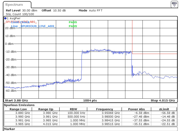
40MHz_15kHz_3960MHz_DFT-s-OFDM QPSK_RB216@0 -27.48 dBm
