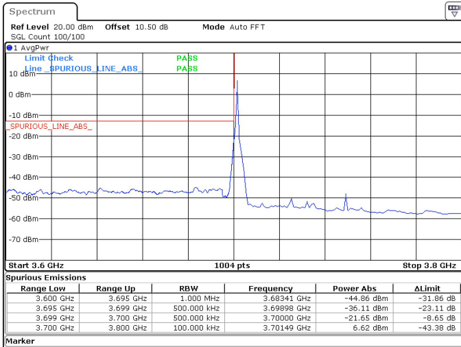
50MHz_30kHz_3725MHz_DFT-s-OFDM QPSK_RB1@0 -21.65 dBm
