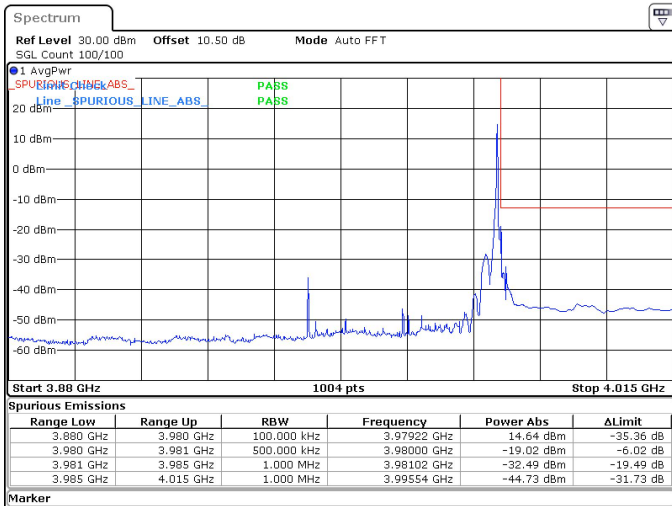
40MHz_15kHz_3960MHz_DFT-s-OFDM QPSK_RB1@215 -19.02 dBm
