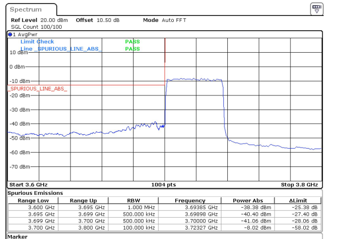
40MHz_30kHz_3720MHz_DFT-s-OFDM QPSK_RB100@0 -38.38 dBm
