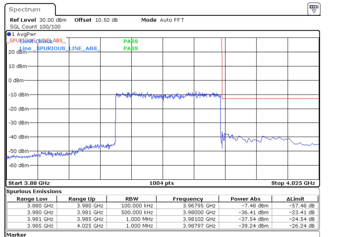
50MHz_15kHz_3955MHz_DFT-s-OFDM QPSK_RB270@0 -36.41 dBm
