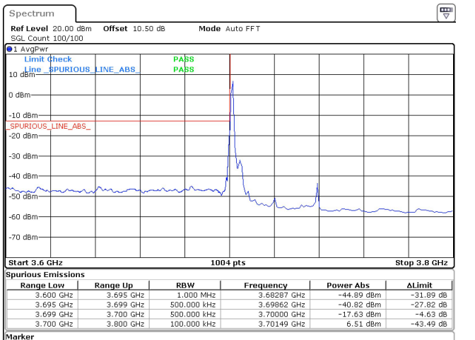
40MHz_30kHz_3720MHz_DFT-s-OFDM QPSK_RB1@0 -17.63 dBm
