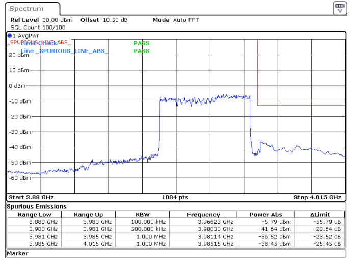
40MHz_30kHz_3960MHz_DFT-s-OFDM QPSK_RB100@0 -36.52 dBm
