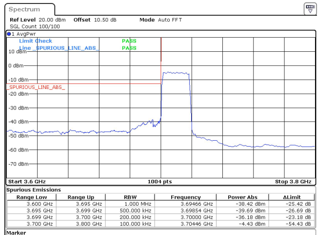
20MHz_30kHz_3710MHz_DFT-s-OFDM QPSK_RB50@0 -36.18 dBm
