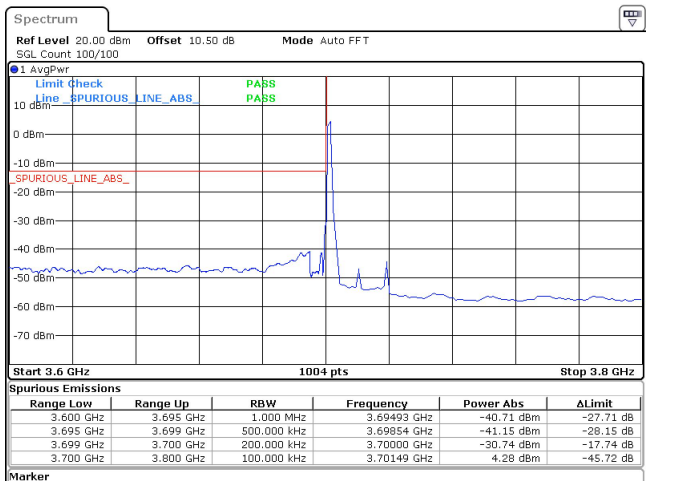
20MHz_30kHz_3710MHz_DFT-s-OFDM QPSK_RB1@0 -30.74 dBm
