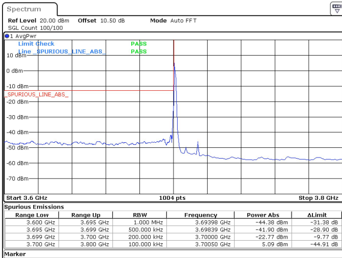
15MHz_30kHz_3707.5MHz_DFT-s-OFDM QPSK_RB1@0 -22.77 dBm
