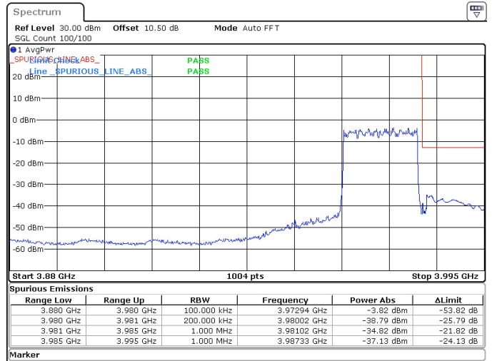
20MHz_30kHz_3970MHz_DFT-s-OFDM QPSK_RB50@0 -34.82 dBm
