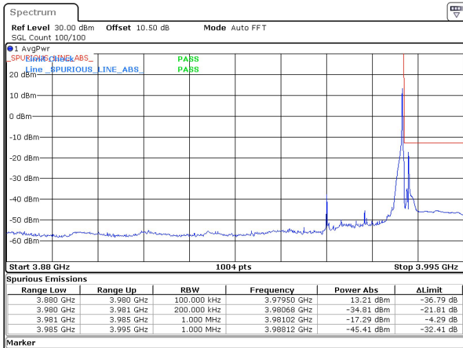
20MHz_15kHz_3970MHz_DFT-s-OFDM QPSK_RB1@105 -17.29 dBm
