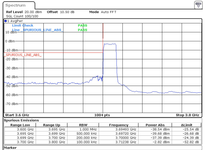
15MHz_30kHz_3707.5MHz_DFT-s-OFDM QPSK_RB36@0 -37.39 dBm
