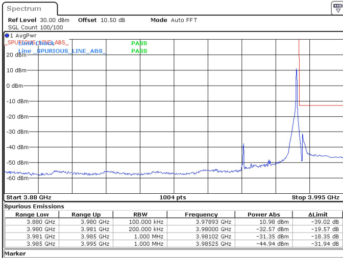
20MHz_30kHz_3970MHz_DFT-s-OFDM QPSK_RB1@50 -31.35 dBm
