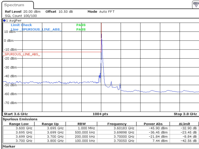
20MHz_15kHz_3710MHz_DFT-s-OFDM QPSK_RB1@0 -21.84 dBm
