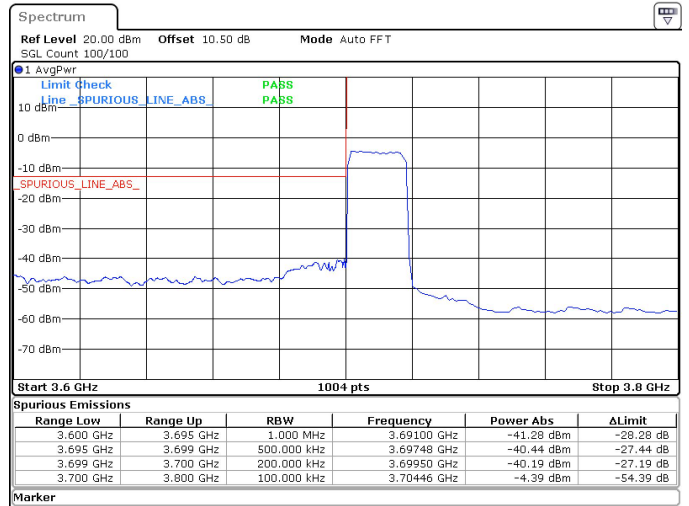
20MHz_15kHz_3710MHz_DFT-s-OFDM QPSK_RB100@0 -40.19 dBm
