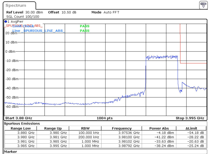
20MHz_15kHz_3970MHz_DFT-s-OFDM QPSK_RB100@0 -33.63 dBm
