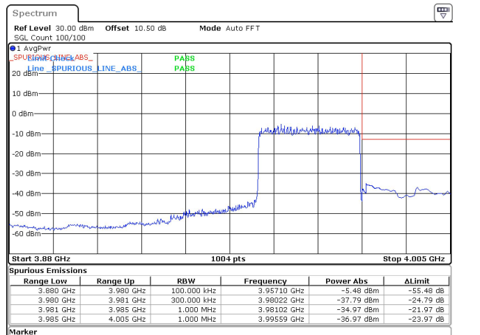
30MHz_15kHz_3965MHz_DFT-s-OFDM QPSK_RB160@0 -34.97 dBm
