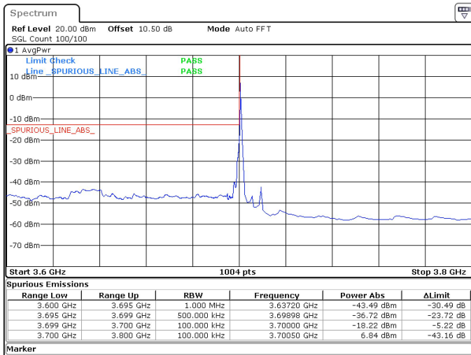
10MHz_15kHz_3705MHz_DFT-s-OFDM QPSK_RB1@0 -18.22 dBm
