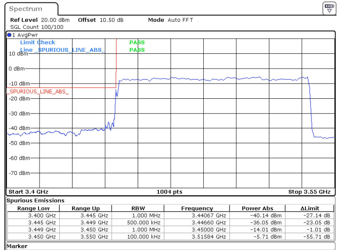
90MHz_30kHz_3495MHz_DFT-s-OFDM QPSK_RB243@0 -14.01 dBm
