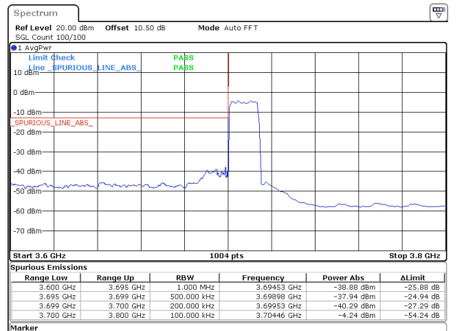
15MHz_15kHz_3707.5MHz_DFT-s-OFDM QPSK_RB75@0 -37.94 dBm
