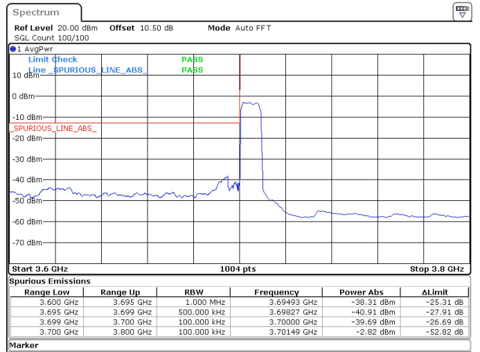
10MHz_15kHz_3705MHz_DFT-s-OFDM QPSK_RB50@0 -38.31 dBm
