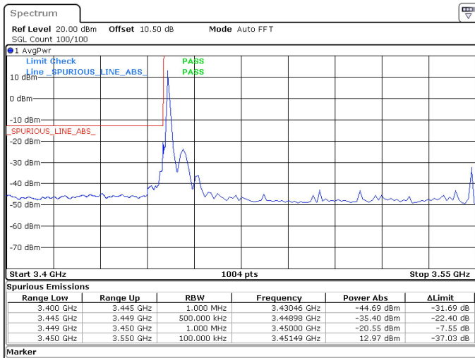
100MHz_30kHz_3500MHz_DFT-s-OFDM QPSK_RB1@0 -20.55 dBm
