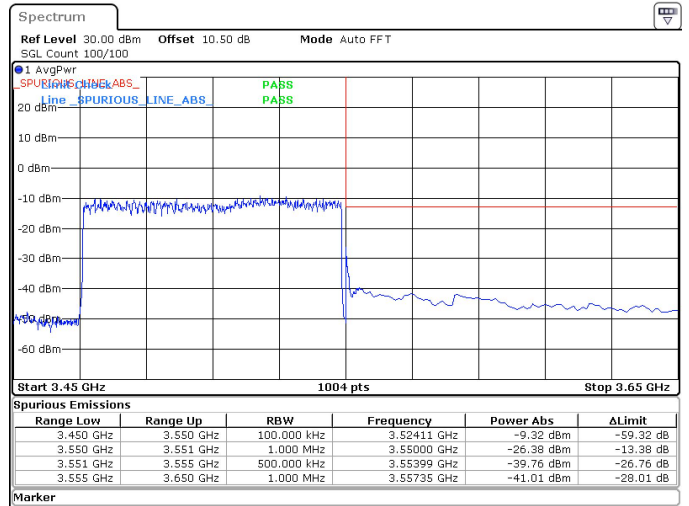
80MHz_30kHz_3510MHz_DFT-s-OFDM QPSK_RB216@0 -26.38 dBm
