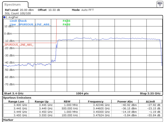
100MHz_30kHz_3500MHz_DFT-s-OFDM QPSK_RB270@0 -14.19 dBm
