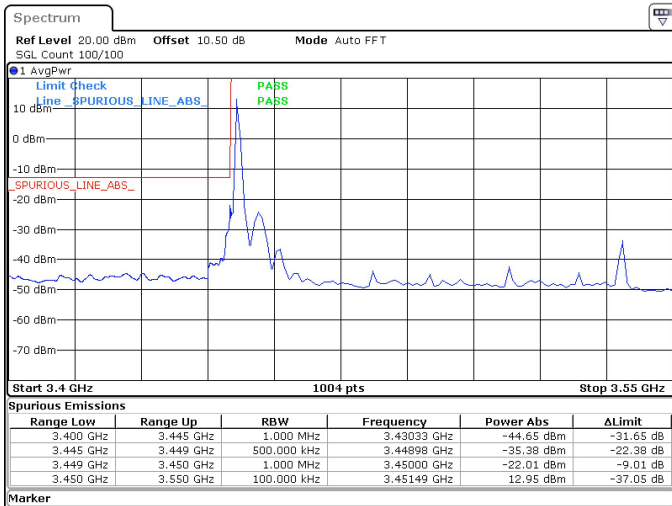
90MHz_30kHz_3495MHz_DFT-s-OFDM QPSK_RB1@0 -22.01 dBm
