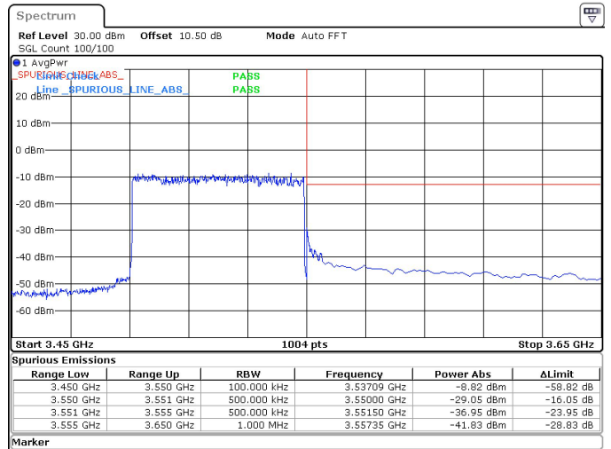
60MHz_30kHz_3520MHz_DFT-s-OFDM QPSK_RB162@0 -29.05 dBm
