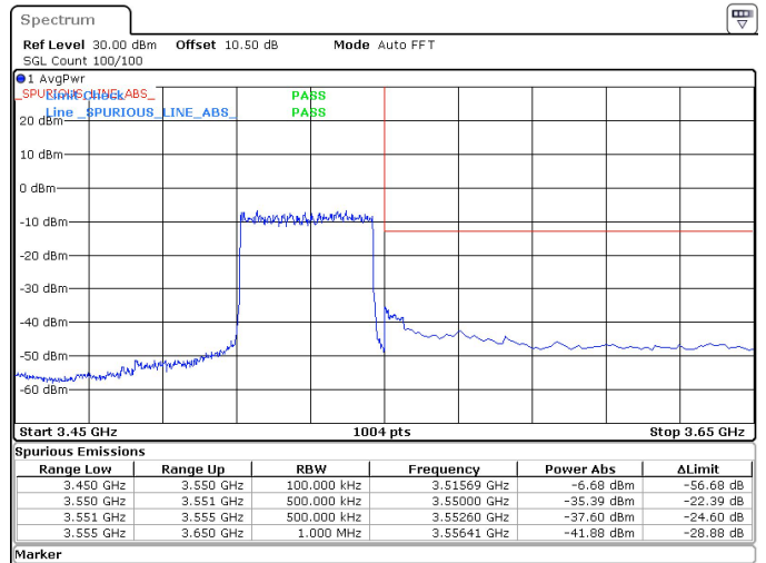
40MHz_30kHz_3530MHz_DFT-s-OFDM QPSK_RB100@0 -35.39 dBm
