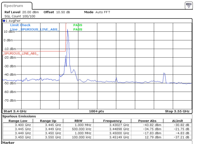
80MHz_30kHz_3490MHz_DFT-s-OFDM QPSK_RB1@0 -17.83 dBm
