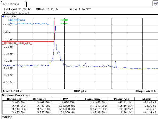
60MHz_30kHz_3480MHz_DFT-s-OFDM QPSK_RB1@0 -18.78 dBm
