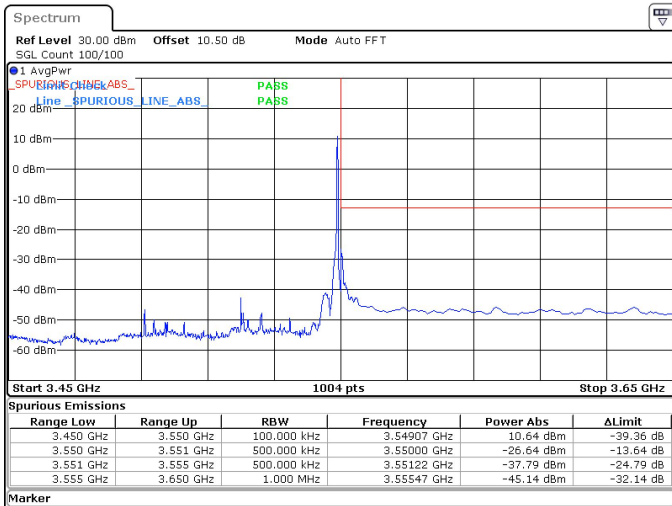
60MHz_30kHz_3520MHz_DFT-s-OFDM QPSK_RB1@161 -26.64 dBm
