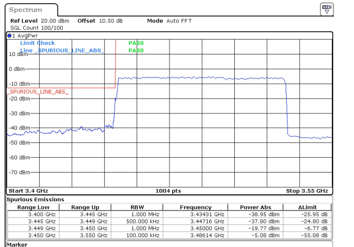
80MHz_30kHz_3490MHz_DFT-s-OFDM QPSK_RB216@0 -19.77 dBm
