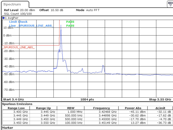
40MHz_30kHz_3470MHz_DFT-s-OFDM QPSK_RB1@0 -17.70 dBm
