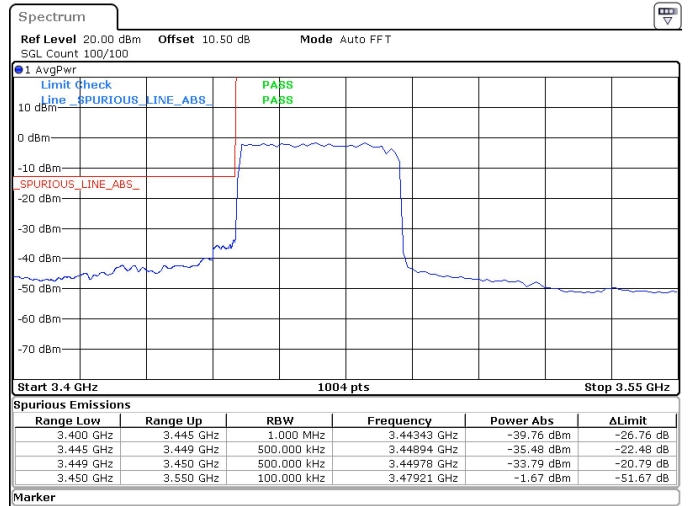
40MHz_30kHz_3470MHz_DFT-s-OFDM QPSK_RB100@0 -33.79 dBm
