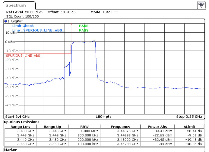
20MHz_15kHz_3460MHz_DFT-s-OFDM QPSK_RB100@0 -22.65 dBm
