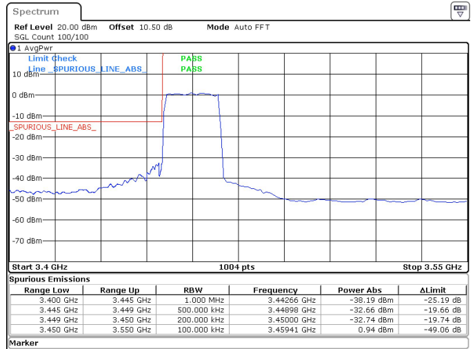
20MHz_30kHz_3460MHz_DFT-s-OFDM QPSK_RB50@0 -32.66 dBm
