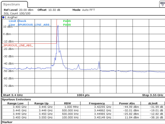
40MHz_15kHz_3470MHz_DFT-s-OFDM QPSK_RB1@0 -25.82 dBm
