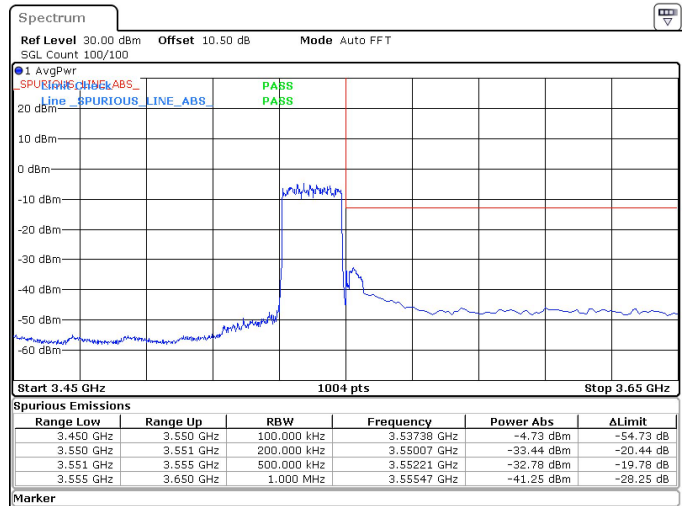
20MHz_30kHz_3540MHz_DFT-s-OFDM QPSK_RB50@0 -32.78 dBm
