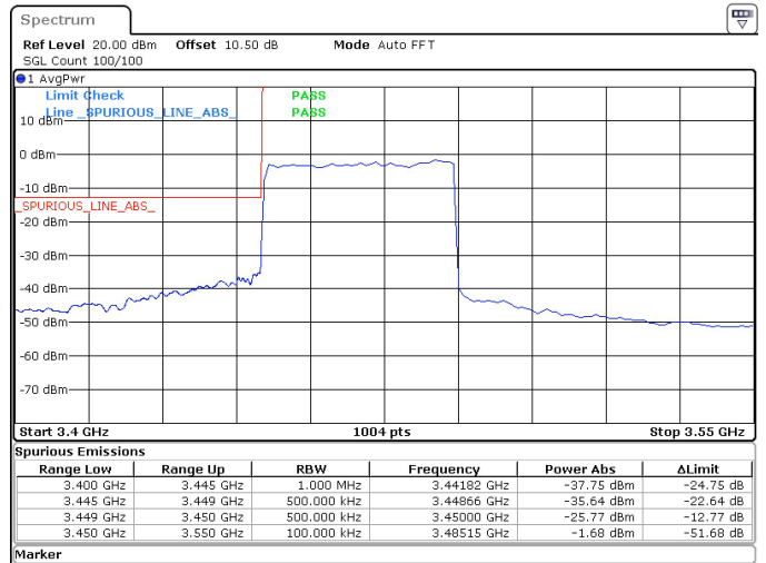
40MHz_15kHz_3470MHz_DFT-s-OFDM QPSK_RB216@0 -25.77 dBm
