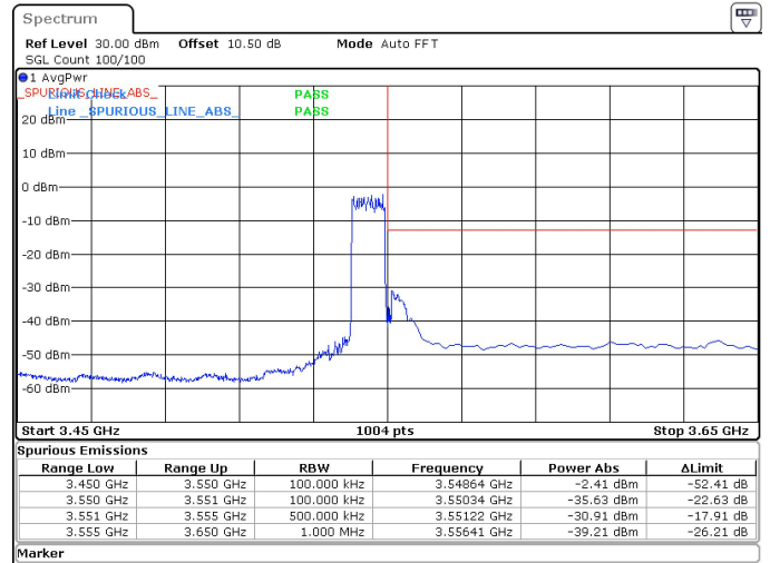
10MHz_15kHz_3545MHz_DFT-s-OFDM QPSK_RB50@0 -30.91 dBm
