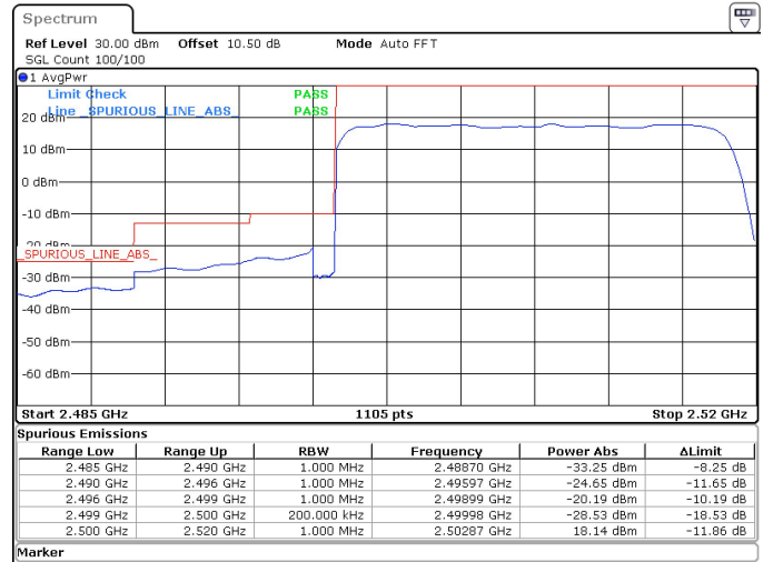
20MHz_15kHz_2510MHz_DFT-s-OFDM QPSK_RB100@0 -33.25 dBm
