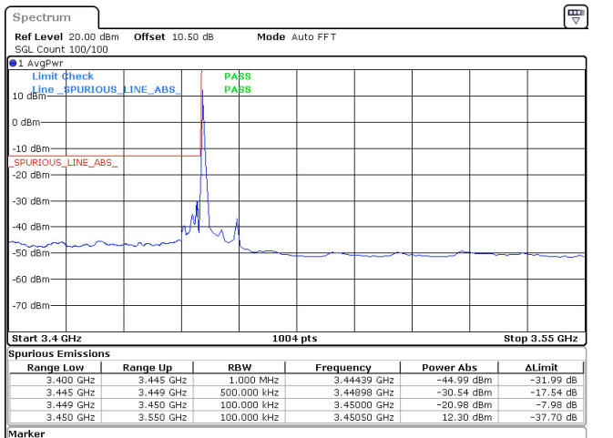
10MHz_15kHz_3455MHz_DFT-s-OFDM QPSK_RB1@0 -20.98 dBm
