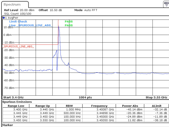
10MHz_30kHz_3455MHz_DFT-s-OFDM QPSK_RB1@0 -20.36 dBm
