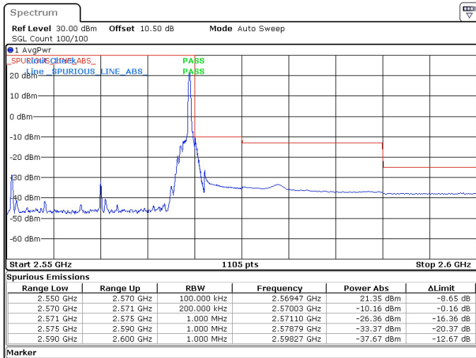
20MHz_15kHz_2560MHz_DFT-s-OFDM QPSK_RB1@105 -10.16 dBm
