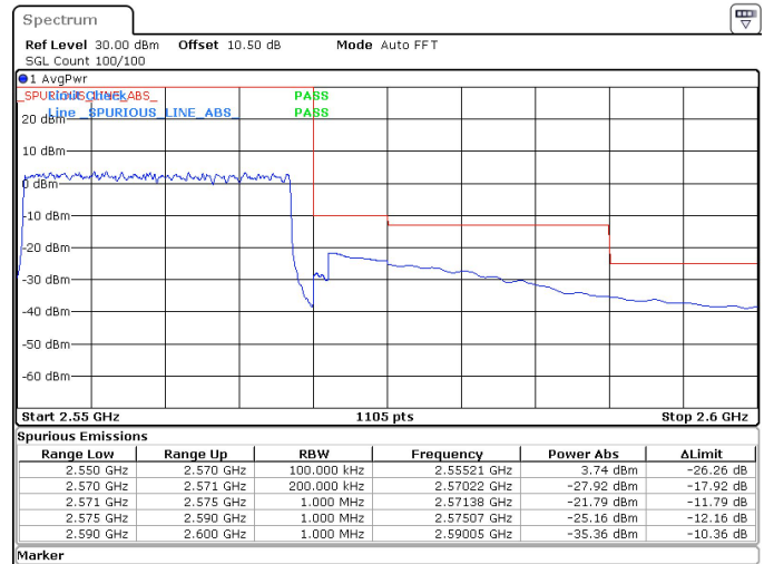
20MHz_15kHz_2560MHz_DFT-s-OFDM QPSK_RB100@0 -35.36 dBm
