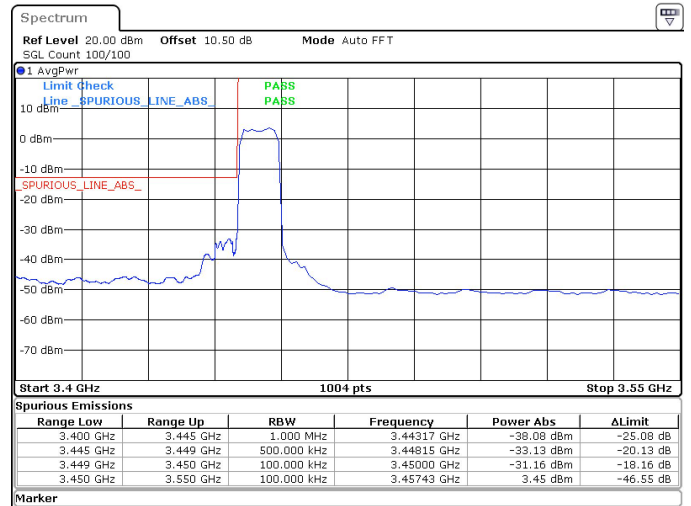
10MHz_30kHz_3455MHz_DFT-s-OFDM QPSK_RB24@0 -31.16 dBm
