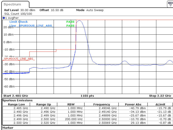
20MHz_15kHz_2510MHz_DFT-s-OFDM QPSK_RB1@0 -10.70 dBm
