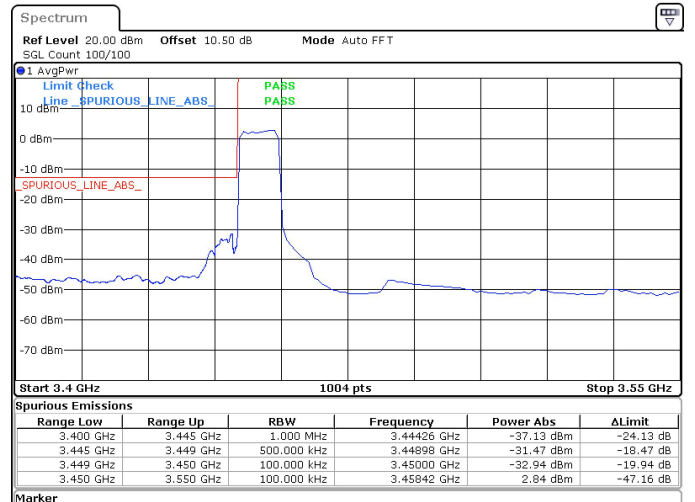
10MHz_15kHz_3455MHz_DFT-s-OFDM QPSK_RB50@0 -31.47 dBm
