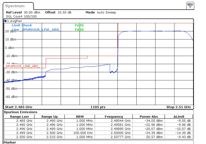
10MHz_15kHz_2505MHz_DFT-s-OFDM QPSK_RB50@0 -34.05 dBm
