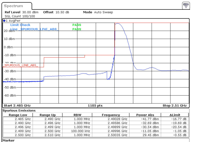
10MHz_15kHz_2505MHz_DFT-s-OFDM QPSK_RB1@0 29.45 dBm
