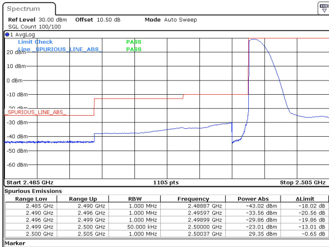
5MHz_15kHz_2502.5MHz_DFT-s-OFDM QPSK_RB1@0 29.35 dBm
