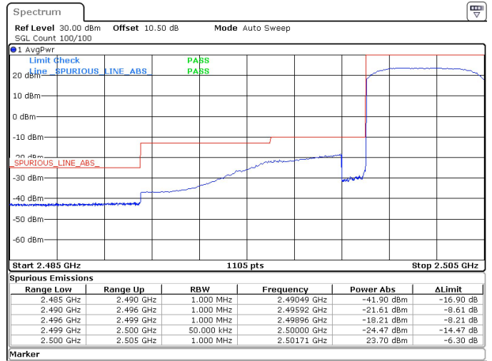
5MHz_15kHz_2502.5MHz_DFT-s-OFDM QPSK_RB25@0 23.70 dBm
