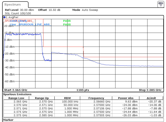
5MHz_15kHz_2567.5MHz_DFT-s-OFDM QPSK_RB25@0 -26.03 dBm
