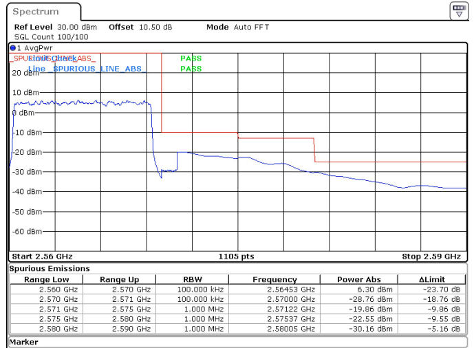
10MHz_15kHz_2565MHz_DFT-s-OFDM QPSK_RB50@0 -30.16 dBm
