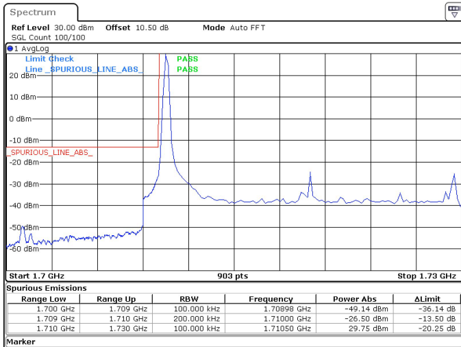
20MHz_15kHz_1720MHz_DFT-s-OFDM QPSK_RB1@0 -26.50 dBm
