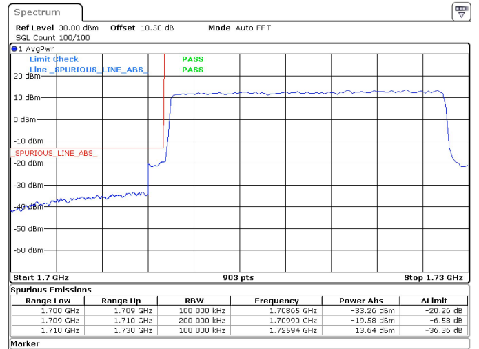
20MHz_15kHz_1720MHz_DFT-s-OFDM QPSK_RB100@0 -19.58 dBm
