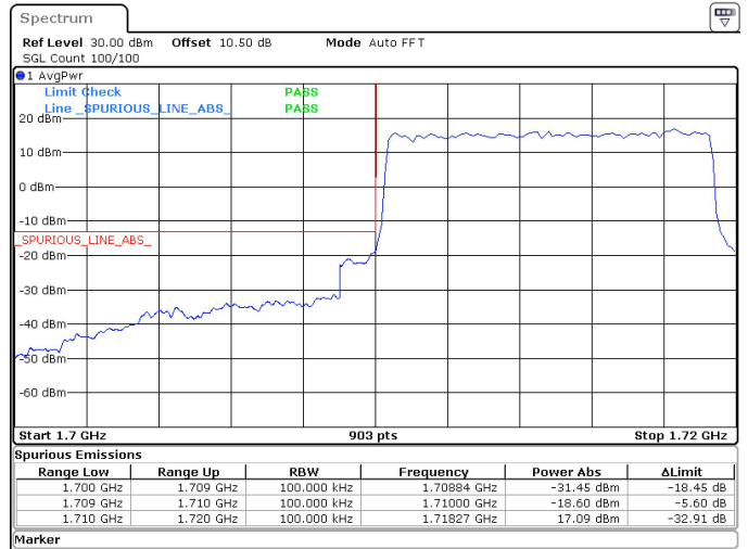
10MHz_15kHz_1715MHz_DFT-s-OFDM QPSK_RB50@0 -18.60 dBm
