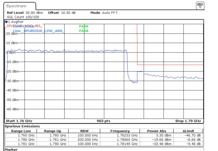
20MHz_15kHz_1770MHz_DFT-s-OFDM QPSK_RB100@0 -19.66 dBm
