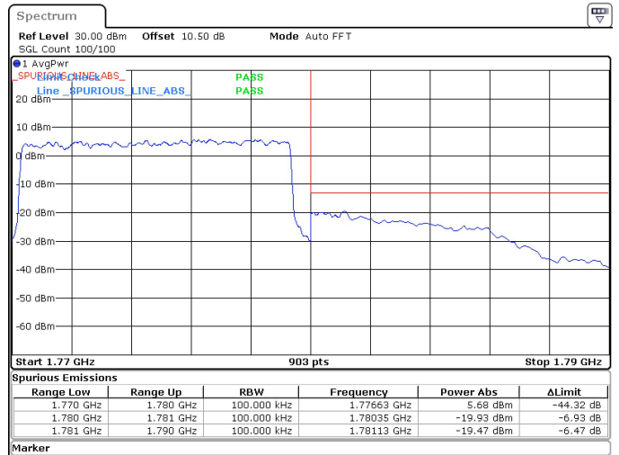
10MHz_15kHz_1775MHz_DFT-s-OFDM QPSK_RB50@0 -19.47 dBm
