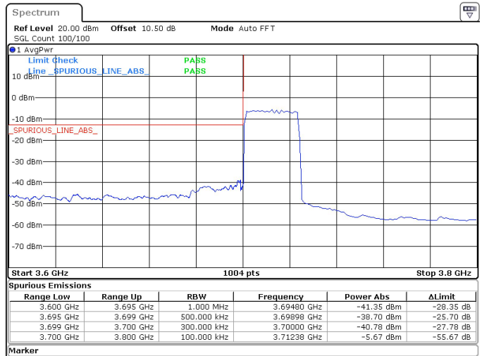
25MHz_30kHz_3712.5MHz_DFT-s-OFDM QPSK_RB64@0 -38.70 dBm
