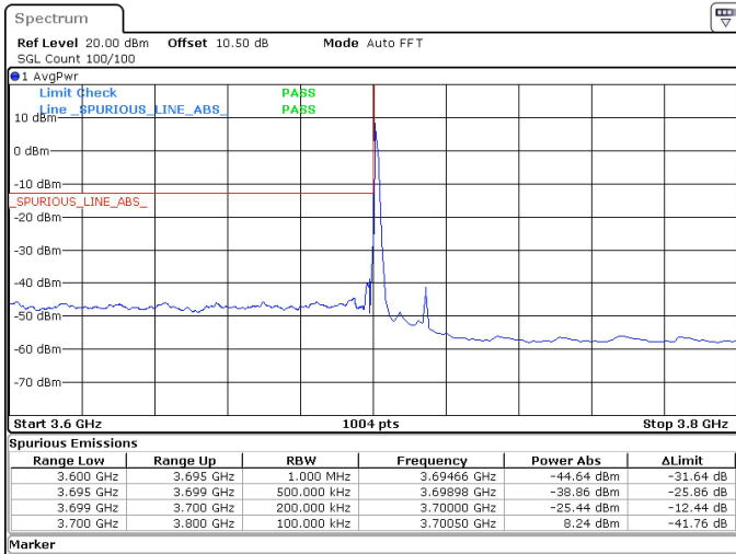
15MHz_30kHz_3707.5MHz_DFT-s-OFDM QPSK_RB1@0 -25.44 dBm
