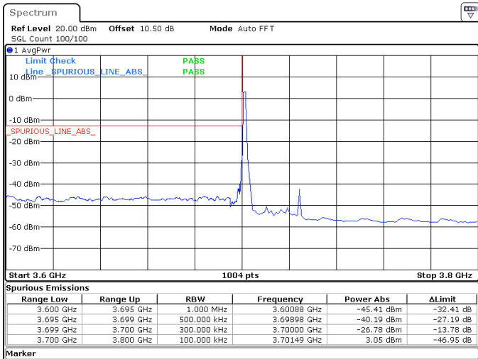
25MHz_30kHz_3712.5MHz_DFT-s-OFDM QPSK_RB1@0 -26.78 dBm
