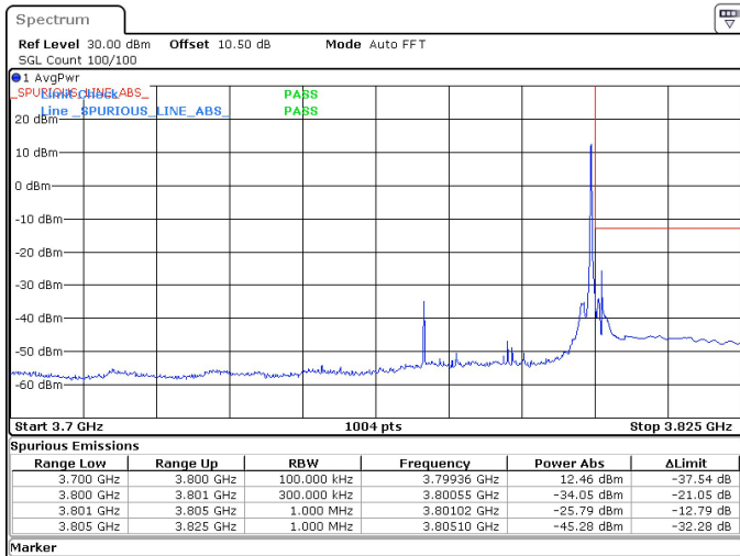
30MHz_15kHz_3785MHz_DFT-s-OFDM QPSK_RB1@159 -25.79 dBm
