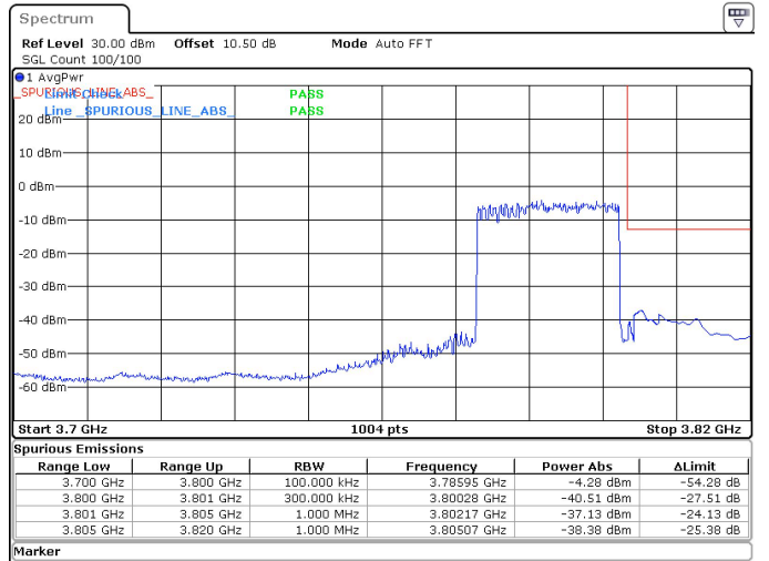
25MHz_15kHz_3787.5MHz_DFT-s-OFDM QPSK_RB128@0 -37.13 dBm
