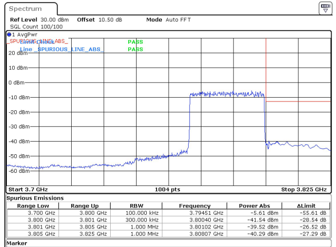
30MHz_15kHz_3785MHz_DFT-s-OFDM QPSK_RB160@0 -39.52 dBm
