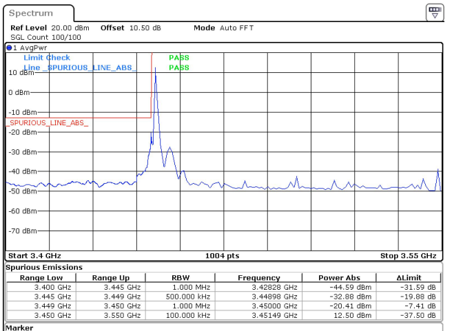
100MHz_30kHz_3500MHz_DFT-s-OFDM QPSK_RB1@0 -20.41 dBm
