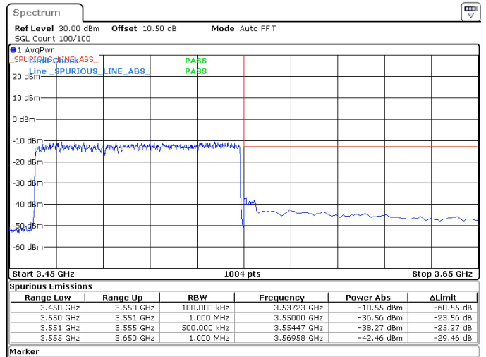
90MHz_30kHz_3505MHz_DFT-s-OFDM QPSK_RB243@0 -36.56 dBm
