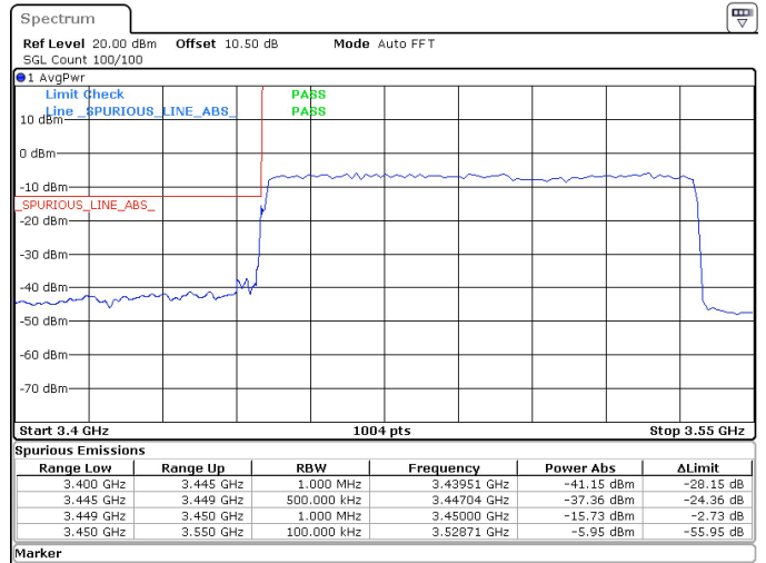
90MHz_30kHz_3495MHz_DFT-s-OFDM QPSK_RB243@0 -15.73 dBm
