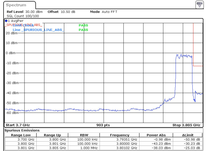
10MHz_30kHz_3795MHz_DFT-s-OFDM QPSK_RB24@0 -38.03 dBm
