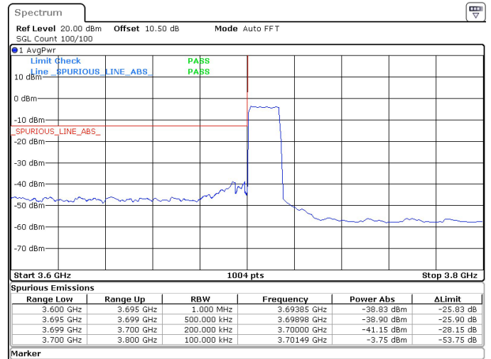
15MHz_15kHz_3707.5MHz_DFT-s-OFDM QPSK_RB75@0 -38.83 dBm
