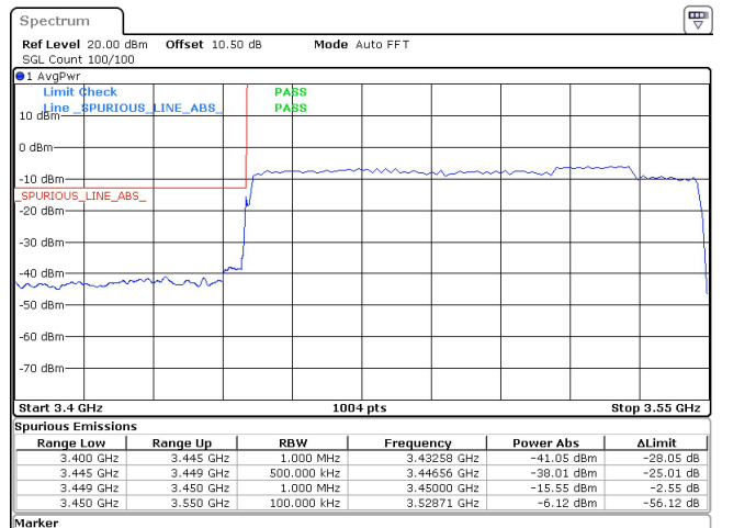
100MHz_30kHz_3500MHz_DFT-s-OFDM QPSK_RB270@0 -15.55 dBm
