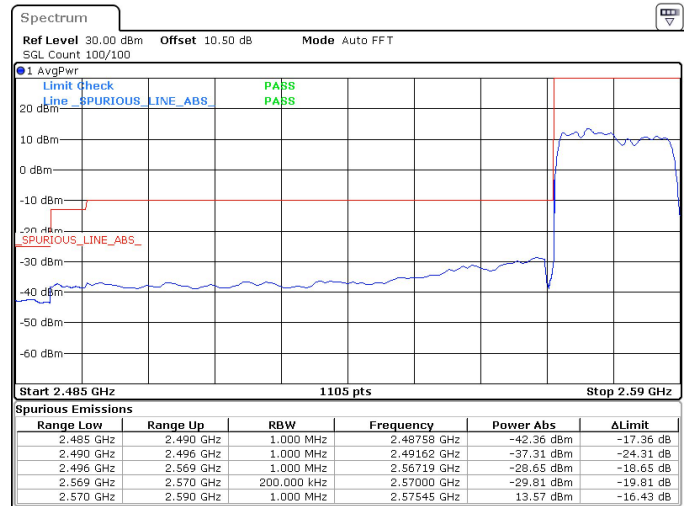
20MHz_30kHz_2580MHz_DFT-s-OFDM QPSK_RB50@0 13.57 dBm
