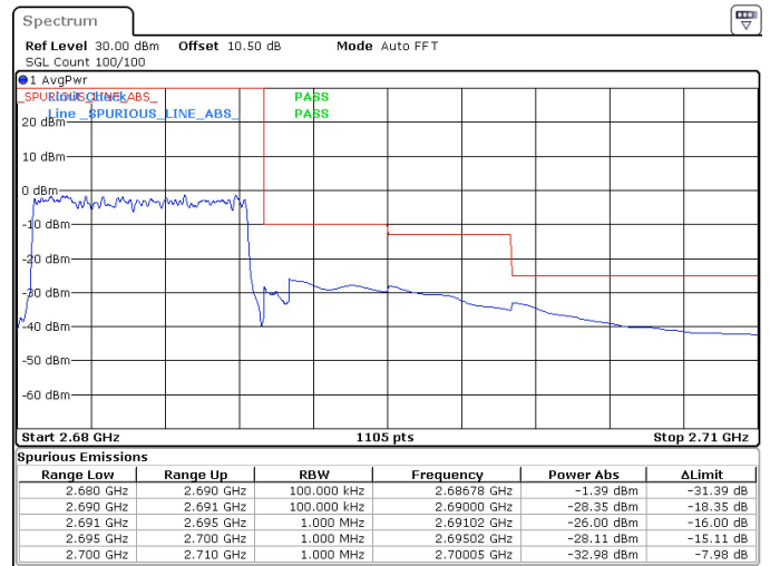
10MHz_30kHz_2685MHz_DFT-s-OFDM QPSK_RB24@0 -32.98 dBm
