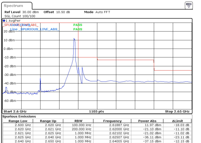
20MHz_30kHz_2610MHz_DFT-s-OFDM QPSK_RB1@50 -21.02 dBm
