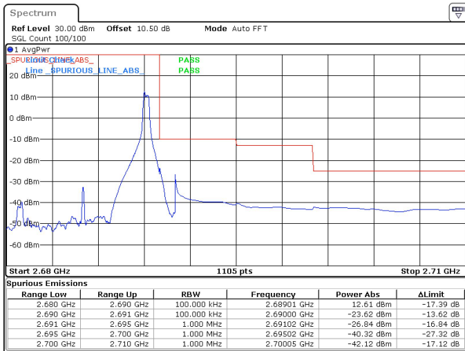
10MHz_30kHz_2685MHz_DFT-s-OFDM QPSK_RB1@23 -23.62 dBm
