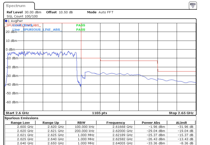
20MHz_30kHz_2610MHz_DFT-s-OFDM QPSK_RB50@0 -33.36 dBm
