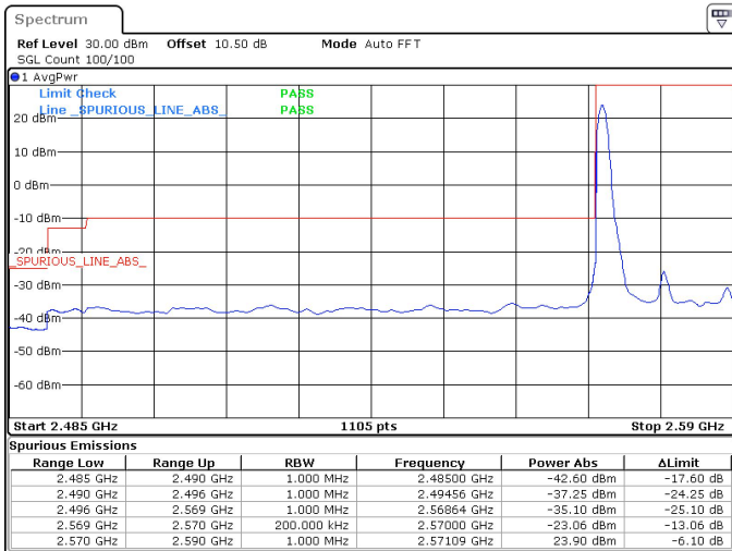
20MHz_30kHz_2580MHz_DFT-s-OFDM QPSK_RB1@0 23.90 dBm
