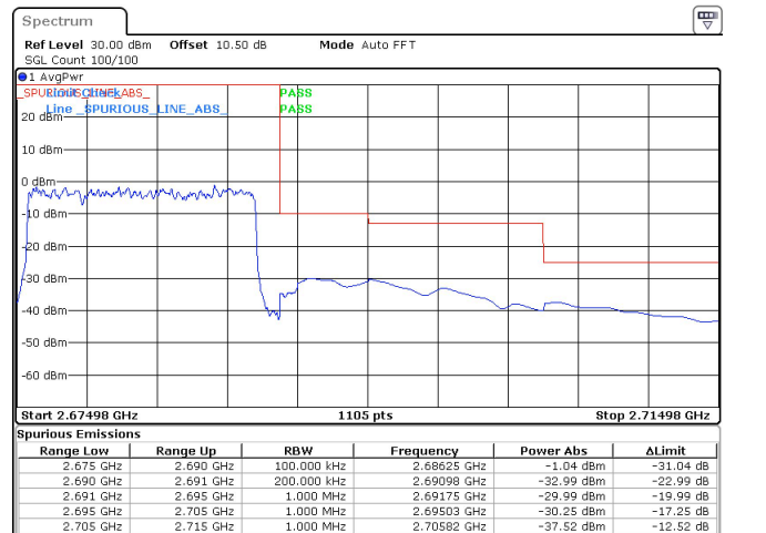
15MHz_30kHz_2682.48MHz_DFT-s-OFDM QPSK_RB36@0 -37.52 dBm
