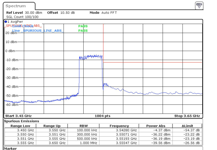
25MHz_30kHz_3537.5MHz_DFT-s-OFDM QPSK_RB64@0 -36.19 dBm
