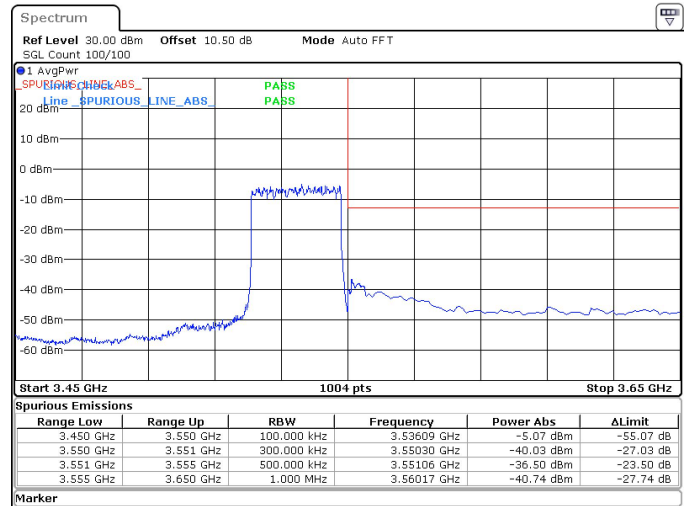
30MHz_30kHz_3535MHz_DFT-s-OFDM QPSK_RB75@0 -36.50 dBm
