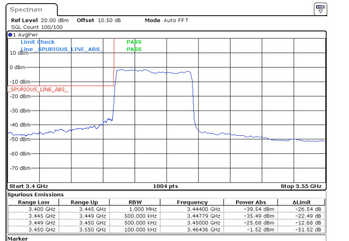
40MHz_30kHz_3470MHz_DFT-s-OFDM QPSK_RB100@0 -25.68 dBm
