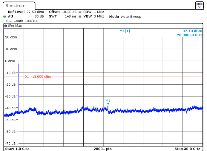
25MHz_15kHz_3750MHz_DFT-s-OFDM QPSK_RB128@0 -37.13 dBm
