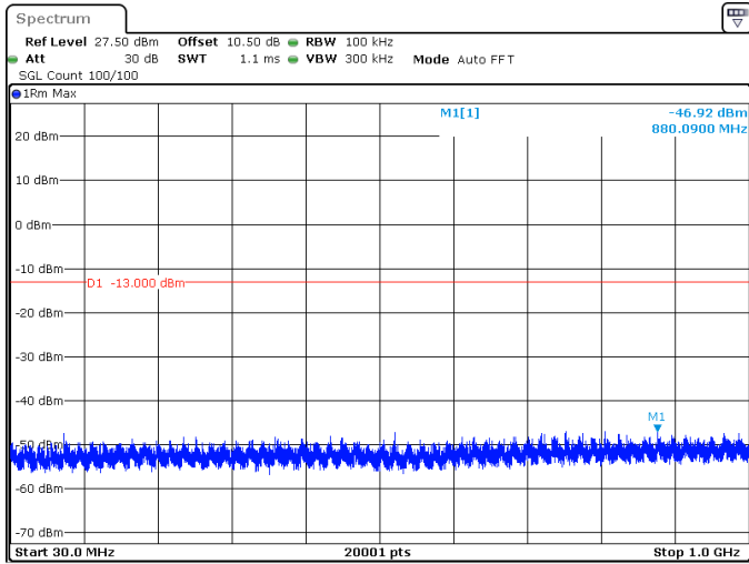
30MHz_30kHz_3715MHz_DFT-s-OFDM QPSK_RB1@0 -46.92 dBm
