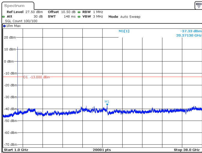
80MHz_30kHz_3740MHz_DFT-s-OFDM QPSK_RB1@0 -37.33 dBm
