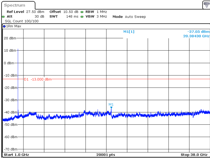
40MHz_30kHz_3750MHz_DFT-s-OFDM QPSK_RB1@0 -37.05 dBm
