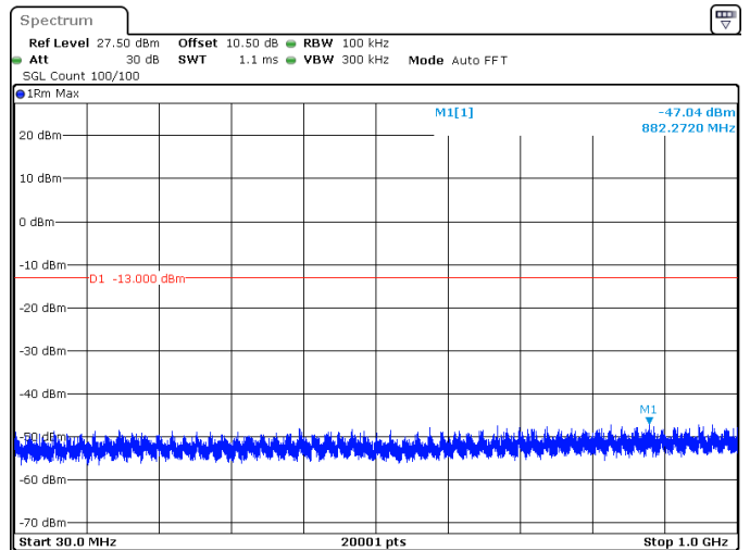
80MHz_30kHz_3740MHz_DFT-s-OFDM QPSK_RB216@0 -47.04 dBm
