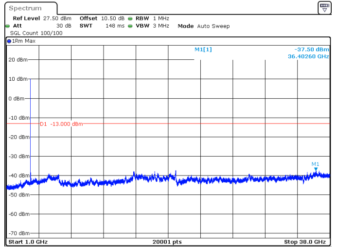
60MHz_30kHz_3750MHz_DFT-s-OFDM QPSK_RB1@0 -37.50 dBm
