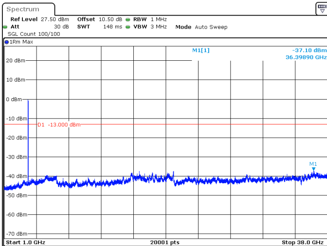
50MHz_30kHz_3750MHz_DFT-s-OFDM QPSK_RB128@0 -37.10 dBm
