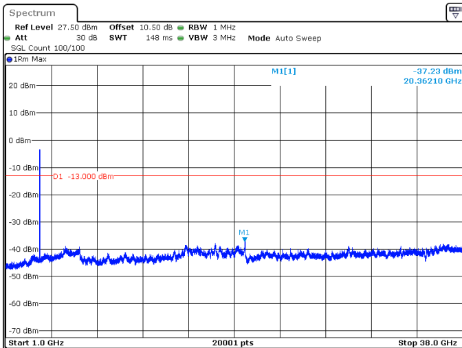
50MHz_15kHz_3750MHz_DFT-s-OFDM QPSK_RB270@0 -37.23 dBm
