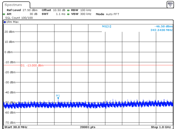
70MHz_30kHz_3765MHz_DFT-s-OFDM QPSK_RB180@0 -46.50 dBm
