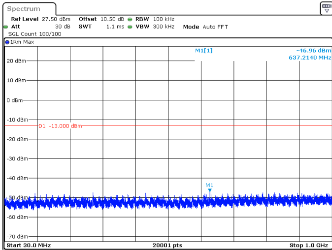
80MHz_30kHz_3740MHz_DFT-s-OFDM QPSK_RB1@216 -46.96 dBm
