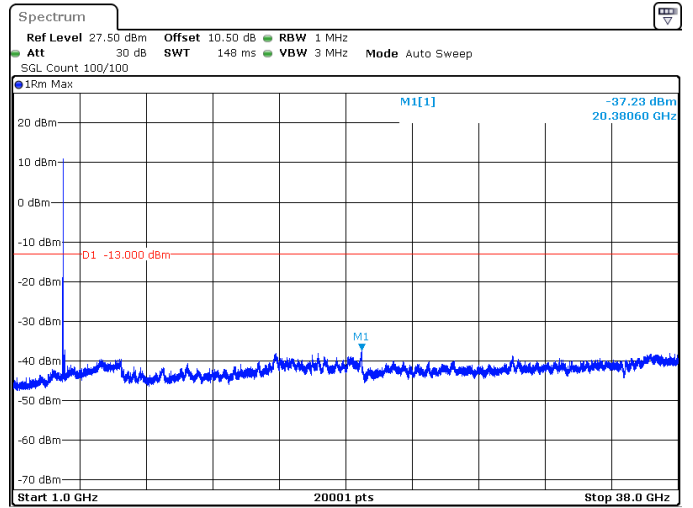
60MHz_30kHz_3770MHz_DFT-s-OFDM QPSK_RB1@0 -37.23 dBm
