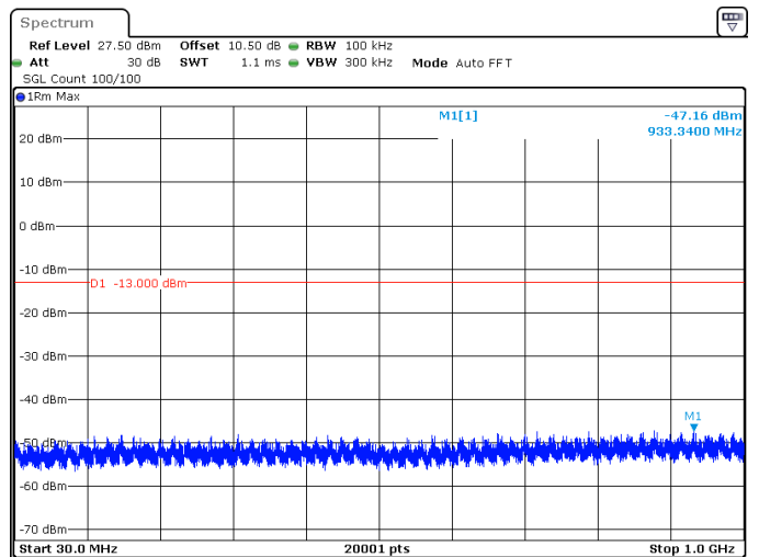
30MHz_30kHz_3750MHz_DFT-s-OFDM QPSK_RB75@0 -47.16 dBm
