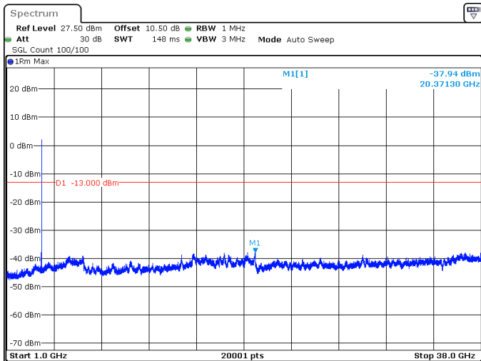
15MHz_30kHz_3707.5MHz_DFT-s-OFDM QPSK_RB36@0 -37.94 dBm
