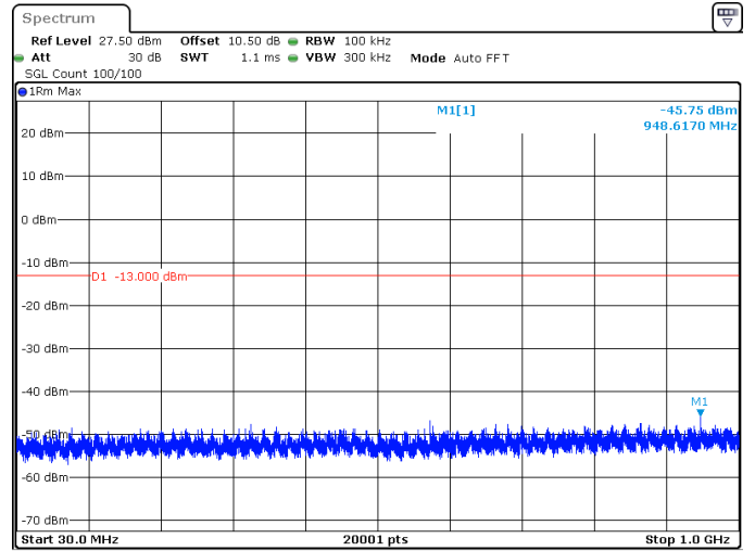
40MHz_30kHz_3750MHz_DFT-s-OFDM QPSK_RB1@0 -45.75 dBm
