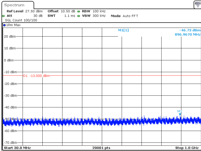
70MHz_30kHz_3750MHz_DFT-s-OFDM QPSK_RB1@0 -46.73 dBm
