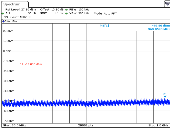
40MHz_30kHz_3780MHz_DFT-s-OFDM QPSK_RB1@0 -46.80 dBm
