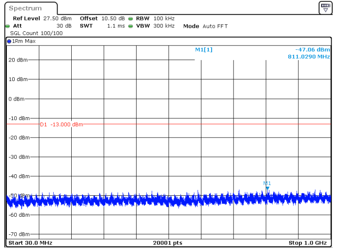
30MHz_15kHz_3715MHz_DFT-s-OFDM QPSK_RB1@0 -47.06 dBm
