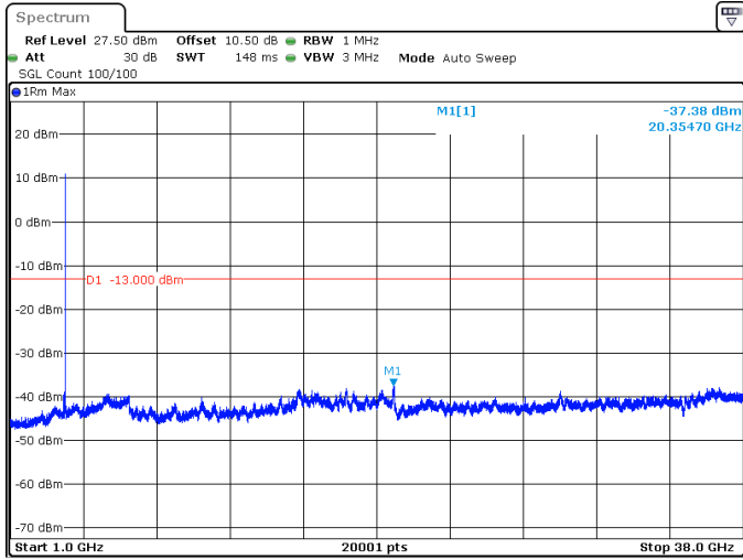
60MHz_30kHz_3750MHz_DFT-s-OFDM QPSK_RB1@161 -37.38 dBm
