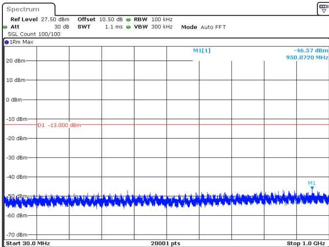
30MHz_15kHz_3785MHz_DFT-s-OFDM QPSK_RB160@0 -46.57 dBm
