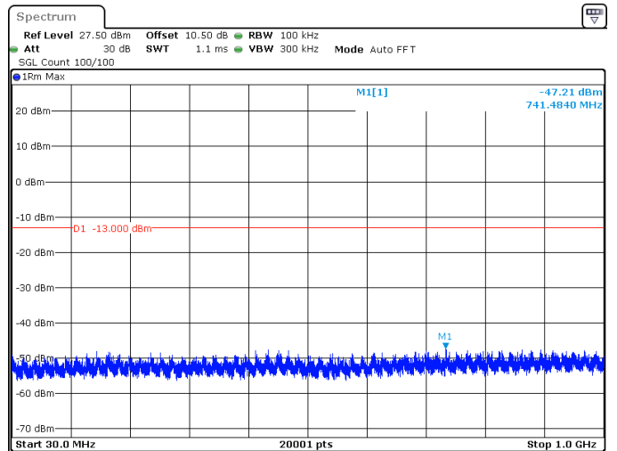
50MHz_30kHz_3725MHz_DFT-s-OFDM QPSK_RB128@0 -47.21 dBm
