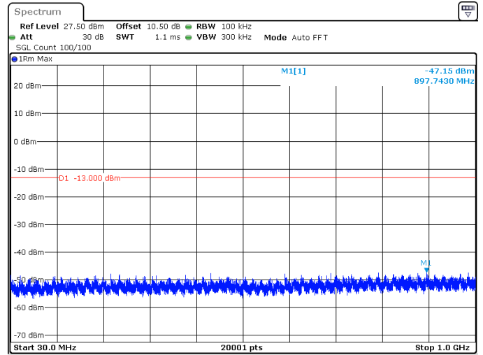
15MHz_30kHz_3750MHz_DFT-s-OFDM QPSK_RB1@0 -47.15 dBm
