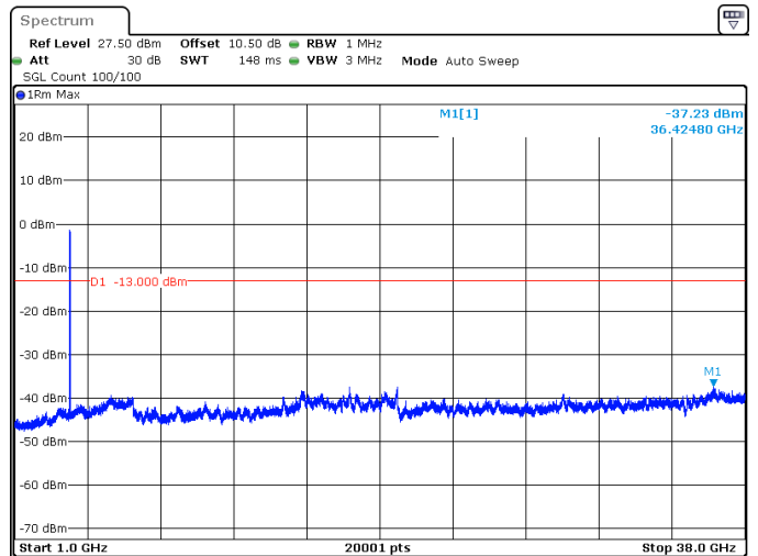
50MHz_30kHz_3775MHz_DFT-s-OFDM QPSK_RB128@0 -37.23 dBm
