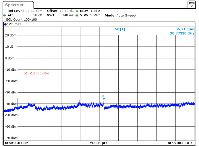
50MHz_30kHz_3725MHz_DFT-s-OFDM QPSK_RB1@0 -36.71 dBm
