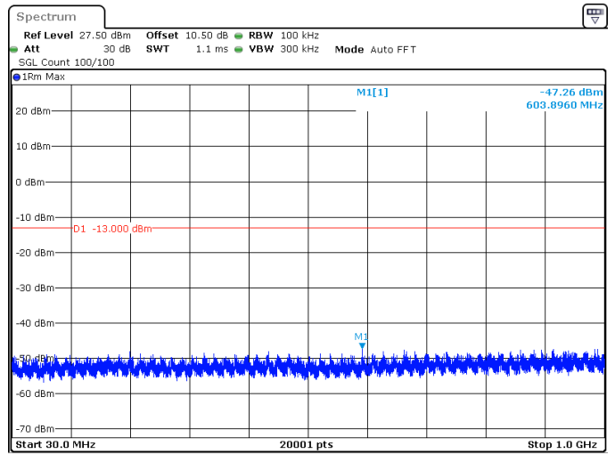
80MHz_30kHz_3740MHz_DFT-s-OFDM QPSK_RB1@0 -47.26 dBm
