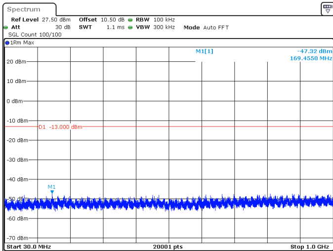
25MHz_30kHz_3712.5MHz_DFT-s-OFDM QPSK_RB1@0 -47.32 dBm
