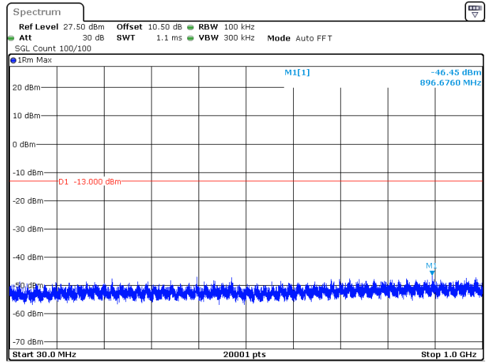
40MHz_15kHz_3720MHz_DFT-s-OFDM QPSK_RB1@0 -46.45 dBm
