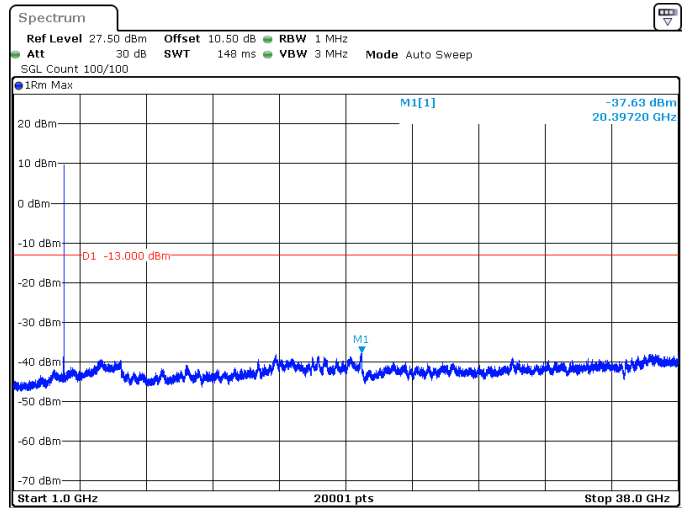
30MHz_30kHz_3785MHz_DFT-s-OFDM QPSK_RB1@77 -37.63 dBm
