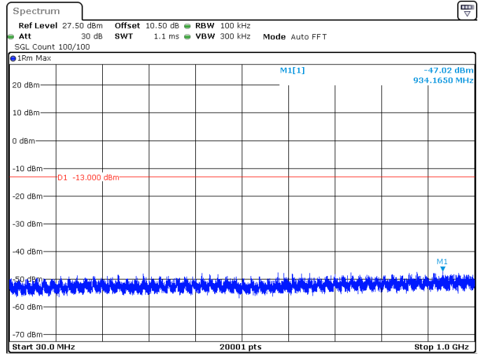
60MHz_30kHz_3750MHz_DFT-s-OFDM QPSK_RB1@161 -47.02 dBm
