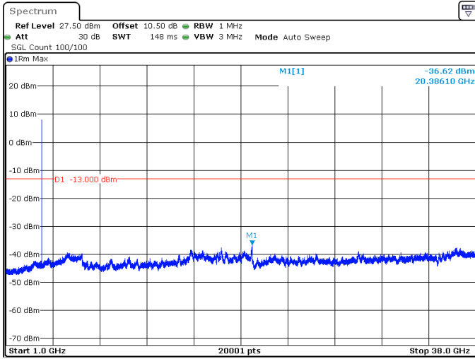
40MHz_15kHz_3780MHz_DFT-s-OFDM QPSK_RB1@215 -36.62 dBm
