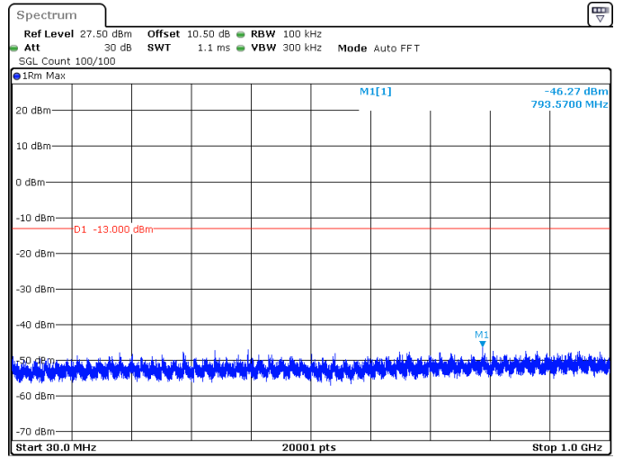
50MHz_30kHz_3750MHz_DFT-s-OFDM QPSK_RB1@0 -46.27 dBm
