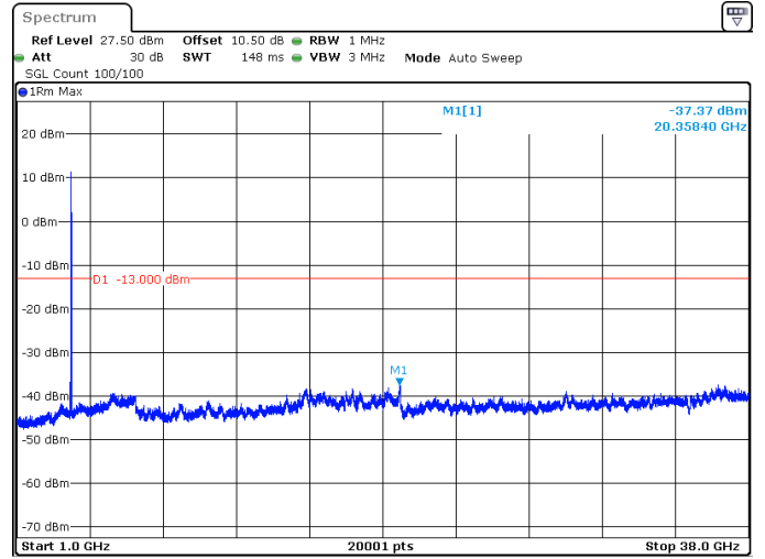
40MHz_30kHz_3720MHz_DFT-s-OFDM QPSK_RB1@105 -37.37 dBm
