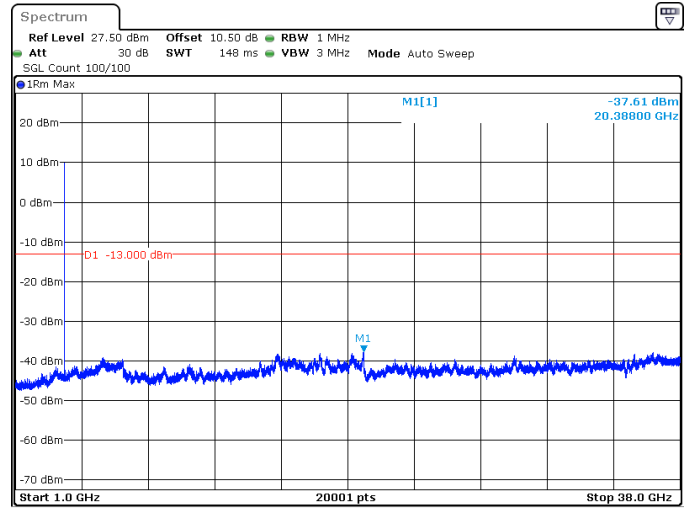
15MHz_30kHz_3707.5MHz_DFT-s-OFDM QPSK_RB1@0 -37.61 dBm
