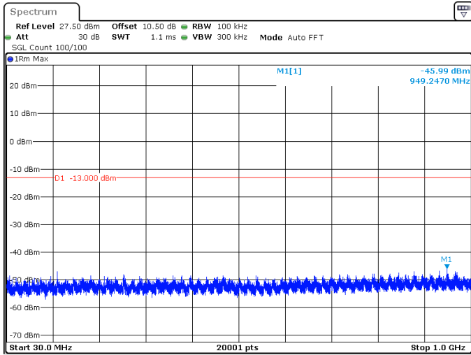
60MHz_30kHz_3770MHz_DFT-s-OFDM QPSK_RB1@0 -45.99 dBm
