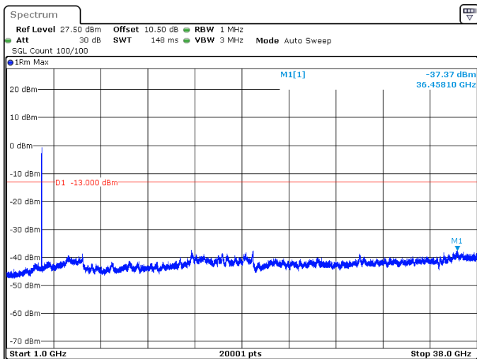
25MHz_30kHz_3750MHz_DFT-s-OFDM QPSK_RB64@0 -37.37 dBm
