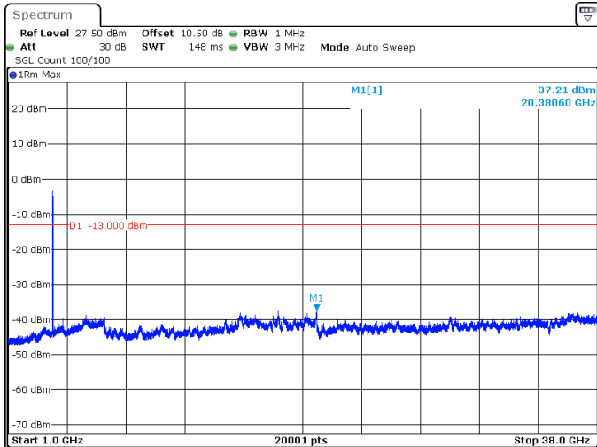
50MHz_15kHz_3775MHz_DFT-s-OFDM QPSK_RB270@0 -37.21 dBm
