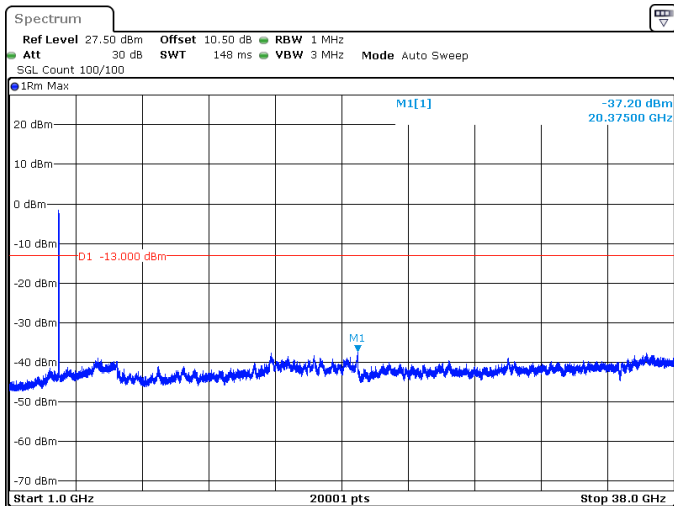
70MHz_30kHz_3750MHz_DFT-s-OFDM QPSK_RB180@0 -37.20 dBm
