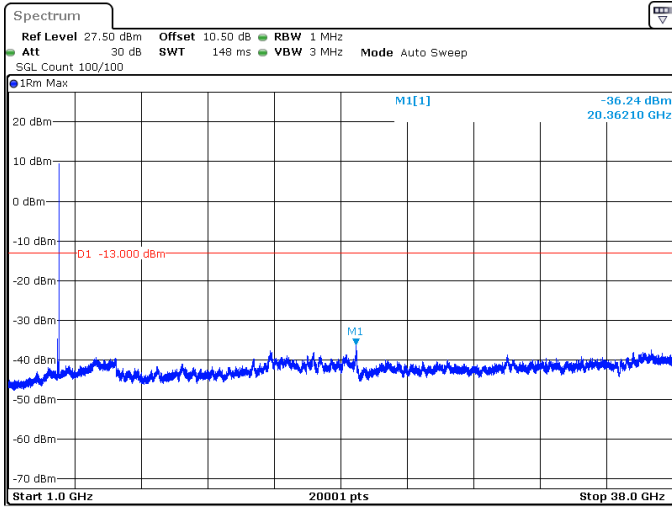
40MHz_30kHz_3780MHz_DFT-s-OFDM QPSK_RB1@105 -36.24 dBm
