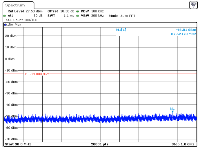
70MHz_30kHz_3765MHz_DFT-s-OFDM QPSK_RB1@188 -46.81 dBm
