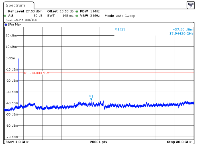
25MHz_15kHz_3712.5MHz_DFT-s-OFDM QPSK_RB128@0 -37.50 dBm
