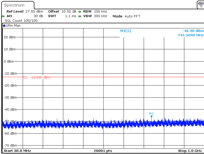
40MHz_15kHz_3780MHz_DFT-s-OFDM QPSK_RB1@0 -46.90 dBm
