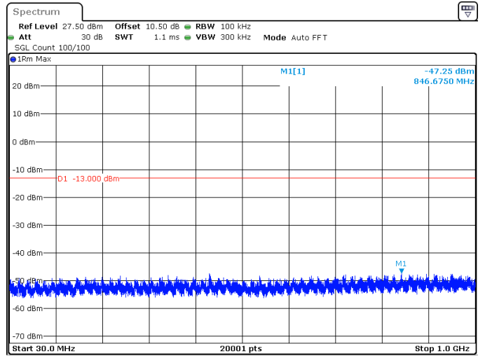
30MHz_30kHz_3750MHz_DFT-s-OFDM QPSK_RB1@0 -47.25 dBm
