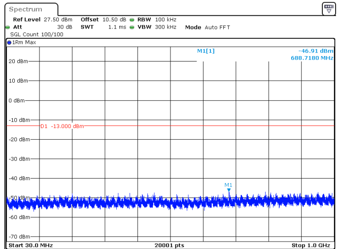
70MHz_30kHz_3750MHz_DFT-s-OFDM QPSK_RB180@0 -46.91 dBm
