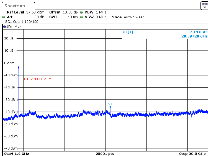
70MHz_30kHz_3765MHz_DFT-s-OFDM QPSK_RB180@0 -37.14 dBm
