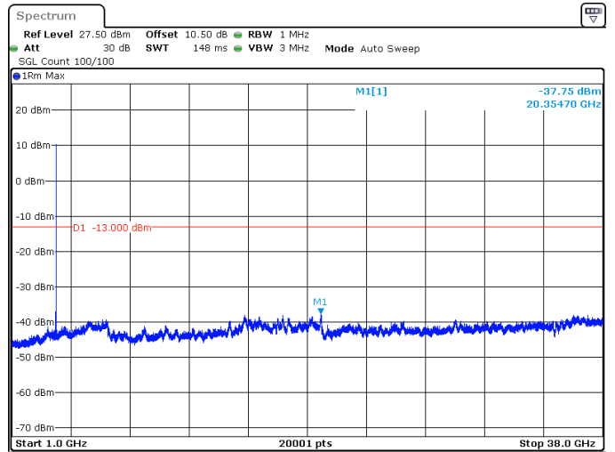
30MHz_30kHz_3750MHz_DFT-s-OFDM QPSK_RB1@77 -37.75 dBm
