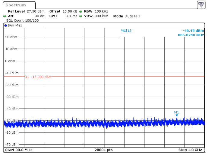
10MHz_15kHz_1775MHz_DFT-s-OFDM QPSK_RB1@0 -46.45 dBm
