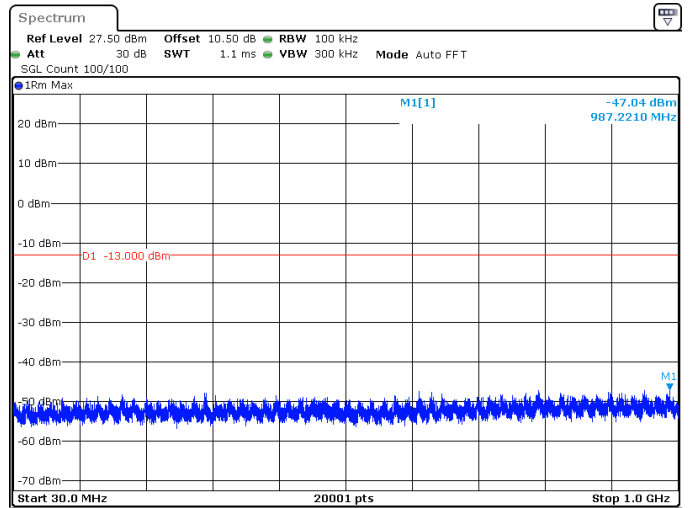
10MHz_30kHz_3455MHz_DFT-s-OFDM QPSK_RB1@23 -47.04 dBm
