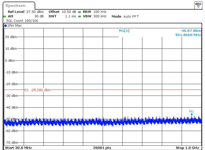
100MHz_30kHz_2640MHz_DFT-s-OFDM QPSK_RB270@0 -46.87 dBm
