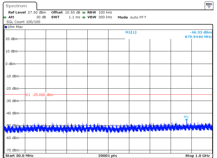
90MHz_30kHz_2644.98MHz_DFT-s-OFDM QPSK_RB243@0 -46.33 dBm
