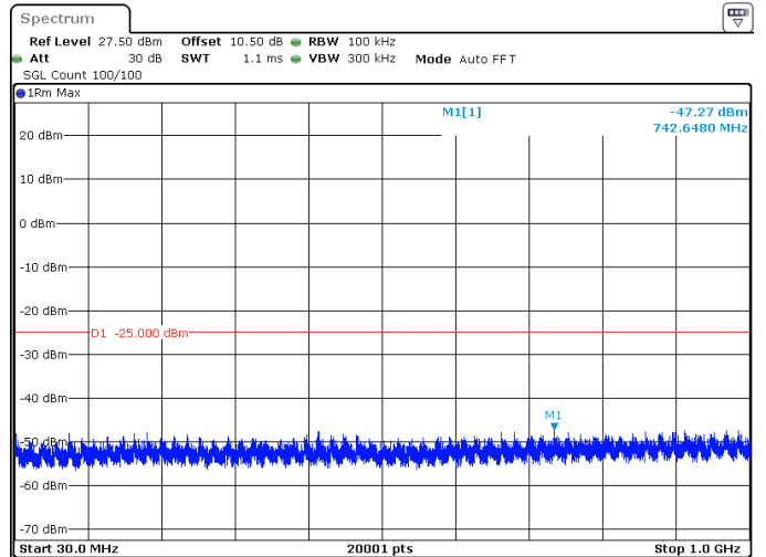
80MHz_30kHz_2592.99MHz_DFT-s-OFDM QPSK_RB216@0 -47.27 dBm
