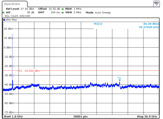
100MHz_30kHz_2592.99MHz_DFT-s-OFDM QPSK_RB1@0 -36.28 dBm
