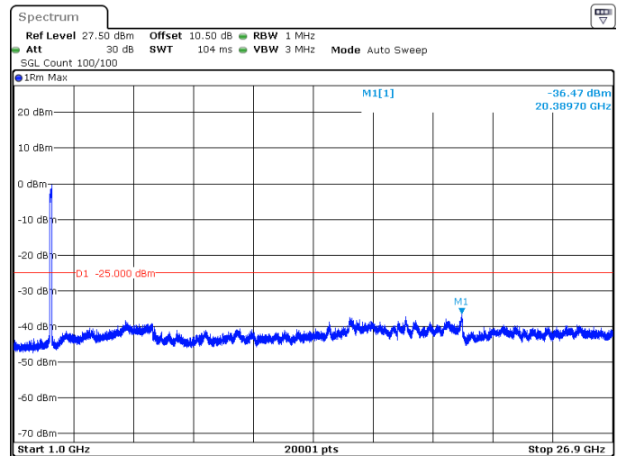
90MHz_30kHz_2592.99MHz_DFT-s-OFDM QPSK_RB243@0 -36.47 dBm
