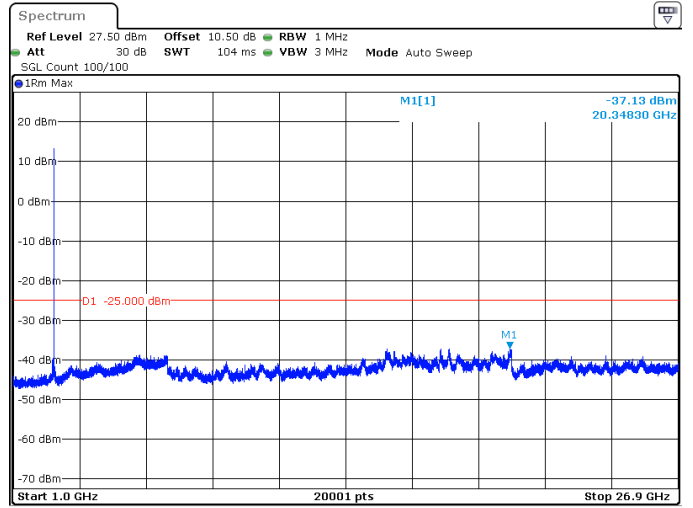
90MHz_30kHz_2541MHz_DFT-s-OFDM QPSK_RB1@244 -37.13 dBm
