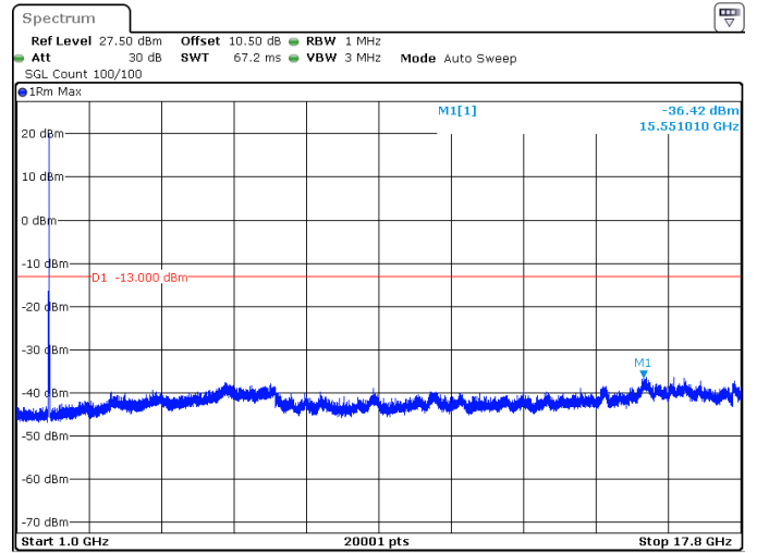
20MHz_15kHz_1745MHz_DFT-s-OFDM QPSK_RB1@0 -36.42 dBm
