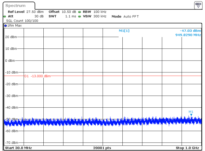
5MHz_15kHz_1712.5MHz_DFT-s-OFDM QPSK_RB25@0 -47.03 dBm
