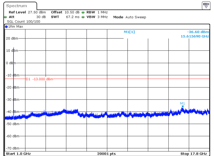
10MHz_15kHz_1715MHz_DFT-s-OFDM QPSK_RB50@0 -36.60 dBm
