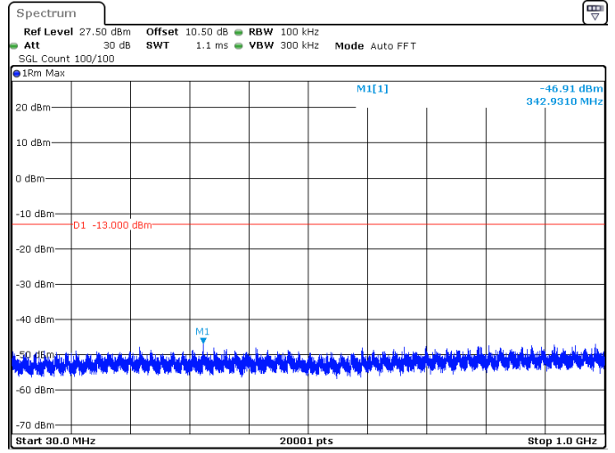
10MHz_30kHz_3455MHz_DFT-s-OFDM QPSK_RB1@0 -46.91 dBm
