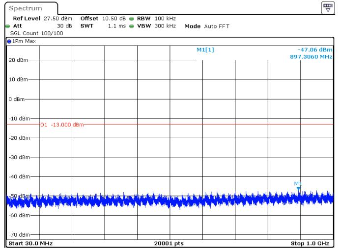
40MHz_15kHz_1760MHz_DFT-s-OFDM QPSK_RB216@0 -47.06 dBm
