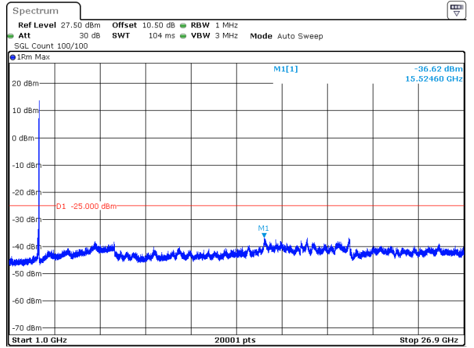
90MHz_30kHz_2644.98MHz_DFT-s-OFDM QPSK_RB1@244 -36.62 dBm
