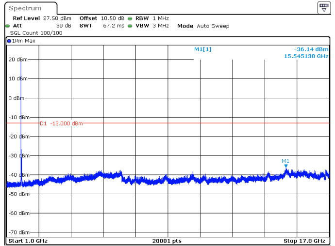
30MHz_15kHz_1765MHz_DFT-s-OFDM QPSK_RB1@0 -36.14 dBm
