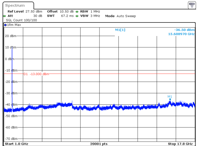
20MHz_15kHz_1720MHz_DFT-s-OFDM QPSK_RB100@0 -36.50 dBm
