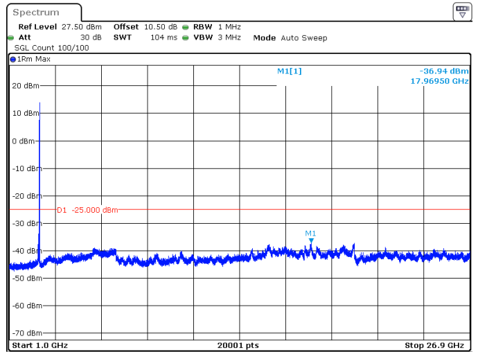
100MHz_30kHz_2640MHz_DFT-s-OFDM QPSK_RB1@272 -36.94 dBm
