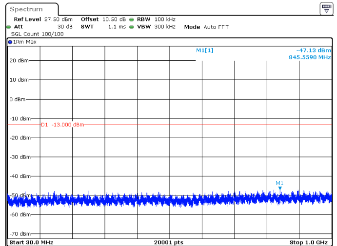
10MHz_15kHz_1745MHz_DFT-s-OFDM QPSK_RB50@0 -47.13 dBm
