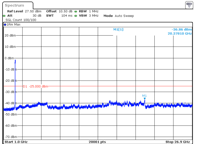
100MHz_30kHz_2592.99MHz_DFT-s-OFDM QPSK_RB270@0 -36.86 dBm
