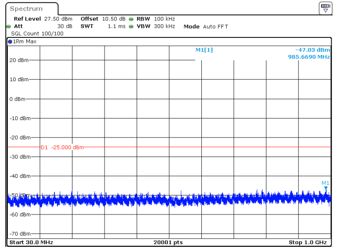
80MHz_30kHz_2649.99MHz_DFT-s-OFDM QPSK_RB1@216 -47.03 dBm
