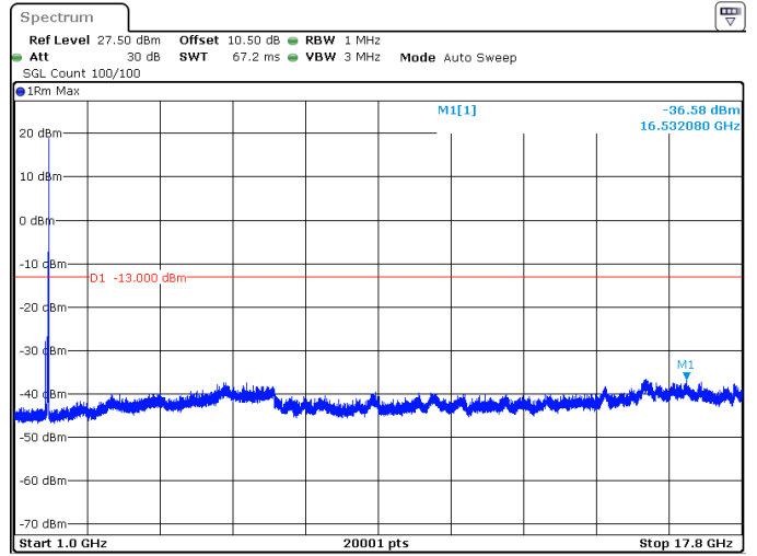
40MHz_15kHz_1760MHz_DFT-s-OFDM QPSK_RB1@215 -36.58 dBm
