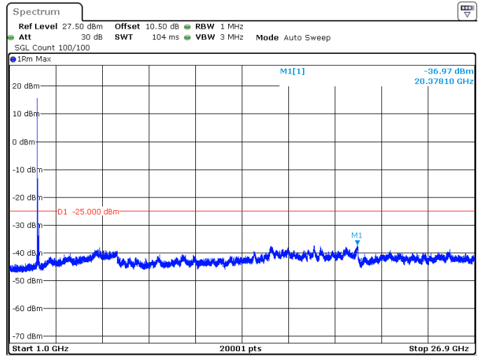
80MHz_30kHz_2592.99MHz_DFT-s-OFDM QPSK_RB1@0 -36.97 dBm
