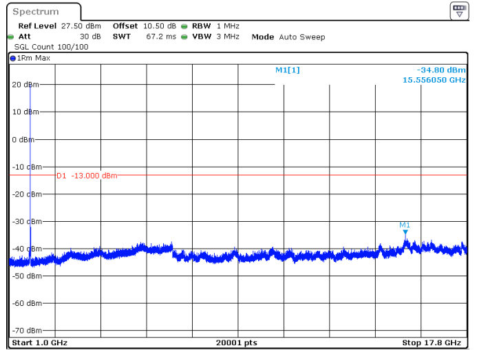
20MHz_15kHz_1770MHz_DFT-s-OFDM QPSK_RB1@0 -34.80 dBm
