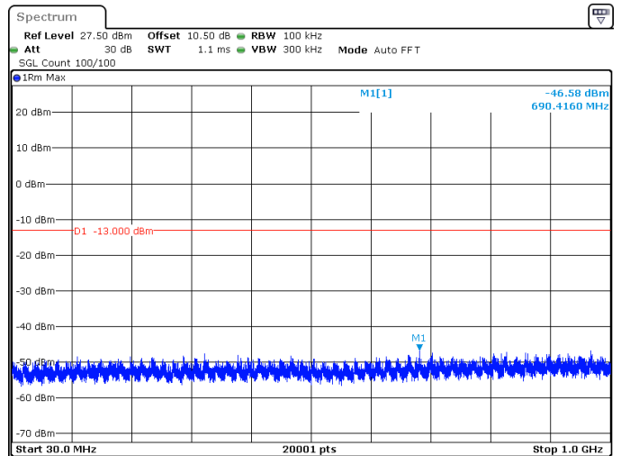
10MHz_30kHz_3455MHz_DFT-s-OFDM QPSK_RB24@0 -46.58 dBm
