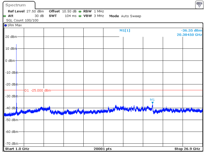
90MHz_30kHz_2644.98MHz_DFT-s-OFDM QPSK_RB1@0 -36.35 dBm
