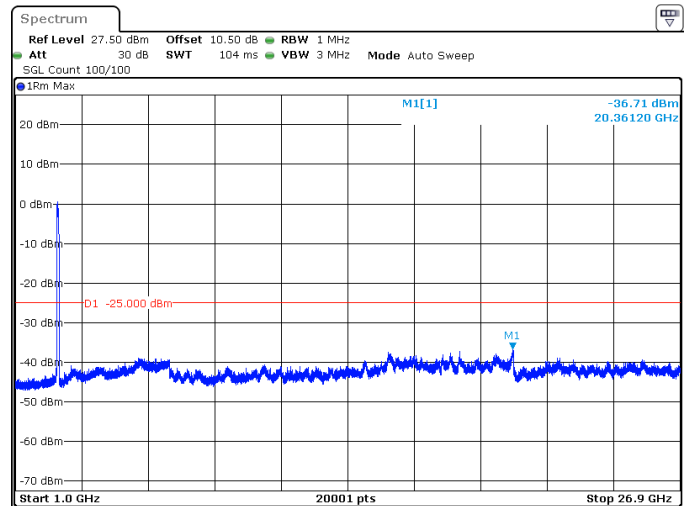
80MHz_30kHz_2649.99MHz_DFT-s-OFDM QPSK_RB216@0 -36.71 dBm
