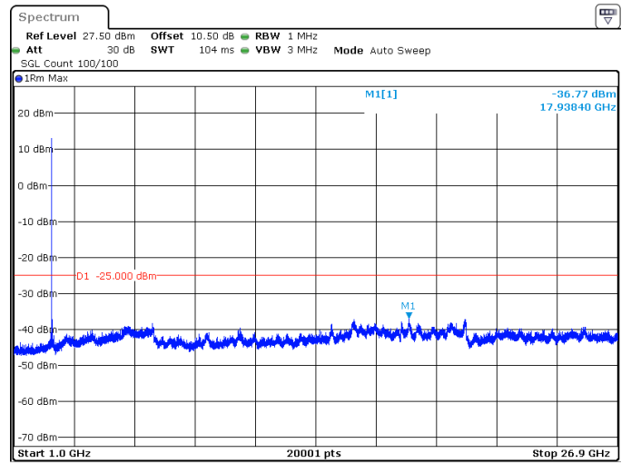
80MHz_30kHz_2649.99MHz_DFT-s-OFDM QPSK_RB1@0 -36.77 dBm
