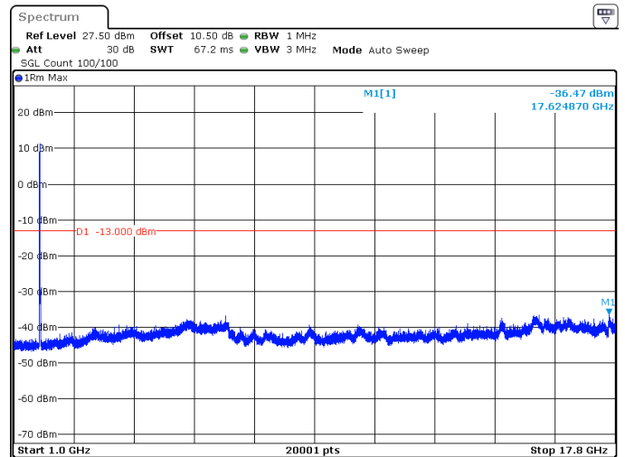
15MHz_15kHz_1717.5MHz_DFT-s-OFDM QPSK_RB75@0 -36.47 dBm
