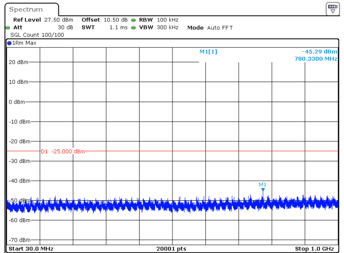
100MHz_30kHz_2640MHz_DFT-s-OFDM QPSK_RB1@0 -45.29 dBm
