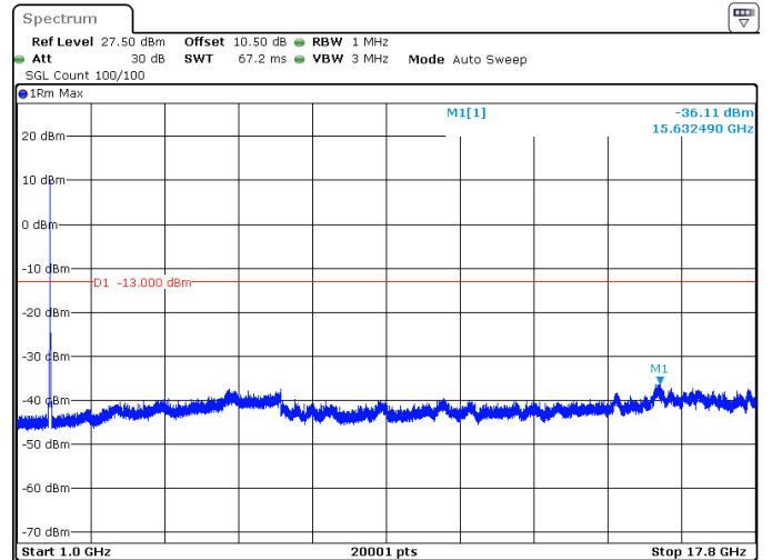
20MHz_15kHz_1745MHz_DFT-s-OFDM QPSK_RB100@0 -36.11 dBm
