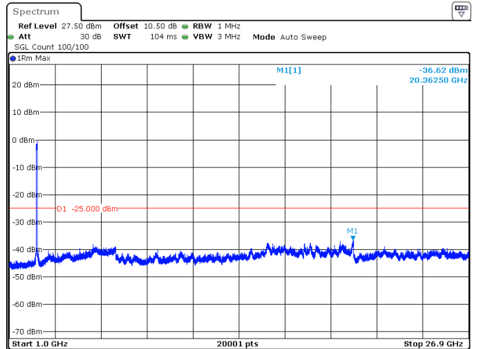
90MHz_30kHz_2541MHz_DFT-s-OFDM QPSK_RB243@0 -36.62 dBm
