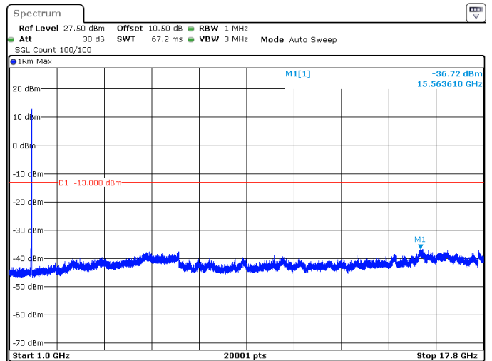
10MHz_15kHz_1775MHz_DFT-s-OFDM QPSK_RB50@0 -36.72 dBm
