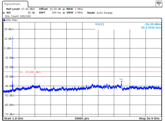
90MHz_30kHz_2541MHz_DFT-s-OFDM QPSK_RB1@0 -36.39 dBm
