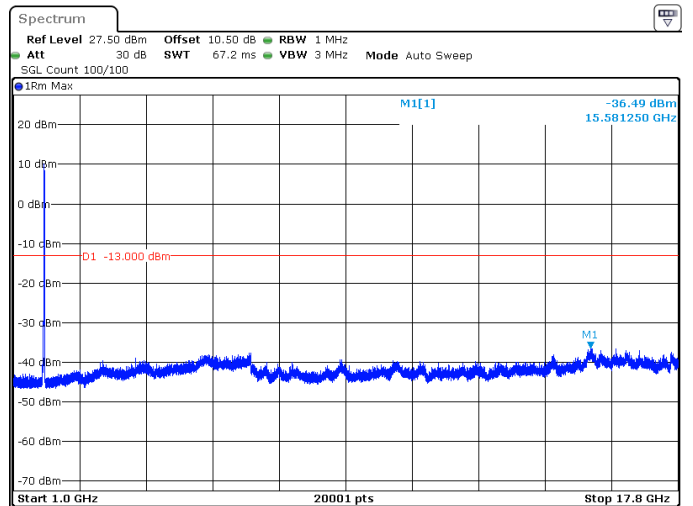
20MHz_15kHz_1770MHz_DFT-s-OFDM QPSK_RB100@0 -36.49 dBm
