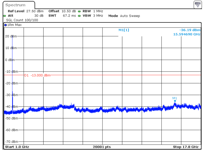
20MHz_15kHz_1720MHz_DFT-s-OFDM QPSK_RB1@0 -36.19 dBm
