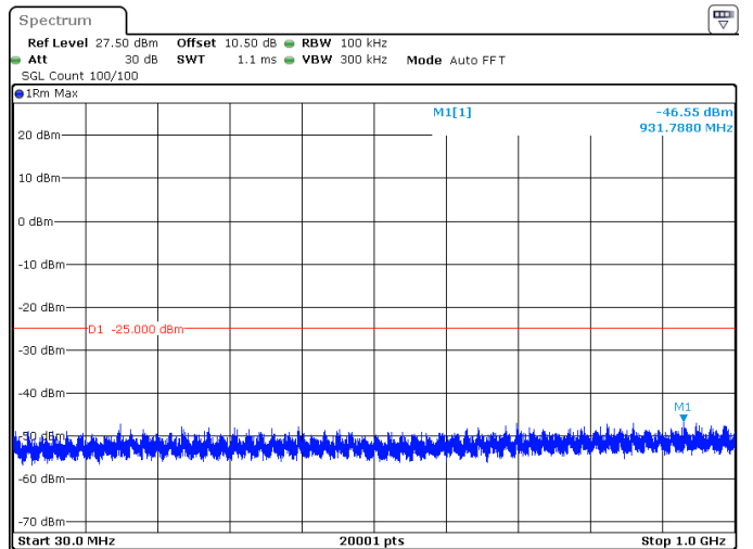
100MHz_30kHz_2546.01MHz_DFT-s-OFDM QPSK_RB270@0 -46.55 dBm
