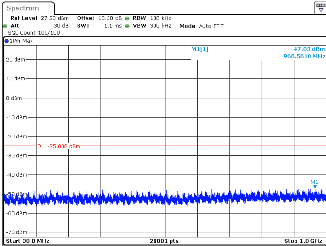
40MHz_30kHz_2670MHz_DFT-s-OFDM QPSK_RB1@0 -47.03 dBm
