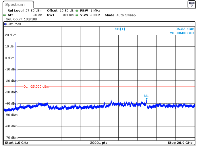
10MHz_30kHz_2592.99MHz_DFT-s-OFDM QPSK_RB1@23 -36.55 dBm
