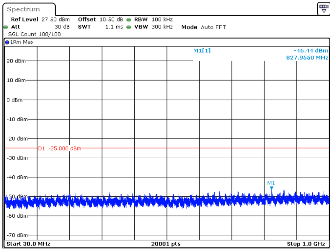
20MHz_15kHz_2593.005MHz_DFT-s-OFDM QPSK_RB1@0 -46.44 dBm
