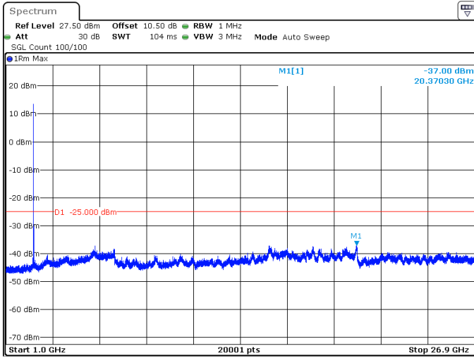
20MHz_30kHz_2506.02MHz_DFT-s-OFDM QPSK_RB1@50 -37.00 dBm
