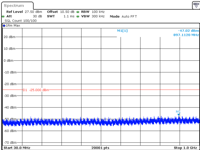
20MHz_15kHz_2506.005MHz_DFT-s-OFDM QPSK_RB100@0 -47.02 dBm
