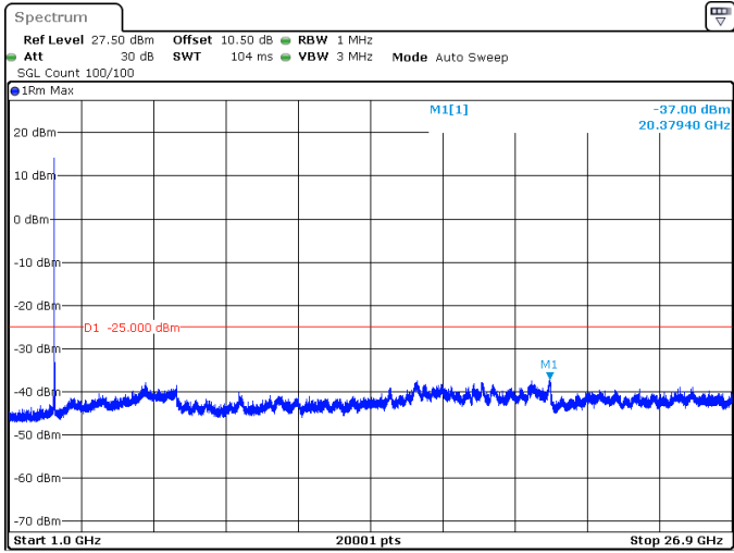
50MHz_15kHz_2593.005MHz_DFT-s-OFDM QPSK_RB1@269 -37.00 dBm
