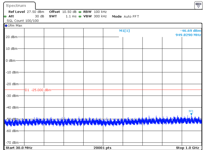
60MHz_30kHz_2659.98MHz_DFT-s-OFDM QPSK_RB162@0 -46.69 dBm
