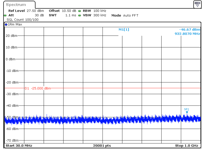
10MHz_30kHz_2685MHz_DFT-s-OFDM QPSK_RB1@23 -46.67 dBm
