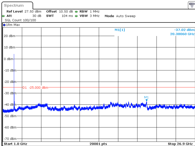
30MHz_30kHz_2511MHz_DFT-s-OFDM QPSK_RB75@0 -37.02 dBm
