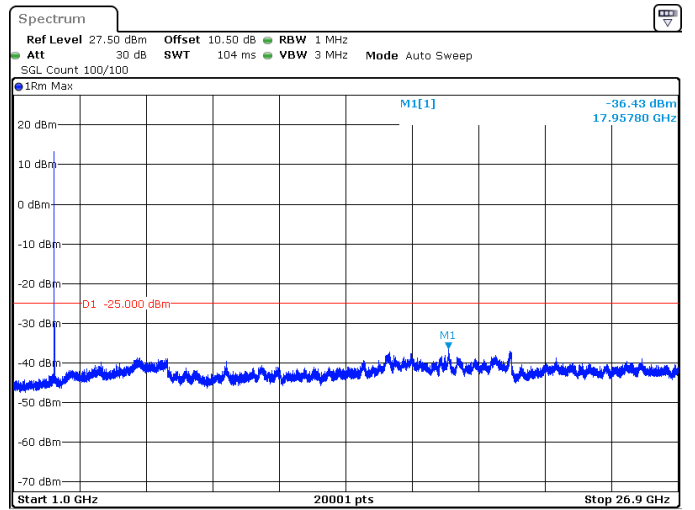
20MHz_15kHz_2593.005MHz_DFT-s-OFDM QPSK_RB1@0 -36.43 dBm
