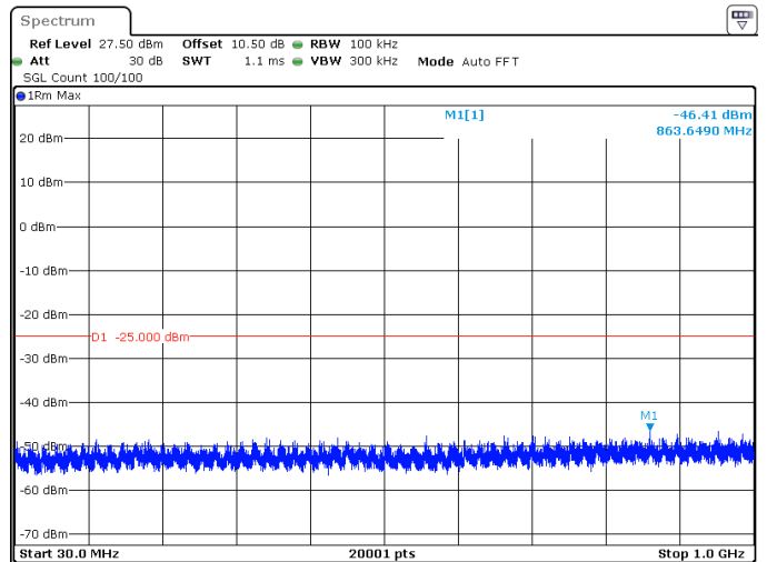
30MHz_30kHz_2674.98MHz_DFT-s-OFDM QPSK_RB75@0 -46.41 dBm
