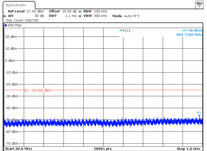
15MHz_30kHz_2682.48MHz_DFT-s-OFDM QPSK_RB36@0 -47.46 dBm
