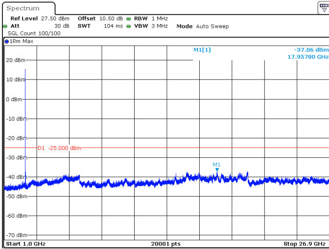
20MHz_30kHz_2679.99MHz_DFT-s-OFDM QPSK_RB1@0 -37.06 dBm
