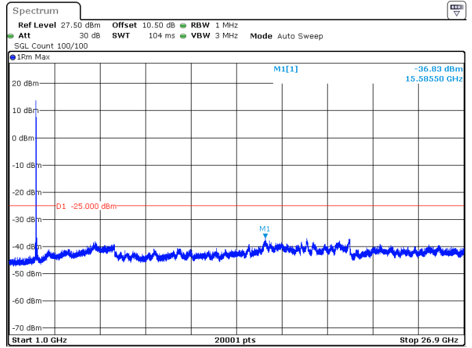
30MHz_30kHz_2511MHz_DFT-s-OFDM QPSK_RB1@77 -36.83 dBm
