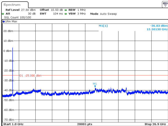
30MHz_30kHz_2592.99MHz_DFT-s-OFDM QPSK_RB75@0 -36.83 dBm
