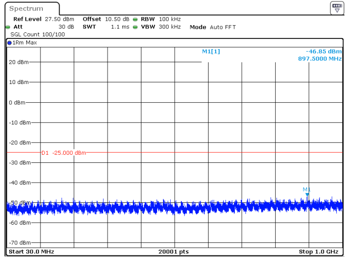
20MHz_30kHz_2592.99MHz_DFT-s-OFDM QPSK_RB1@0 -46.85 dBm
