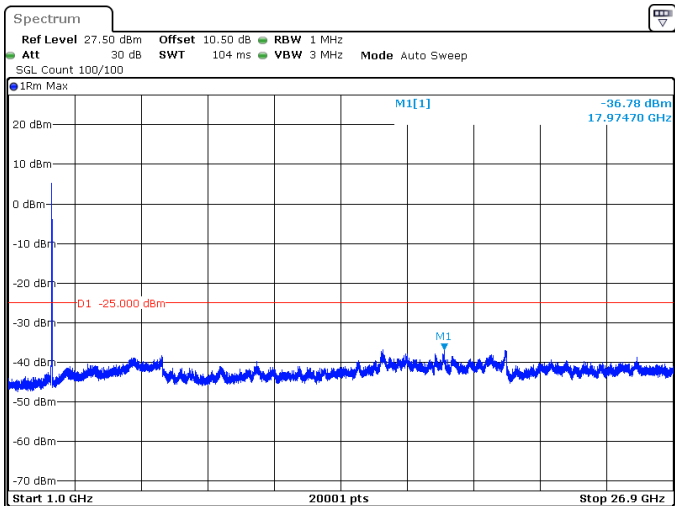
20MHz_15kHz_2679.99MHz_DFT-s-OFDM QPSK_RB100@0 -36.78 dBm
