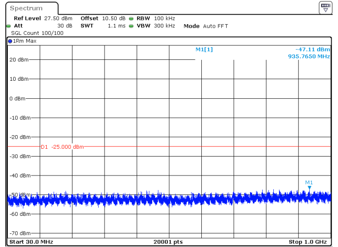
60MHz_30kHz_2592.99MHz_DFT-s-OFDM QPSK_RB1@0 -47.11 dBm
