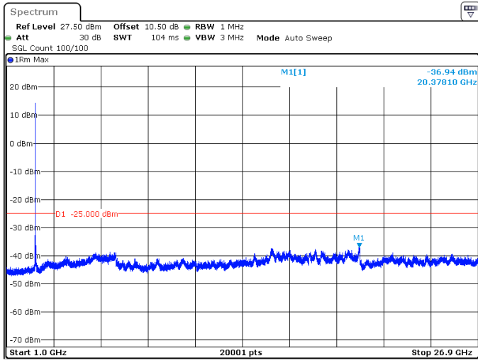
60MHz_30kHz_2592.99MHz_DFT-s-OFDM QPSK_RB1@0 -36.94 dBm
