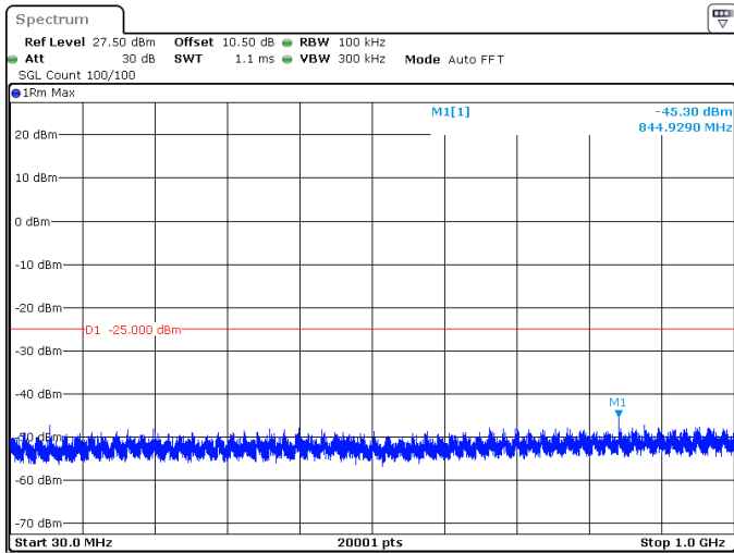
60MHz_30kHz_2659.98MHz_DFT-s-OFDM QPSK_RB1@161 -45.30 dBm
