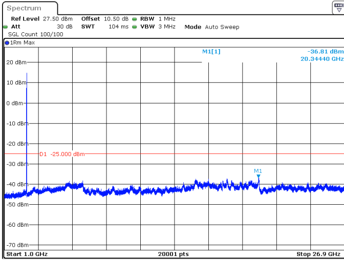
20MHz_30kHz_2679.99MHz_DFT-s-OFDM QPSK_RB1@50 -36.81 dBm
