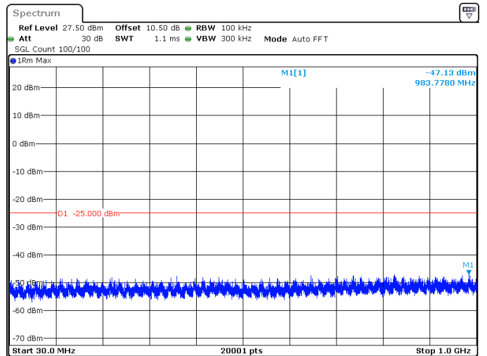
20MHz_15kHz_2679.99MHz_DFT-s-OFDM QPSK_RB100@0 -47.13 dBm
