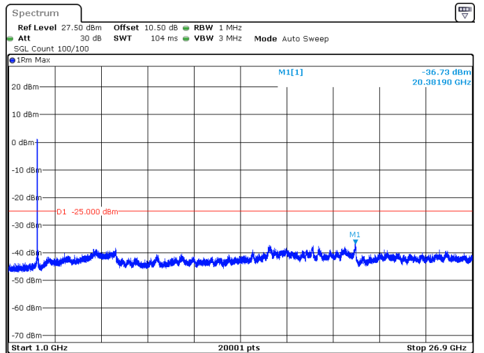
50MHz_15kHz_2593.005MHz_DFT-s-OFDM QPSK_RB270@0 -36.73 dBm
