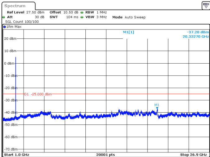
20MHz_15kHz_2593.005MHz_DFT-s-OFDM QPSK_RB100@0 -37.20 dBm
