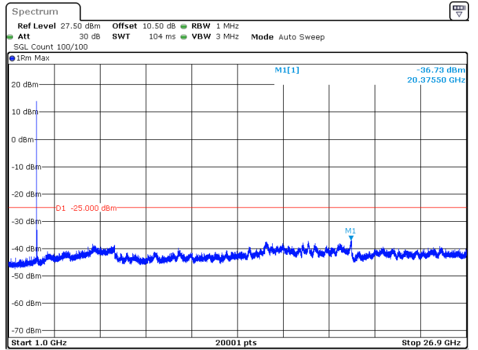
30MHz_15kHz_2593.005MHz_DFT-s-OFDM QPSK_RB1@0 -36.73 dBm
