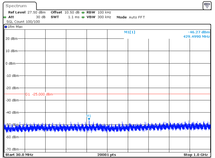
20MHz_15kHz_2679.99MHz_DFT-s-OFDM QPSK_RB1@0 -46.27 dBm
