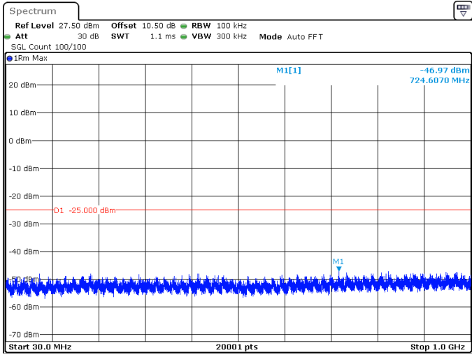
20MHz_15kHz_2506.005MHz_DFT-s-OFDM QPSK_RB1@105 -46.97 dBm
