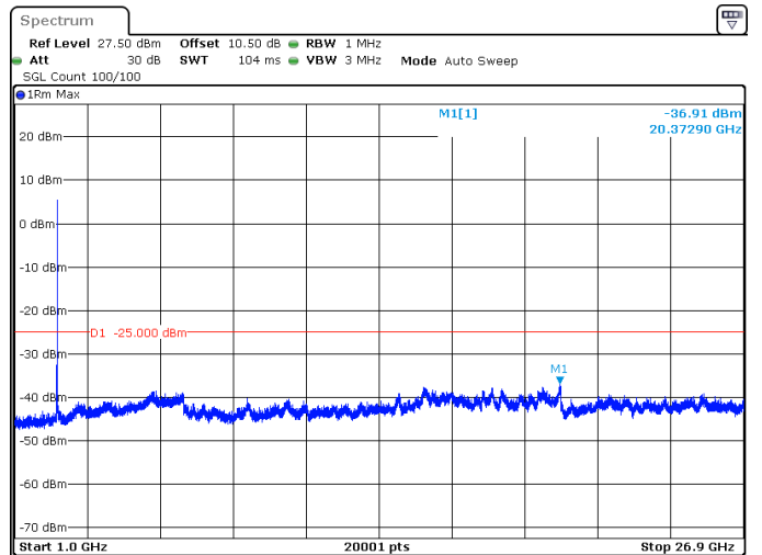
20MHz_15kHz_2506.005MHz_DFT-s-OFDM QPSK_RB100@0 -36.91 dBm
