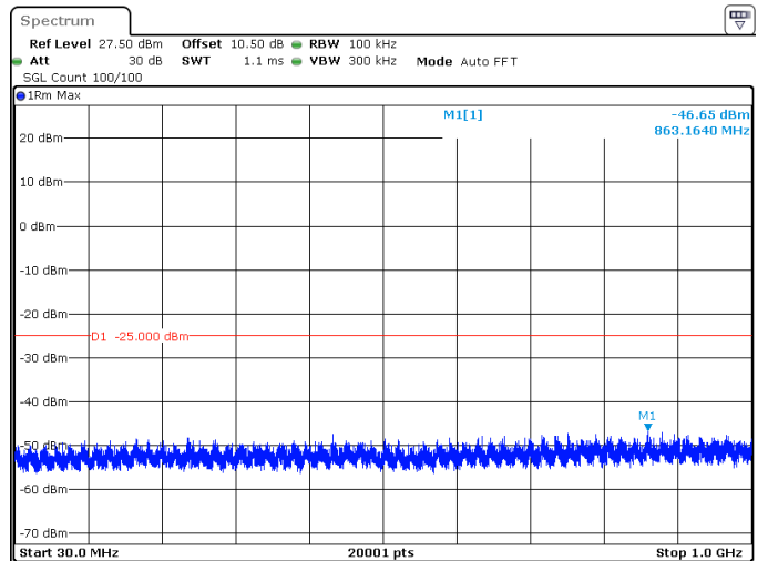
40MHz_30kHz_2670MHz_DFT-s-OFDM QPSK_RB100@0 -46.65 dBm
