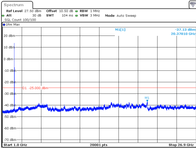
10MHz_30kHz_2592.99MHz_DFT-s-OFDM QPSK_RB1@0 -37.13 dBm
