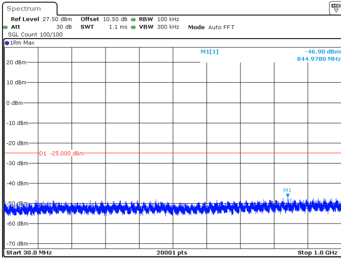
20MHz_30kHz_2506.02MHz_DFT-s-OFDM QPSK_RB1@0 -46.90 dBm
