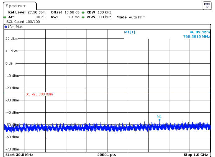
20MHz_30kHz_2592.99MHz_DFT-s-OFDM QPSK_RB50@0 -46.89 dBm
