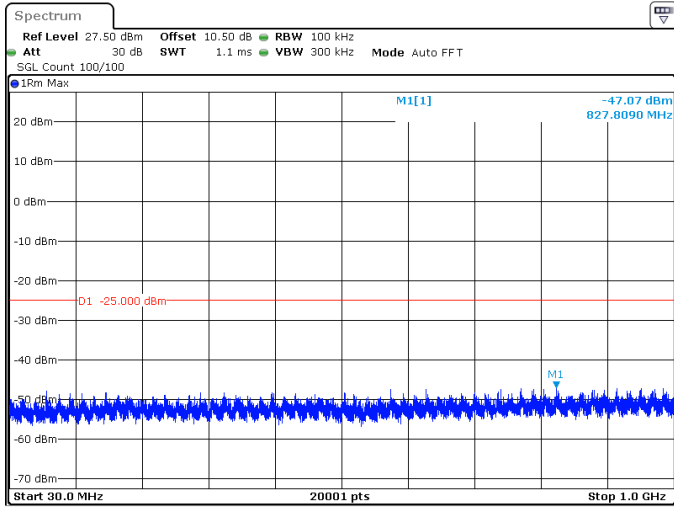
30MHz_30kHz_2511MHz_DFT-s-OFDM QPSK_RB1@77 -47.07 dBm
