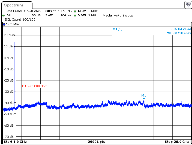
20MHz_15kHz_2593.005MHz_DFT-s-OFDM QPSK_RB1@105 -36.84 dBm
