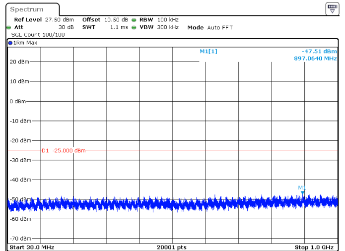
20MHz_30kHz_2506.02MHz_DFT-s-OFDM QPSK_RB50@0 -47.51 dBm
