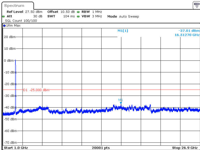
60MHz_30kHz_2659.98MHz_DFT-s-OFDM QPSK_RB162@0 -37.01 dBm
