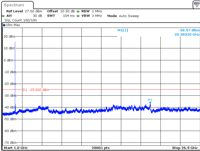
40MHz_15kHz_2670MHz_DFT-s-OFDM QPSK_RB1@0 -36.97 dBm
