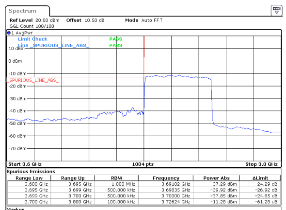
50MHz_15kHz_3725MHz_DFT-s-OFDM QPSK_RB270@0&-37.29 dBm
