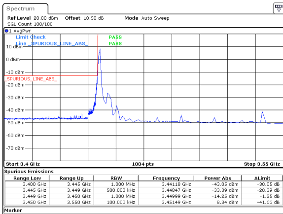
90MHz_30kHz_3495MHz_DFT-s-OFDM QPSK_RB1@0&-14.25 dBm
