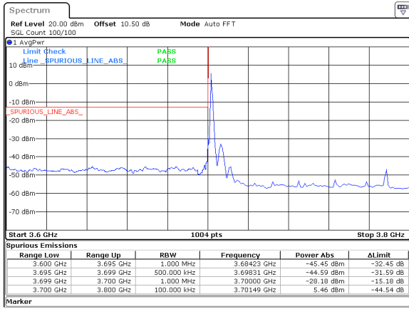
90MHz_30kHz_3745MHz_DFT-s-OFDM QPSK_RB1@0&-28.18 dBm
