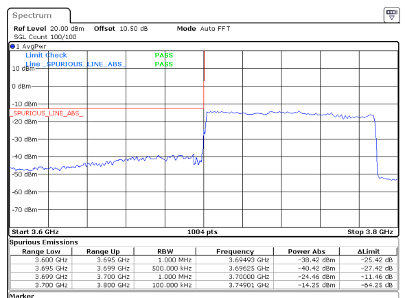
90MHz_30kHz_3745MHz_DFT-s-OFDM QPSK_RB243@0&-24.46 dBm
