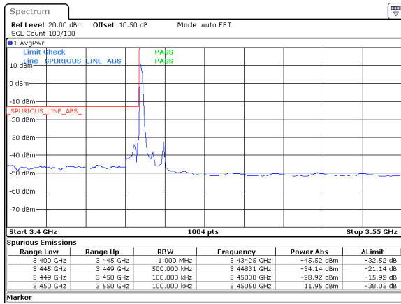
10MHz_30kHz_3455MHz_DFT-s-OFDM QPSK_RB1@0&-28.92 dBm
