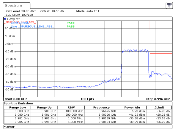
20MHz_30kHz_3970MHz_DFT-s-OFDM QPSK_RB50@0&-36.58 dBm
