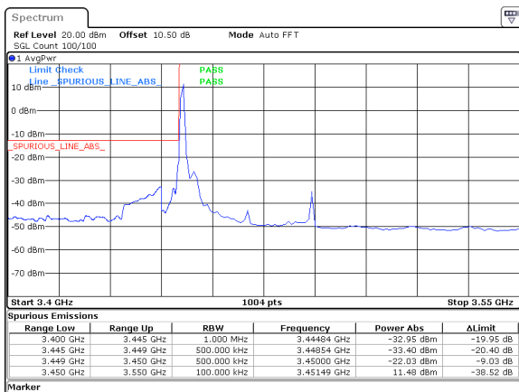
40MHz_30kHz_3470MHz_DFT-s-OFDM QPSK_RB1@0&-22.03 dBm
