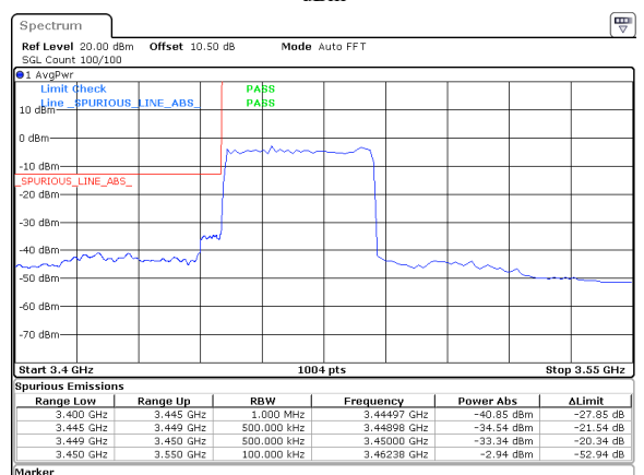
40MHz_30kHz_3470MHz_DFT-s-OFDM QPSK_RB100@0&-33.34 dBm
