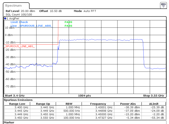
80MHz_30kHz_3490MHz_DFT-s-OFDM QPSK_RB216@0&-15.20 dBm
