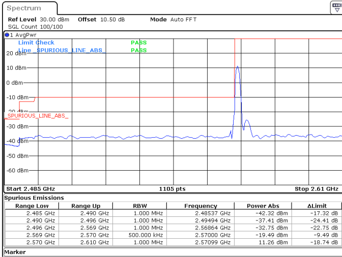
40MHz_30kHz_2590MHz_DFT-s-OFDM QPSK_RB1@0 -19.49 dBm
