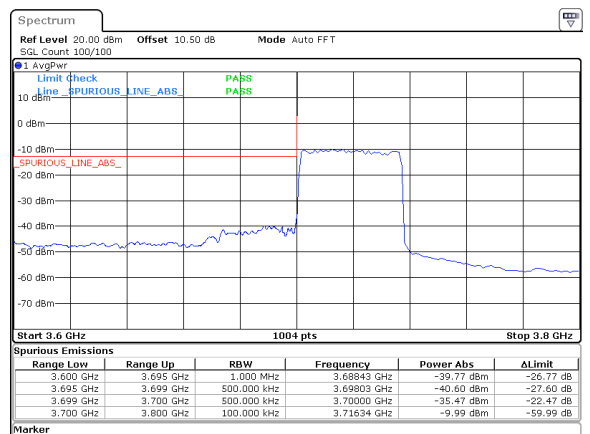
40MHz_30kHz_3720MHz_DFT-s-OFDM QPSK_RB100@0&-35.47 dBm
