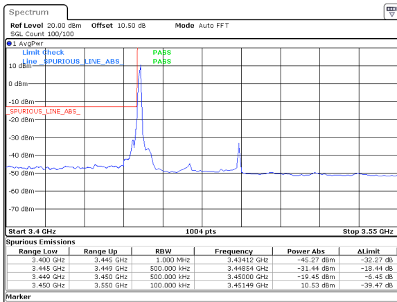
40MHz_30kHz_3470MHz_DFT-s-OFDM QPSK_RB1@0&-19.45 dBm
