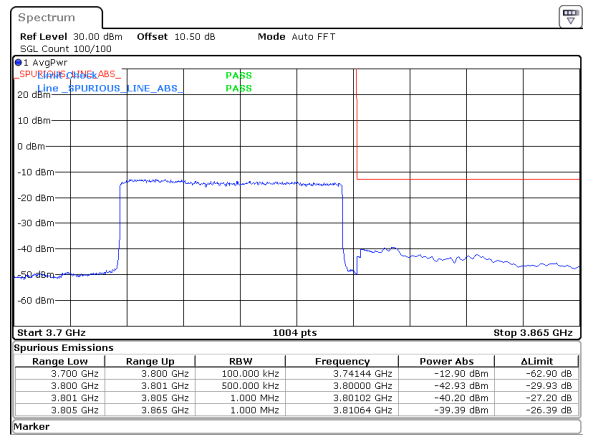
70MHz_30kHz_3765MHz_DFT-s-OFDM QPSK_RB180@0&-39.39 dBm
