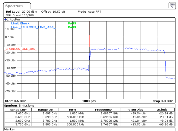
90MHz_30kHz_3745MHz_DFT-s-OFDM QPSK_RB243@0&-21.04 dBm
