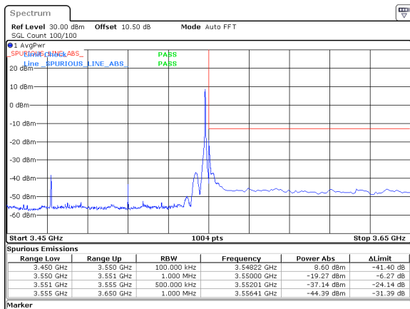
80MHz_30kHz_3510MHz_DFT-s-OFDM QPSK_RB1@216&-19.27 dBm
