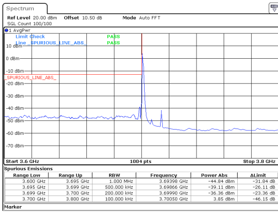
15MHz_30kHz_3707.5MHz_DFT-s-OFDM QPSK_RB1@0&-36.36 dBm
