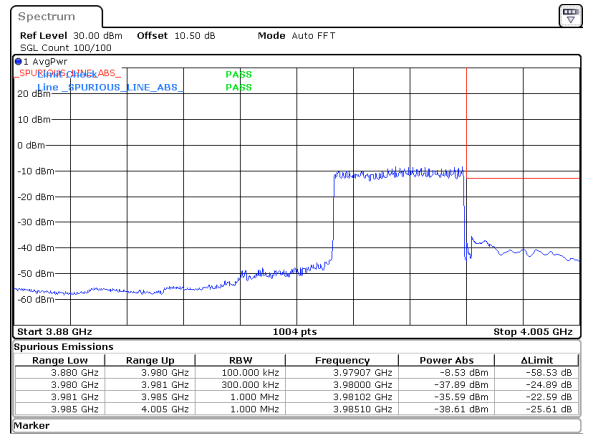
30MHz_15kHz_3965MHz_DFT-s-OFDM QPSK_RB160@0&-35.59 dBm
