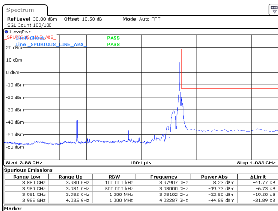
60MHz_30kHz_3950MHz_DFT-s-OFDM QPSK_RB1@161&-19.73 dBm
