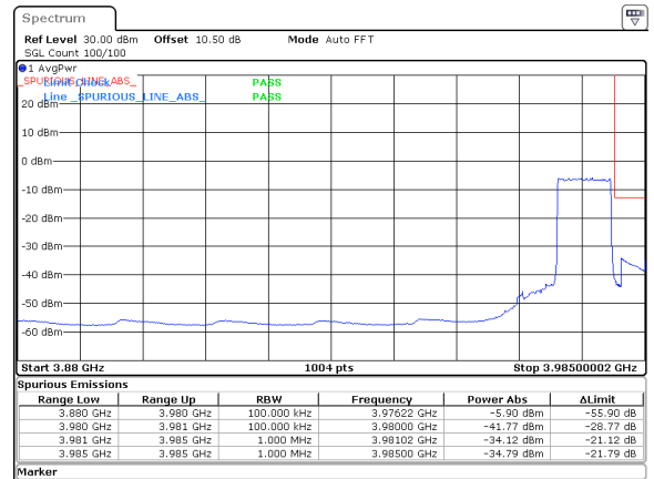
10MHz_15kHz_3975MHz_DFT-s-OFDM QPSK_RB50@0&-34.12 dBm
