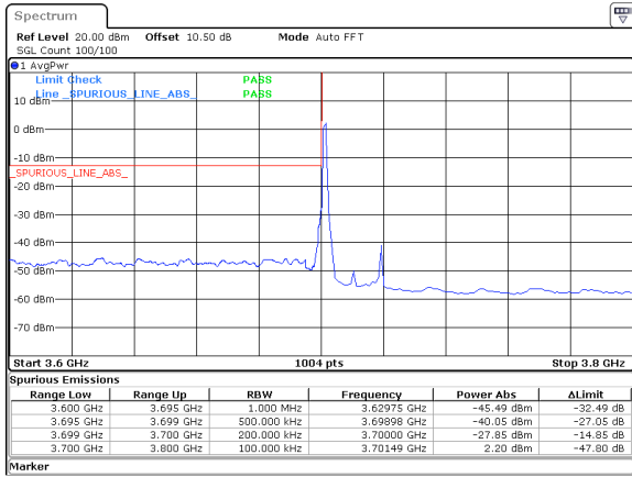
20MHz_30kHz_3710MHz_DFT-s-OFDM QPSK_RB1@0&-27.85 dBm
