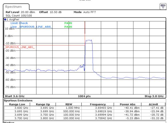
10MHz_30kHz_3705MHz_DFT-s-OFDM QPSK_RB24@0&-38.94 dBm
