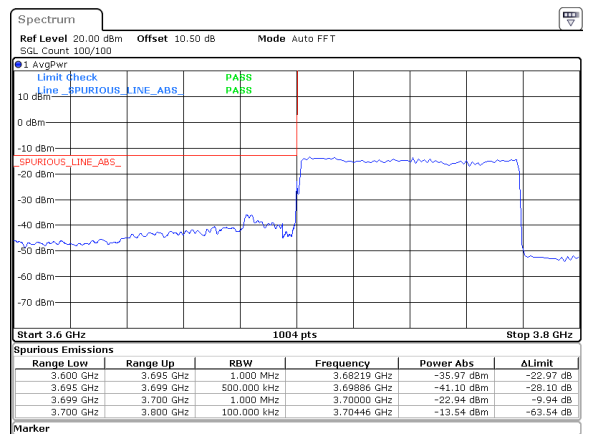
80MHz_30kHz_3740MHz_DFT-s-OFDM QPSK_RB216@0&-22.94 dBm
