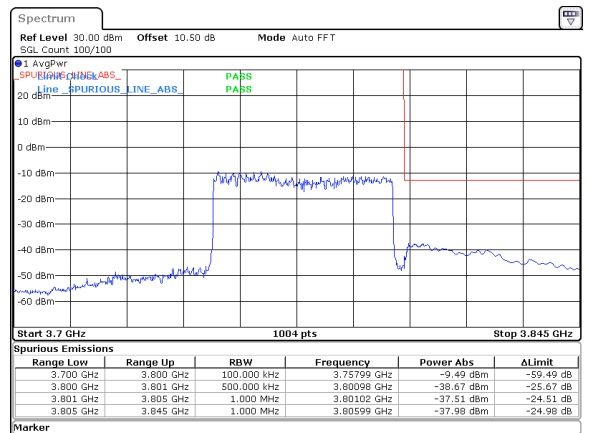
50MHz_30kHz_3775MHz_DFT-s-OFDM QPSK_RB128@0&-37.51 dBm
