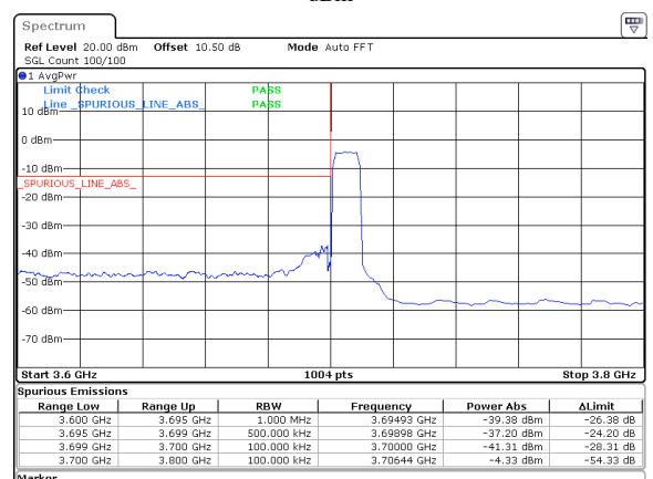
10MHz_30kHz_3705MHz_DFT-s-OFDM QPSK_RB24@0&-37.20 dBm
