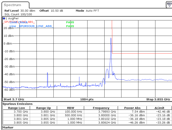
60MHz_30kHz_3770MHz_DFT-s-OFDM QPSK_RB1@161&-36.16 dBm
