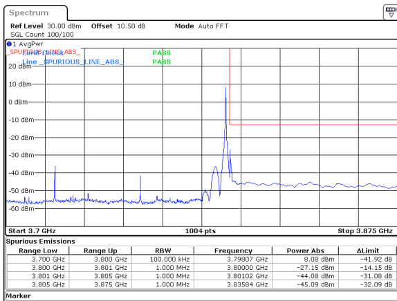
80MHz_30kHz_3760MHz_DFT-s-OFDM QPSK_RB1@216&-27.15 dBm
