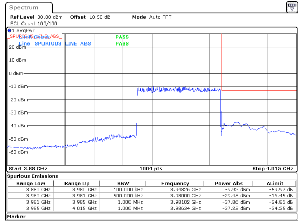
40MHz_15kHz_3960MHz_DFT-s-OFDM QPSK_RB216@0&-29.45 dBm
