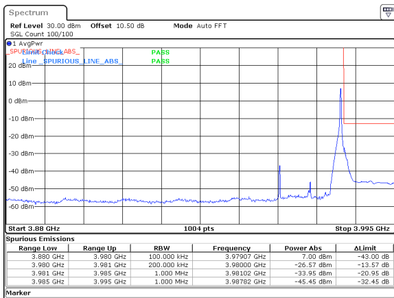
20MHz_30kHz_3970MHz_DFT-s-OFDM QPSK_RB1@50&-26.57 dBm
