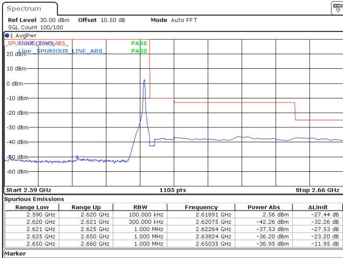
30MHz_30kHz_2605MHz_DFT-s-OFDM QPSK_RB1@77 -36.95 dBm
