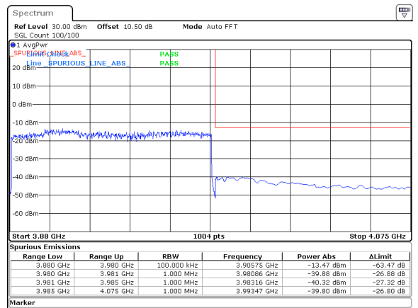
100MHz_30kHz_3930MHz_DFT-s-OFDM QPSK_RB270@0&-39.80 dBm
