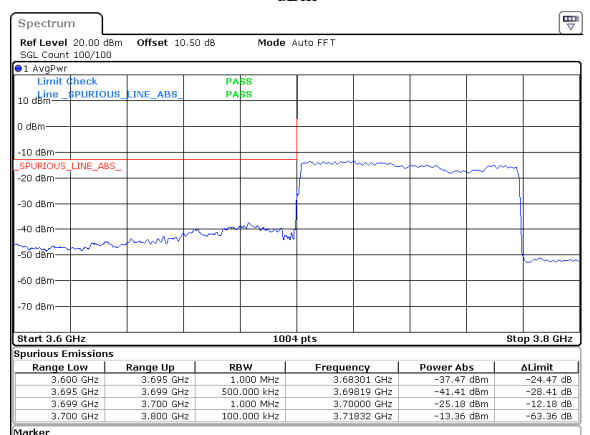
80MHz_30kHz_3740MHz_DFT-s-OFDM QPSK_RB216@0&-25.18 dBm
