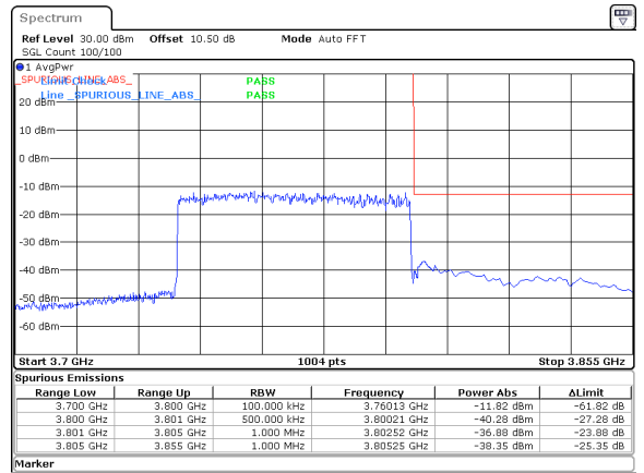
60MHz_30kHz_3770MHz_DFT-s-OFDM QPSK_RB162@0&-36.88 dBm
