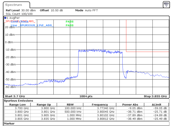
40MHz_30kHz_3780MHz_DFT-s-OFDM QPSK_RB100@0&-37.89 dBm
