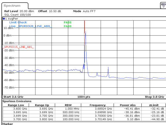
30MHz_30kHz_3715MHz_DFT-s-OFDM QPSK_RB1@0&-36.81 dBm
