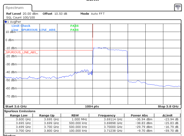
40MHz_15kHz_3720MHz_DFT-s-OFDM QPSK_RB216@0&-29.79 dBm
