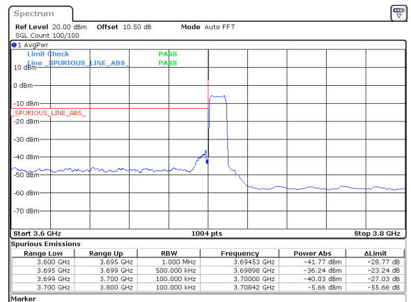
10MHz_15kHz_3705MHz_DFT-s-OFDM QPSK_RB50@0&-36.24 dBm
