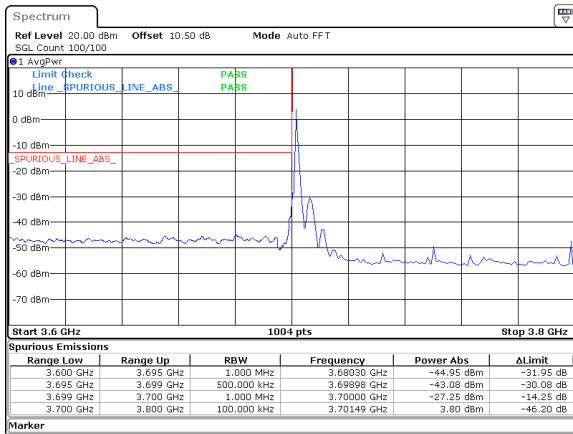
100MHz_30kHz_3750MHz_DFT-s-OFDM QPSK_RB1@0&-27.25 dBm
