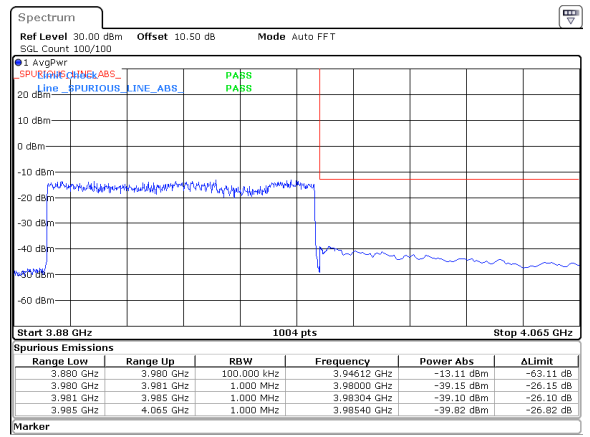
90MHz_30kHz_3935MHz_DFT-s-OFDM QPSK_RB243@0&-39.10 dBm
