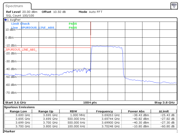
40MHz_30kHz_3720MHz_DFT-s-OFDM QPSK_RB100@0&-38.43 dBm
