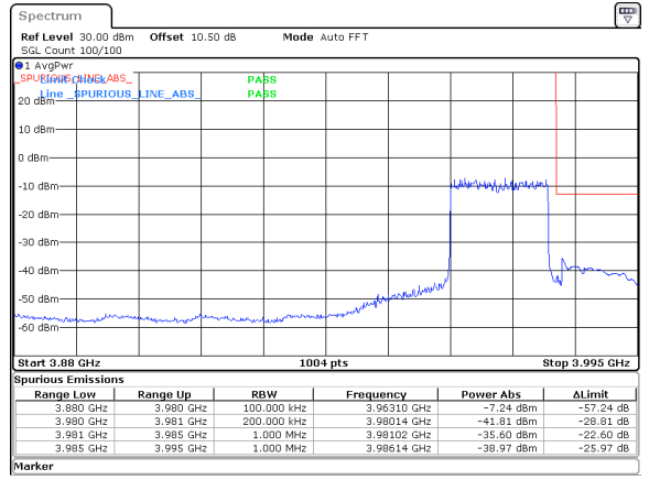
20MHz_15kHz_3970MHz_DFT-s-OFDM QPSK_RB100@0&-35.60 dBm
