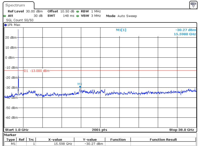
60MHz_30kHz_3770MHz_DFT-s-OFDM QPSK_RB1@0 -30.27 dBm
