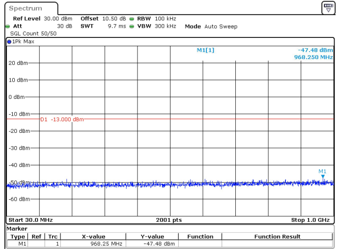
70MHz_30kHz_3735MHz_DFT-s-OFDM QPSK_RB180@0 -47.48 dBm
