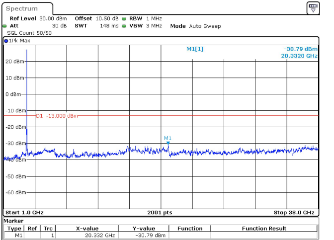
70MHz_30kHz_3750MHz_DFT-s-OFDM QPSK_RB1@0 -30.79 dBm
