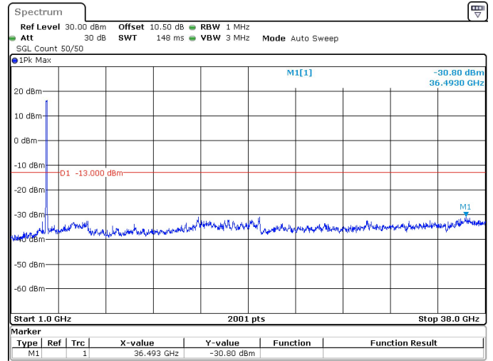
60MHz_30kHz_3770MHz_DFT-s-OFDM QPSK_RB162@0 -30.80 dBm
