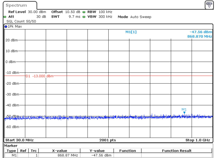
60MHz_30kHz_3750MHz_DFT-s-OFDM QPSK_RB162@0 -47.56 dBm
