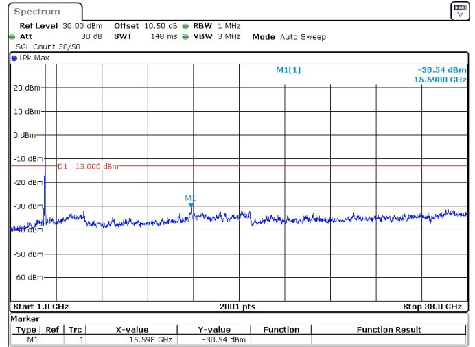
60MHz_30kHz_3770MHz_DFT-s-OFDM QPSK_RB1@161 -30.54 dBm
