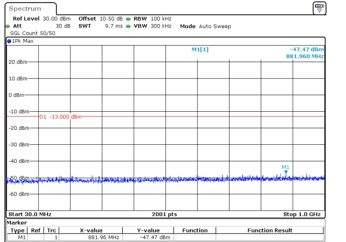
70MHz_30kHz_3750MHz_DFT-s-OFDM QPSK_RB1@0 -47.47 dBm
