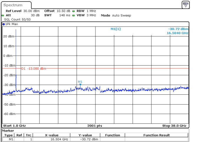
60MHz_30kHz_3750MHz_DFT-s-OFDM QPSK_RB1@0 -30.72 dBm
