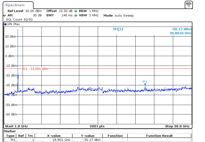
50MHz_30kHz_3775MHz_DFT-s-OFDM QPSK_RB1@0 -30.17 dBm
