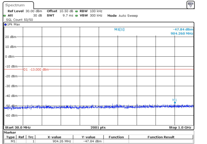
60MHz_30kHz_3750MHz_DFT-s-OFDM QPSK_RB1@0 -47.84 dBm
