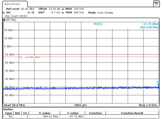
60MHz_30kHz_3730MHz_DFT-s-OFDM QPSK_RB162@0 -47.75 dBm
