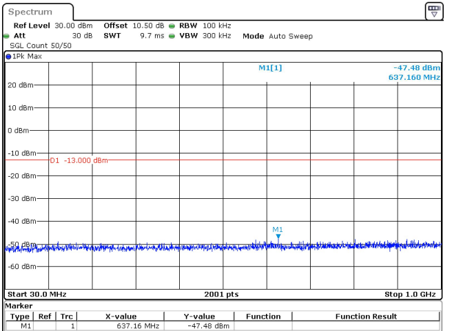
50MHz_30kHz_3775MHz_DFT-s-OFDM QPSK_RB1@0 -47.48 dBm
