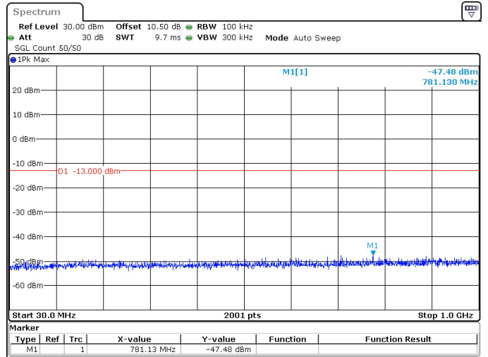
50MHz_30kHz_3750MHz_DFT-s-OFDM QPSK_RB128@0 -47.48 dBm
