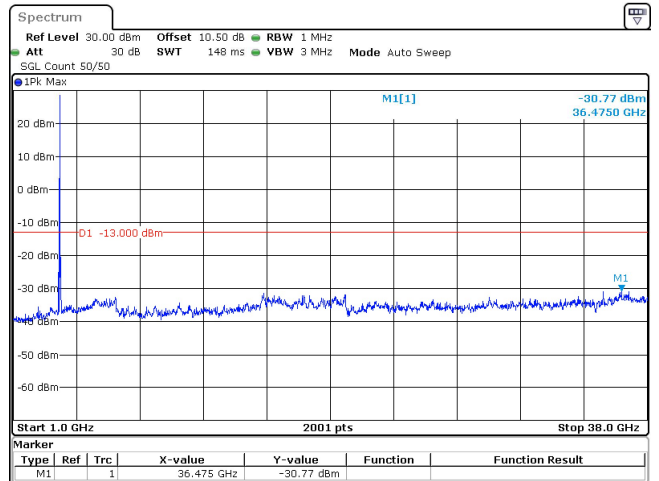
60MHz_30kHz_3730MHz_DFT-s-OFDM QPSK_RB1@0 -30.77 dBm
