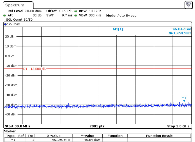
50MHz_30kHz_3750MHz_DFT-s-OFDM QPSK_RB1@0 -46.84 dBm
