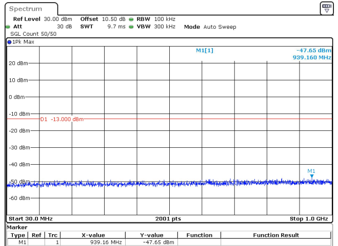
50MHz_30kHz_3725MHz_DFT-s-OFDM QPSK_RB1@0 -47.65 dBm
