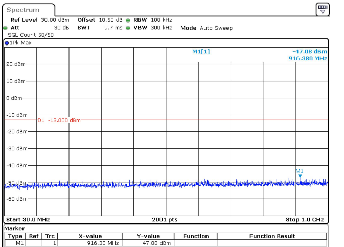
50MHz_15kHz_3775MHz_DFT-s-OFDM QPSK_RB1@0 -47.08 dBm
