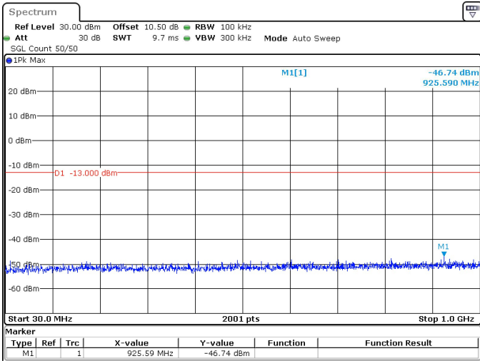
25MHz_30kHz_3750MHz_DFT-s-OFDM QPSK_RB1@64 -46.74 dBm
