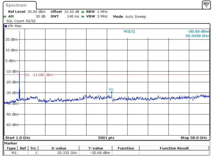
25MHz_30kHz_3750MHz_DFT-s-OFDM QPSK_RB1@64 -30.68 dBm
