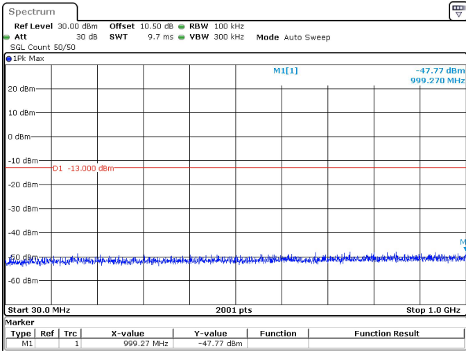
25MHz_30kHz_3787.5MHz_DFT-s-OFDM QPSK_RB1@64 -47.77 dBm
