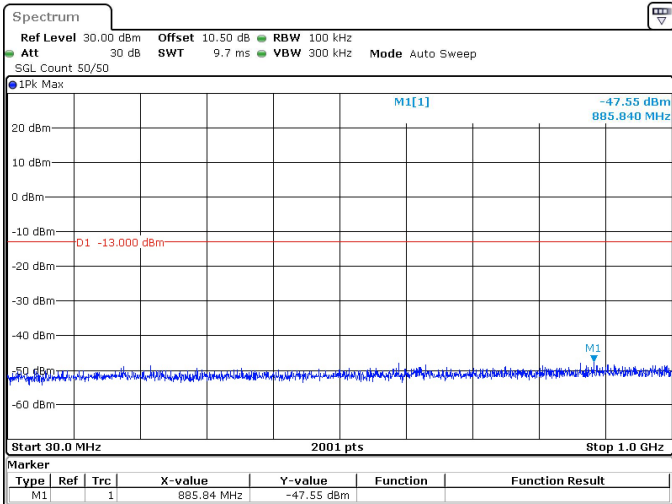
25MHz_30kHz_3750MHz_DFT-s-OFDM QPSK_RB64@0 -47.55 dBm
