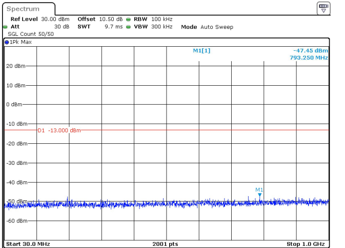
30MHz_15kHz_3750MHz_DFT-s-OFDM QPSK_RB1@0 -47.45 dBm
