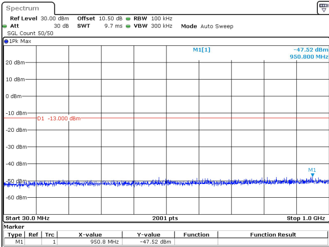
25MHz_30kHz_3787.5MHz_DFT-s-OFDM QPSK_RB64@0 -47.52 dBm
