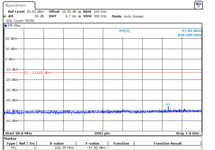
25MHz_30kHz_3750MHz_DFT-s-OFDM QPSK_RB1@0 -47.80 dBm
