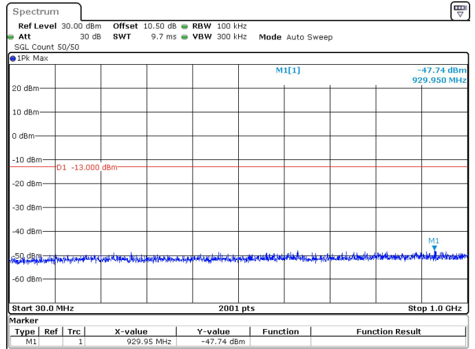
25MHz_30kHz_3712.5MHz_DFT-s-OFDM QPSK_RB64@0 -47.74 dBm
