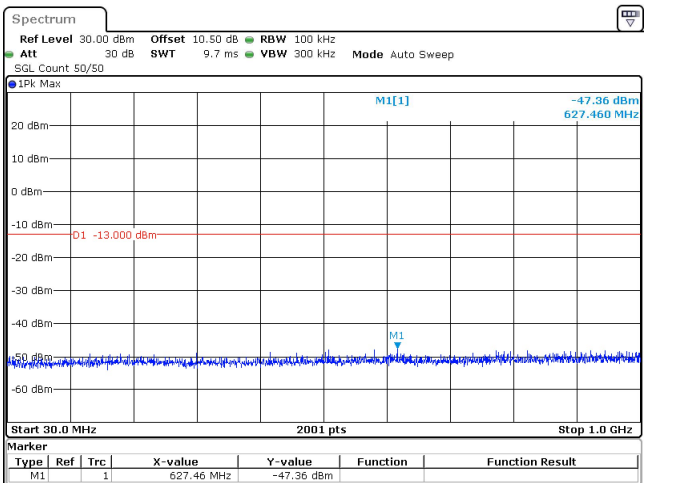
25MHz_30kHz_3712.5MHz_DFT-s-OFDM QPSK_RB1@0 -47.36 dBm
