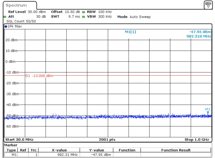
25MHz_30kHz_3712.5MHz_DFT-s-OFDM QPSK_RB1@64 -47.95 dBm
