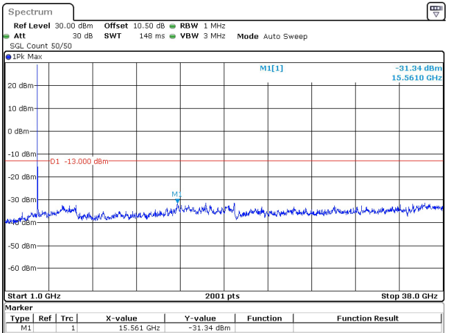
25MHz_30kHz_3750MHz_DFT-s-OFDM QPSK_RB1@0 -31.34 dBm
