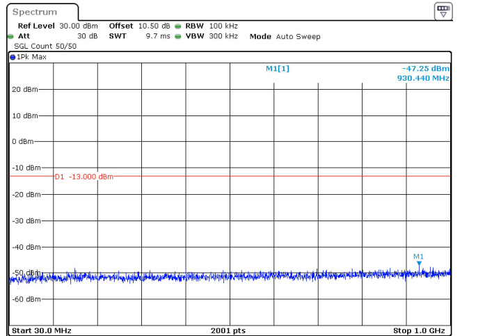
25MHz_15kHz_3750MHz_DFT-s-OFDM QPSK_RB1@0 -47.25 dBm
