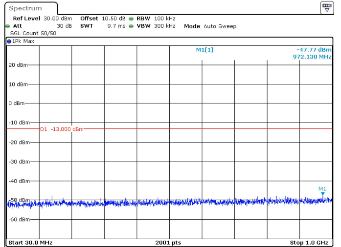
25MHz_15kHz_3712.5MHz_DFT-s-OFDM QPSK_RB128@0 -47.77 dBm
