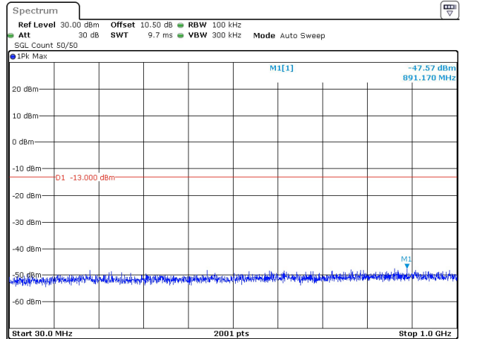
25MHz_15kHz_3712.5MHz_DFT-s-OFDM QPSK_RB1@0 -47.57 dBm
