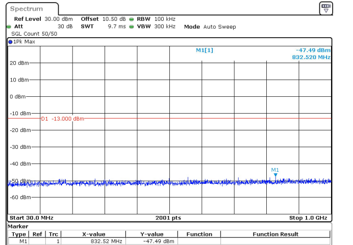
15MHz_30kHz_3750MHz_DFT-s-OFDM QPSK_RB1@0 -47.49 dBm
