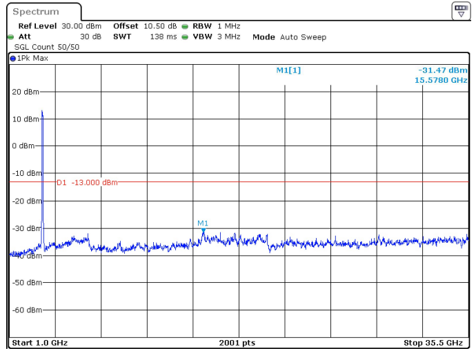
70MHz_30kHz_3500MHz_DFT-s-OFDM QPSK_RB180@0 -31.47 dBm
