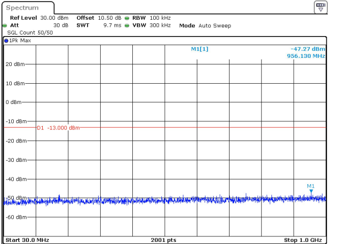
70MHz_30kHz_3515MHz_DFT-s-OFDM QPSK_RB1@0 -47.27 dBm
