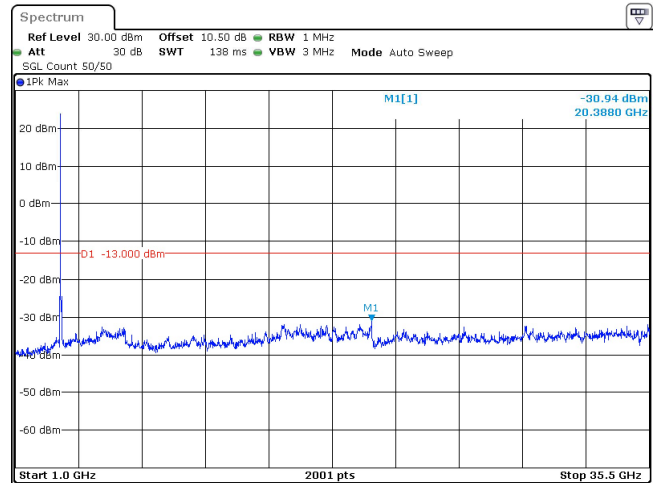
70MHz_30kHz_3485MHz_DFT-s-OFDM QPSK_RB1@0 -30.94 dBm
