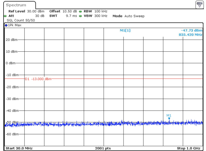
60MHz_30kHz_3520MHz_DFT-s-OFDM QPSK_RB162@0 -47.73 dBm
