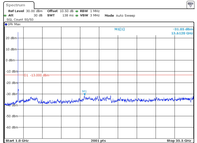
70MHz_30kHz_3500MHz_DFT-s-OFDM QPSK_RB1@0 -31.05 dBm
