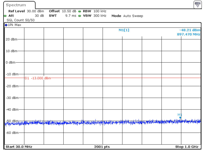
70MHz_30kHz_3485MHz_DFT-s-OFDM QPSK_RB1@188 -48.21 dBm
