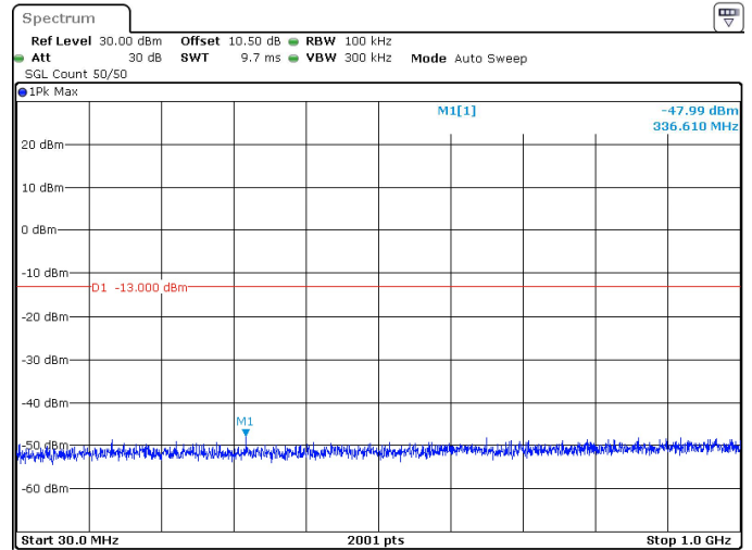
70MHz_30kHz_3485MHz_DFT-s-OFDM QPSK_RB180@0 -47.99 dBm
