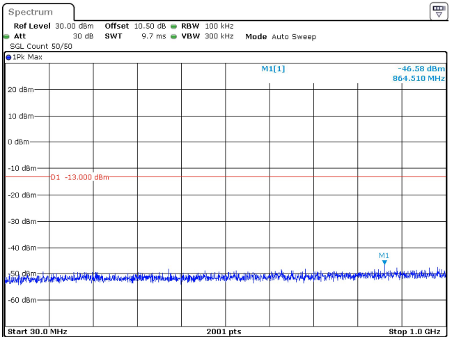
70MHz_30kHz_3500MHz_DFT-s-OFDM QPSK_RB1@0 -46.58 dBm
