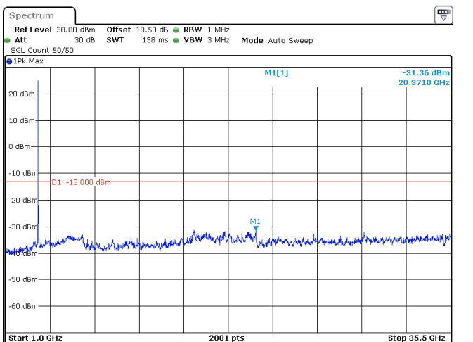
60MHz_30kHz_3520MHz_DFT-s-OFDM QPSK_RB1@0 -31.36 dBm
