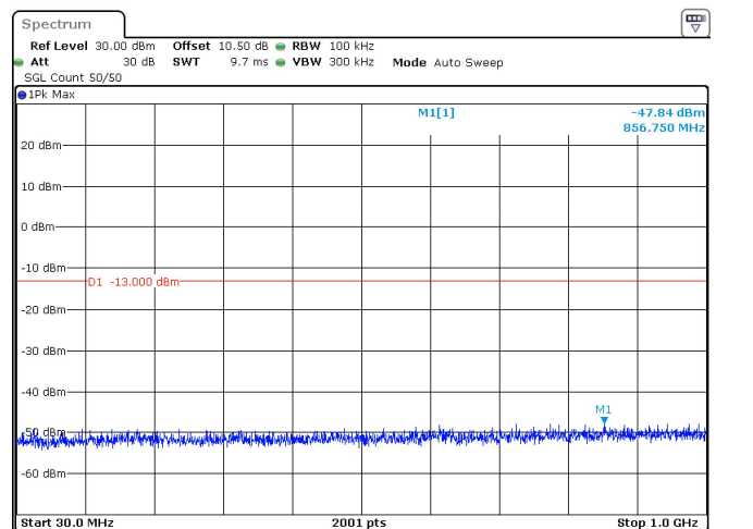
60MHz_30kHz_3520MHz_DFT-s-OFDM QPSK_RB1@0 -47.84 dBm
