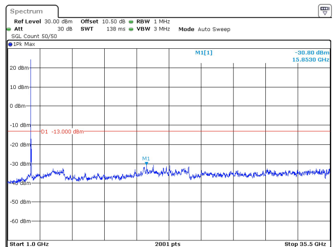
60MHz_30kHz_3500MHz_DFT-s-OFDM QPSK_RB1@0 -30.80 dBm
