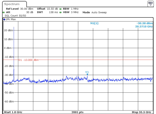
60MHz_30kHz_3480MHz_DFT-s-OFDM QPSK_RB1@0 -30.38 dBm
