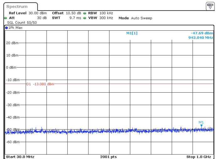
60MHz_30kHz_3500MHz_DFT-s-OFDM QPSK_RB162@0 -47.69 dBm
