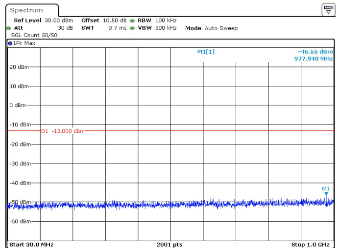
60MHz_30kHz_3480MHz_DFT-s-OFDM QPSK_RB162@0 -46.55 dBm
