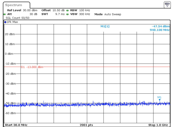
50MHz_30kHz_3475MHz_DFT-s-OFDM QPSK_RB1@0 -47.54 dBm
