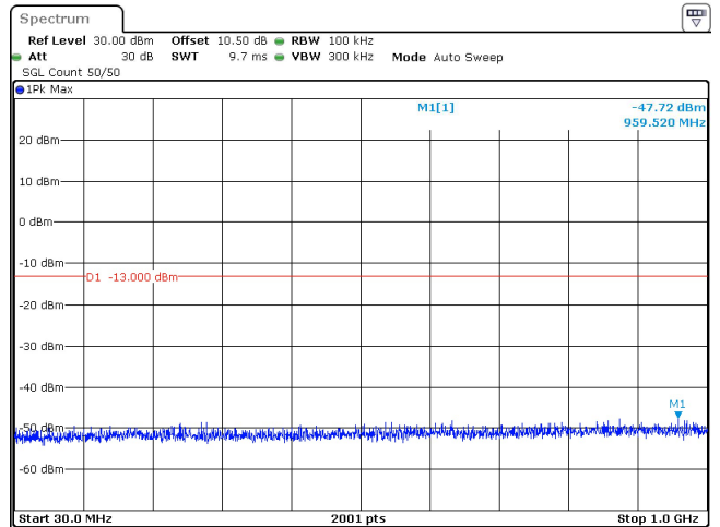
50MHz_30kHz_3500MHz_DFT-s-OFDM QPSK_RB1@0 -47.72 dBm
