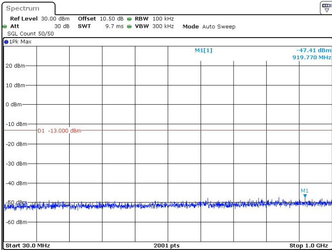
40MHz_30kHz_3530MHz_DFT-s-OFDM QPSK_RB100@0 -47.41 dBm
