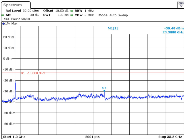
50MHz_30kHz_3500MHz_DFT-s-OFDM QPSK_RB1@0 -30.48 dBm
