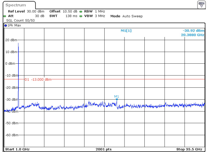
40MHz_30kHz_3470MHz_DFT-s-OFDM QPSK_RB100@0 -30.92 dBm
