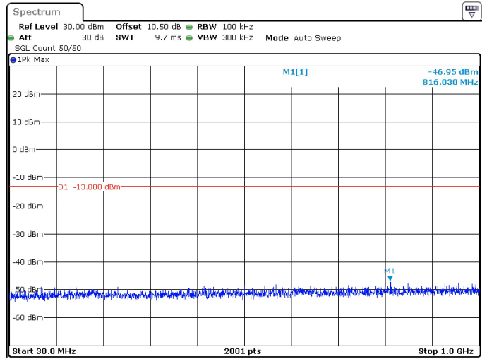
30MHz_30kHz_3535MHz_DFT-s-OFDM QPSK_RB1@77 -46.95 dBm
