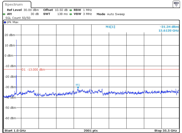
30MHz_30kHz_3535MHz_DFT-s-OFDM QPSK_RB75@0 -31.34 dBm
