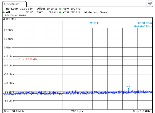
40MHz_30kHz_3500MHz_DFT-s-OFDM QPSK_RB1@0 -47.58 dBm
