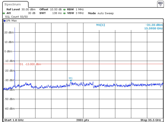
40MHz_30kHz_3470MHz_DFT-s-OFDM QPSK_RB1@0 -31.35 dBm
