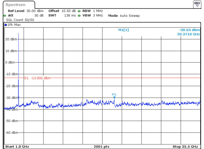
25MHz_30kHz_3537.5MHz_DFT-s-OFDM QPSK_RB1@0 -30.65 dBm
