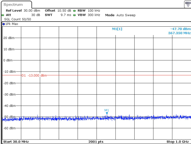
25MHz_30kHz_3537.5MHz_DFT-s-OFDM QPSK_RB1@0 -47.70 dBm
