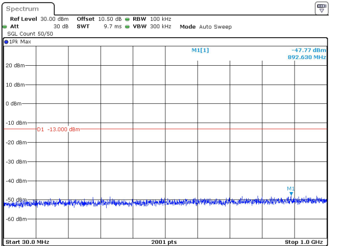
25MHz_30kHz_3500MHz_DFT-s-OFDM QPSK_RB1@0 -47.77 dBm
