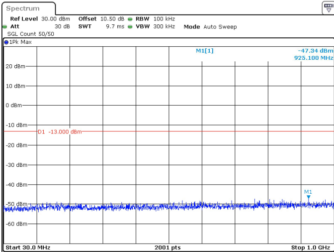
25MHz_30kHz_3500MHz_DFT-s-OFDM QPSK_RB64@0 -47.34 dBm
