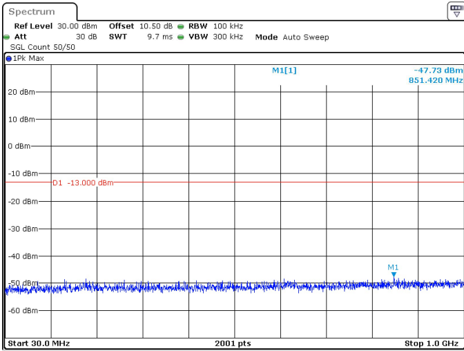
25MHz_30kHz_3500MHz_DFT-s-OFDM QPSK_RB1@64 -47.73 dBm
