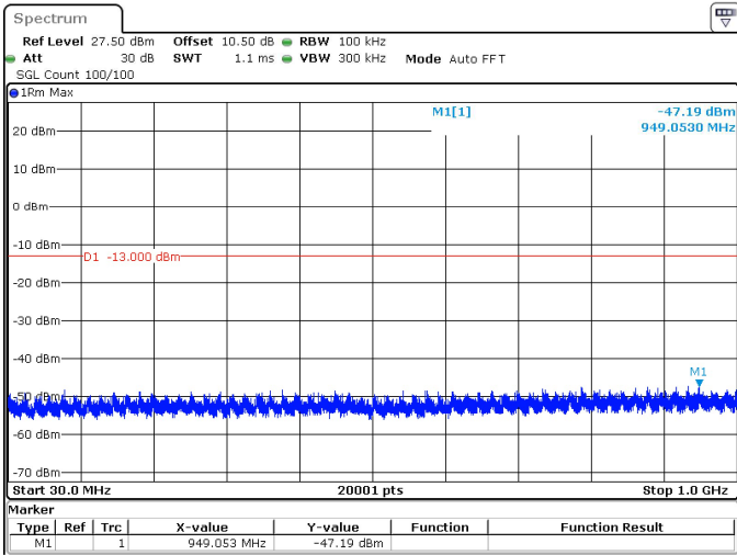
60MHz_30kHz_3840MHz_DFT-s-OFDM QPSK_RB1@0 -47.19 dBm
