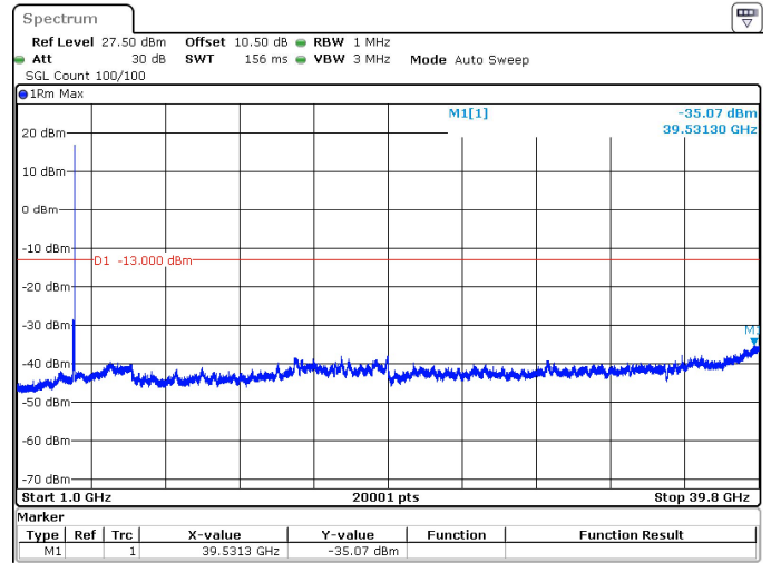
60MHz_30kHz_3950MHz_DFT-s-OFDM QPSK_RB1@161 -35.07 dBm
