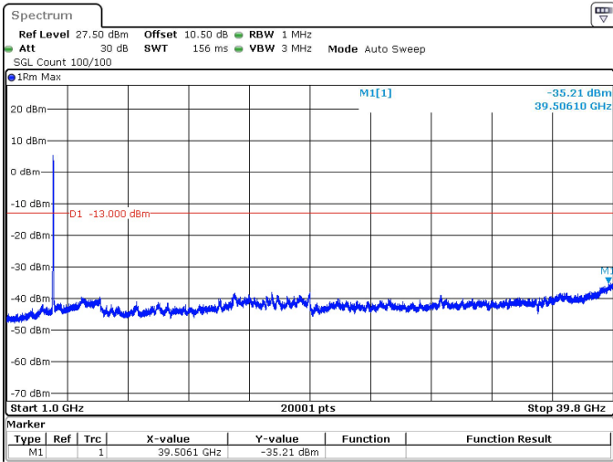
50MHz_30kHz_3955MHz_DFT-s-OFDM QPSK_RB128@0 -35.21 dBm
