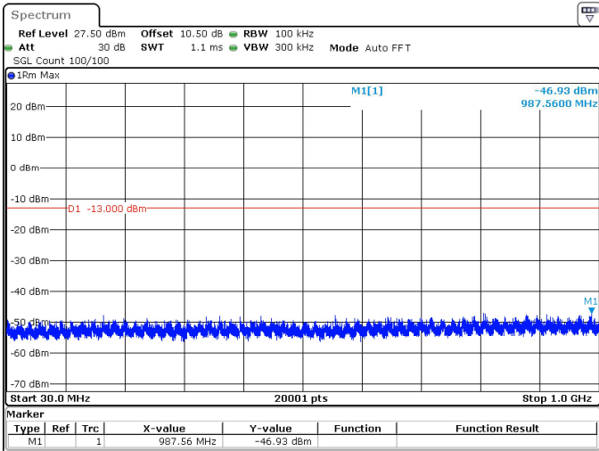
60MHz_30kHz_3950MHz_DFT-s-OFDM QPSK_RB1@0 -46.93 dBm
