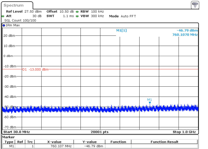
60MHz_30kHz_3950MHz_DFT-s-OFDM QPSK_RB1@161 -46.79 dBm
