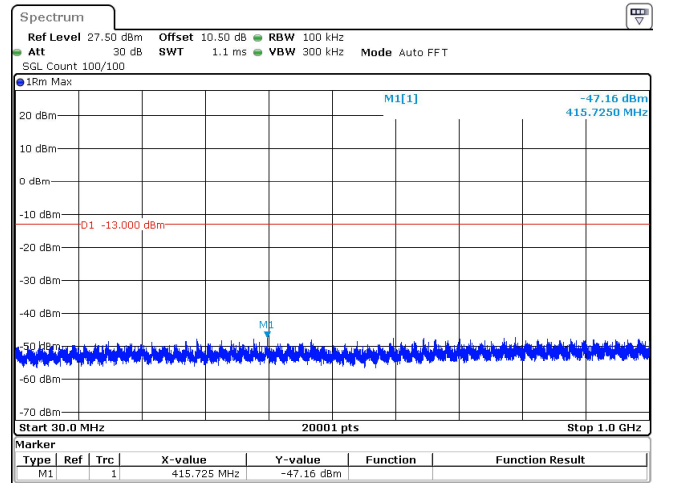
60MHz_30kHz_3950MHz_DFT-s-OFDM QPSK_RB162@0 -47.16 dBm
