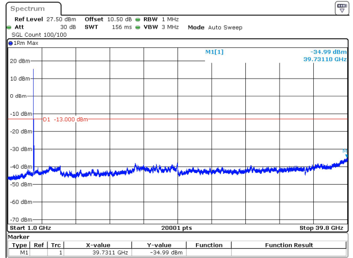
60MHz_30kHz_3950MHz_DFT-s-OFDM QPSK_RB1@0 -34.99 dBm
