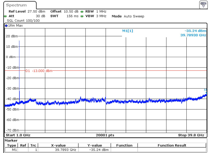
60MHz_30kHz_3840MHz_DFT-s-OFDM QPSK_RB1@0 -35.24 dBm
