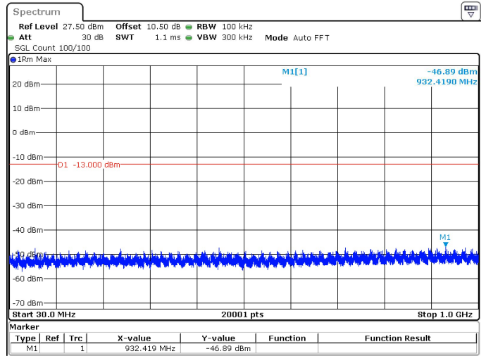
60MHz_30kHz_3730MHz_DFT-s-OFDM QPSK_RB1@0 -46.89 dBm
