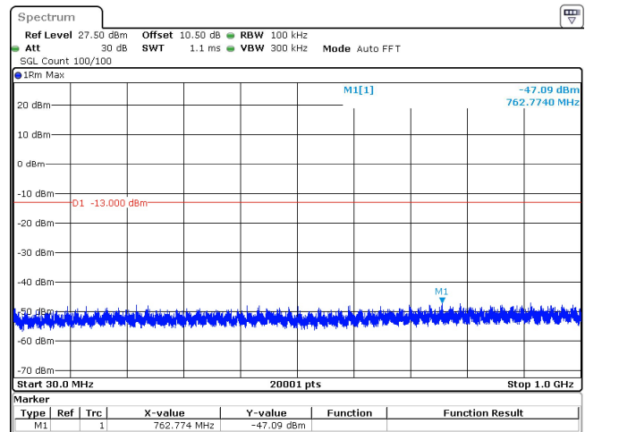
50MHz_15kHz_3725MHz_DFT-s-OFDM QPSK_RB270@0 -47.09 dBm
