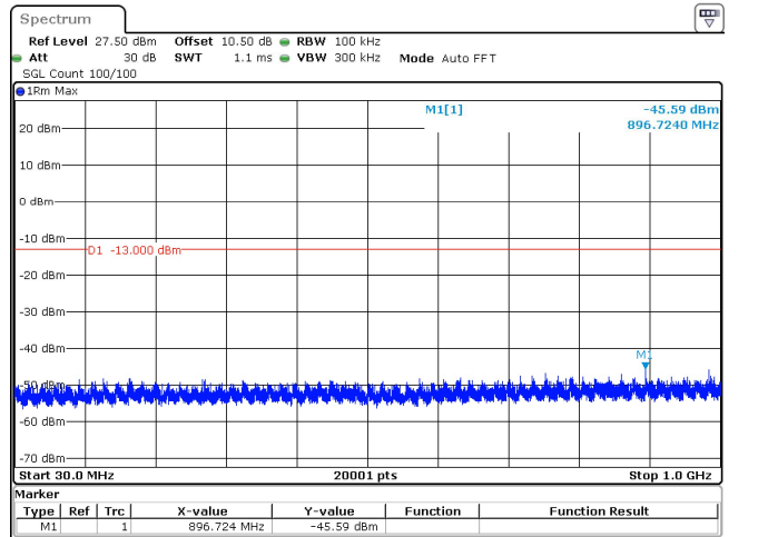
50MHz_15kHz_3955MHz_DFT-s-OFDM QPSK_RB270@0 -45.59 dBm
