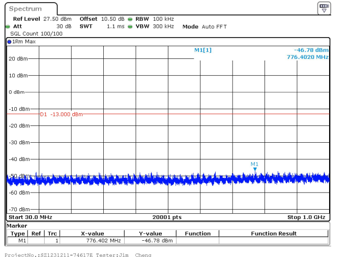
40MHz_15kHz_3960MHz_DFT-s-OFDM QPSK_RB216@0 -46.78 dBm
