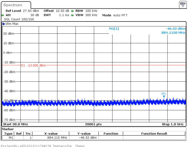
40MHz_15kHz_3960MHz_DFT-s-OFDM QPSK_RB1@215 -46.52 dBm
