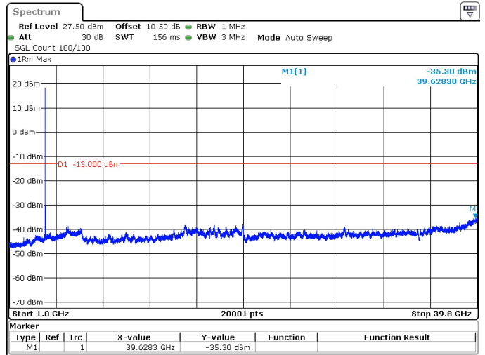
30MHz_15kHz_3965MHz_DFT-s-OFDM QPSK_RB1@0 -35.30 dBm
