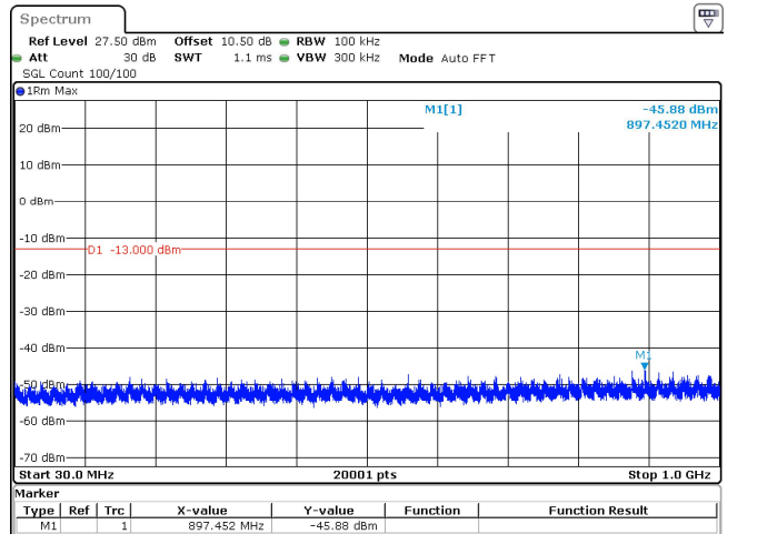
30MHz_15kHz_3965MHz_DFT-s-OFDM QPSK_RB160@0 -45.88 dBm
