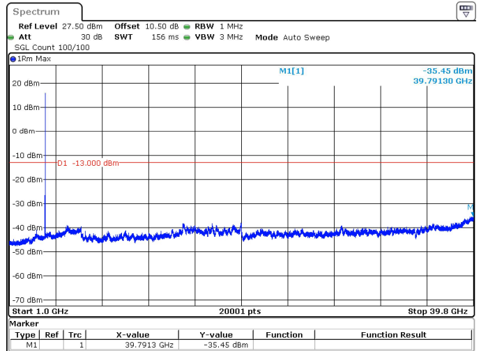
30MHz_15kHz_3965MHz_DFT-s-OFDM QPSK_RB1@159 -35.45 dBm
