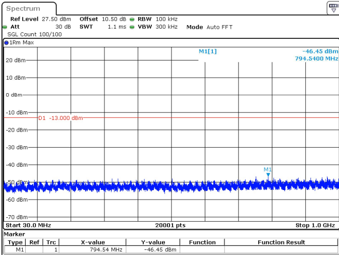
20MHz_30kHz_3970MHz_DFT-s-OFDM QPSK_RB1@0 -46.45 dBm
