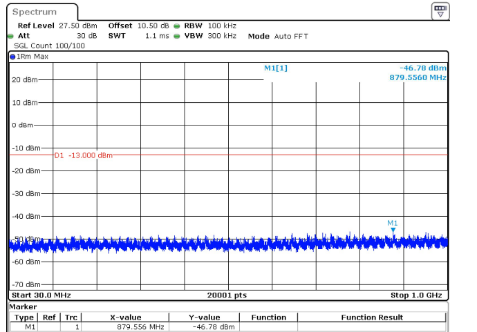
20MHz_30kHz_3840MHz_DFT-s-OFDM QPSK_RB50@0 -46.78 dBm
