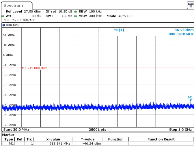
20MHz_30kHz_3710MHz_DFT-s-OFDM QPSK_RB1@0 -46.24 dBm
