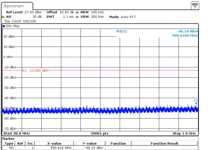
20MHz_30kHz_3710MHz_DFT-s-OFDM QPSK_RB1@50 -46.19 dBm
