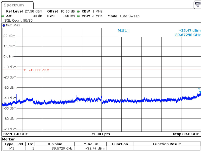
20MHz_30kHz_3840MHz_DFT-s-OFDM QPSK_RB1@0 -35.47 dBm
