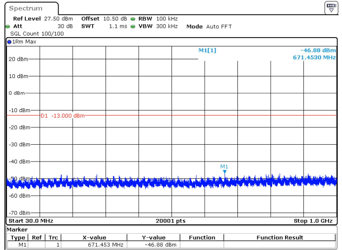
20MHz_30kHz_3840MHz_DFT-s-OFDM QPSK_RB1@0 -46.88 dBm
