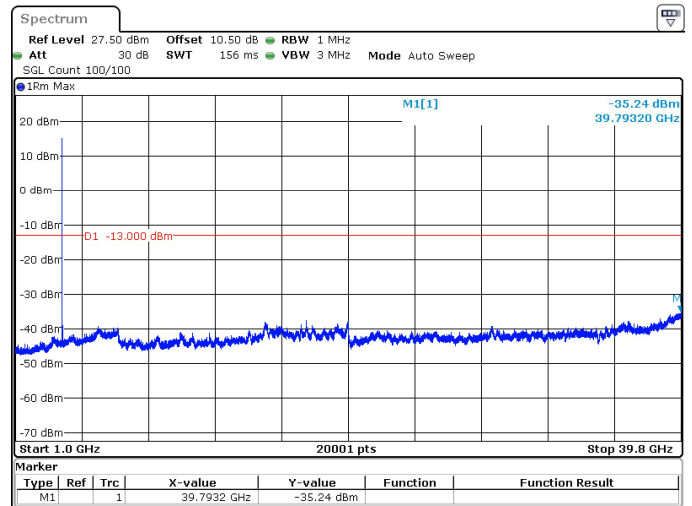
20MHz_30kHz_3710MHz_DFT-s-OFDM QPSK_RB1@50 -35.24 dBm
