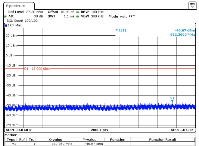
20MHz_30kHz_3710MHz_DFT-s-OFDM QPSK_RB50@0 -46.67 dBm
