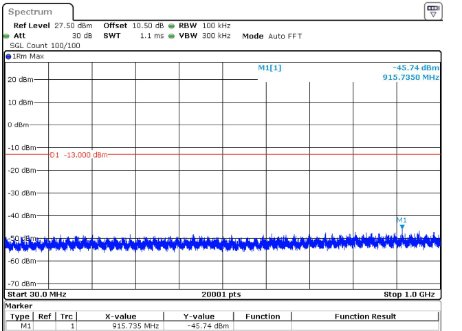
20MHz_30kHz_3840MHz_DFT-s-OFDM QPSK_RB1@50 -45.74 dBm
