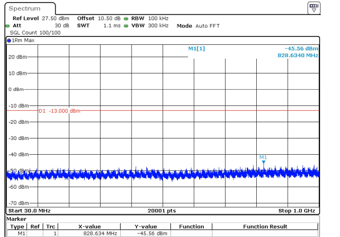
20MHz_30kHz_3970MHz_DFT-s-OFDM QPSK_RB50@0 -45.56 dBm
