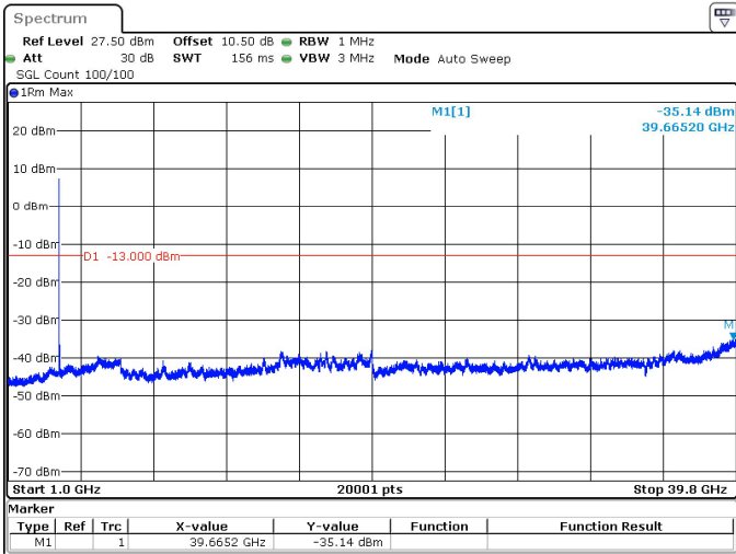
20MHz_30kHz_3710MHz_DFT-s-OFDM QPSK_RB50@0 -35.14 dBm
