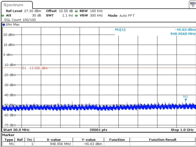
20MHz_15kHz_3970MHz_DFT-s-OFDM QPSK_RB100@0 -45.63 dBm
