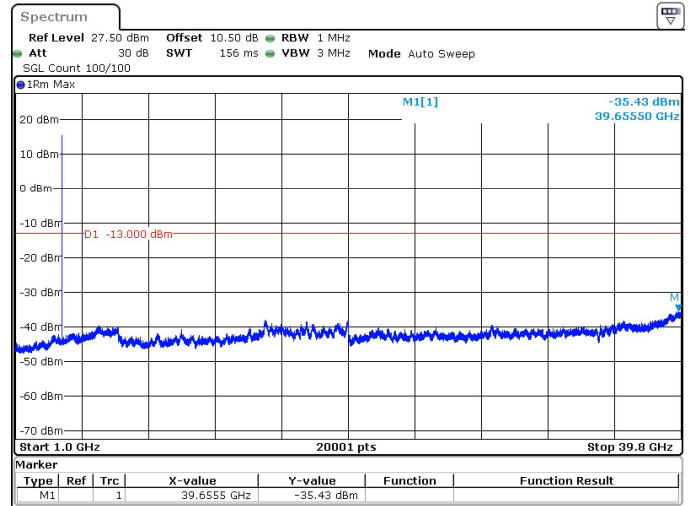
20MHz_30kHz_3710MHz_DFT-s-OFDM QPSK_RB1@0 -35.43 dBm
