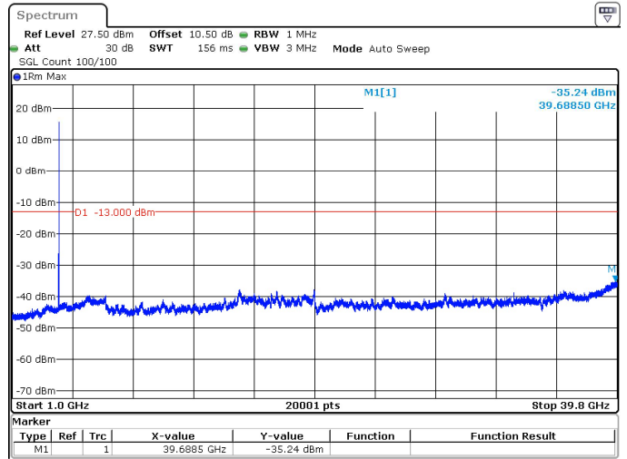
20MHz_30kHz_3970MHz_DFT-s-OFDM QPSK_RB1@50 -35.24 dBm
