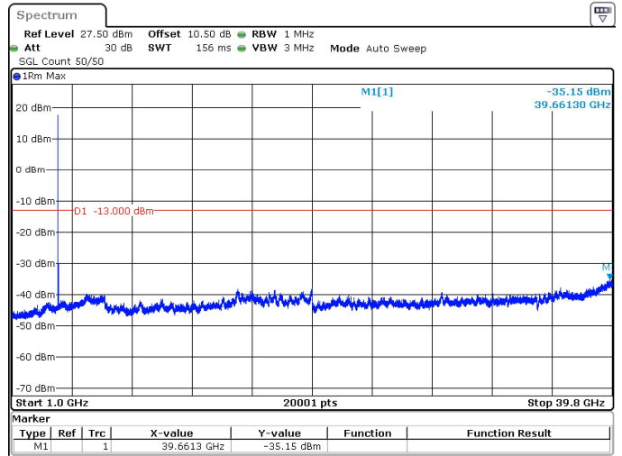
20MHz_30kHz_3970MHz_DFT-s-OFDM QPSK_RB1@0 -35.15 dBm
