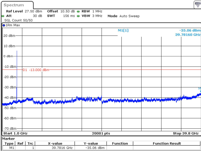
20MHz_30kHz_3840MHz_DFT-s-OFDM QPSK_RB50@0 -35.06 dBm
