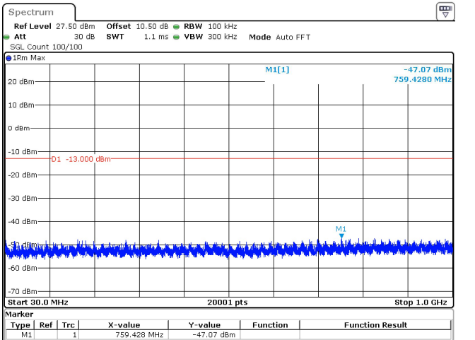
20MHz_30kHz_3970MHz_DFT-s-OFDM QPSK_RB1@50 -47.07 dBm
