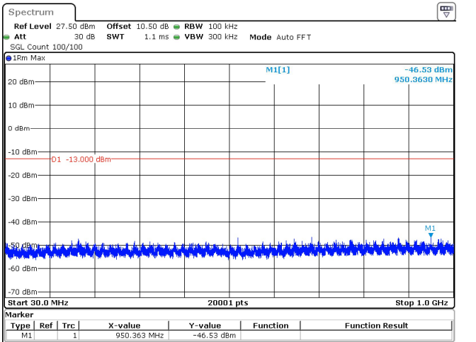
20MHz_15kHz_3970MHz_DFT-s-OFDM QPSK_RB1@105 -46.53 dBm
