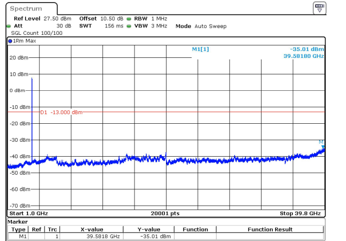
20MHz_15kHz_3970MHz_DFT-s-OFDM QPSK_RB100@0 -35.01 dBm
