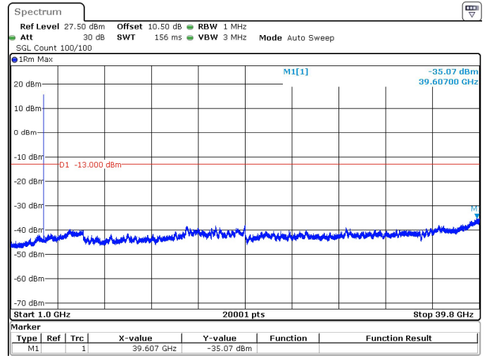
20MHz_15kHz_3710MHz_DFT-s-OFDM QPSK_RB1@105 -35.07 dBm
