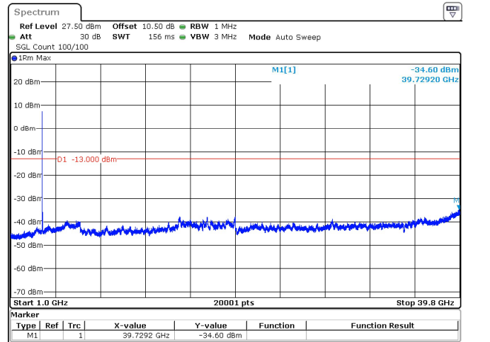
20MHz_15kHz_3710MHz_DFT-s-OFDM QPSK_RB100@0 -34.60 dBm
