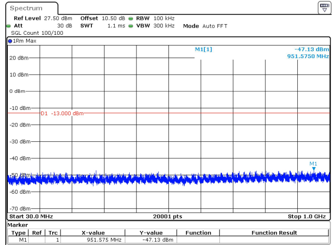
20MHz_15kHz_3710MHz_DFT-s-OFDM QPSK_RB1@0 -47.13 dBm
