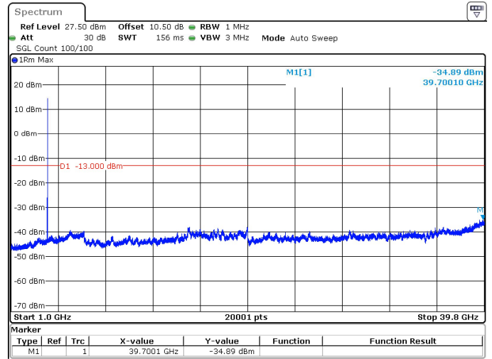
20MHz_15kHz_3970MHz_DFT-s-OFDM QPSK_RB1@105 -34.89 dBm
