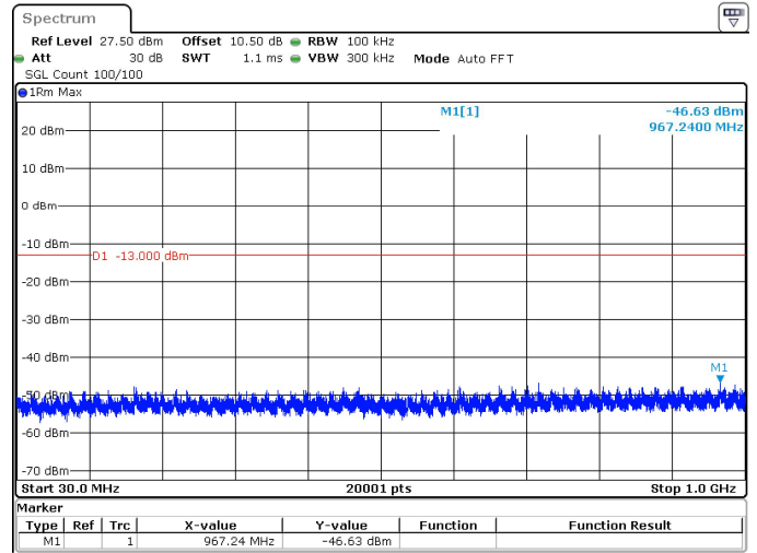
20MHz_15kHz_3970MHz_DFT-s-OFDM QPSK_RB1@0 -46.63 dBm
