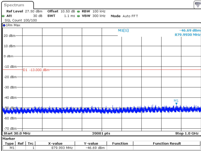
10MHz_30kHz_3975MHz_DFT-s-OFDM QPSK_RB24@0 -46.69 dBm
