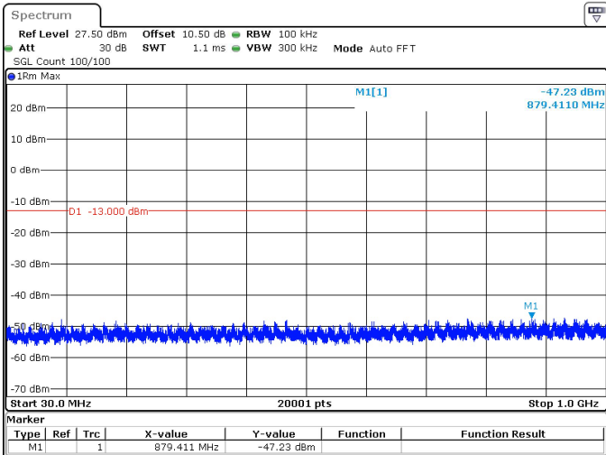
15MHz_15kHz_3972.5MHz_DFT-s-OFDM QPSK_RB1@0 -47.23 dBm
