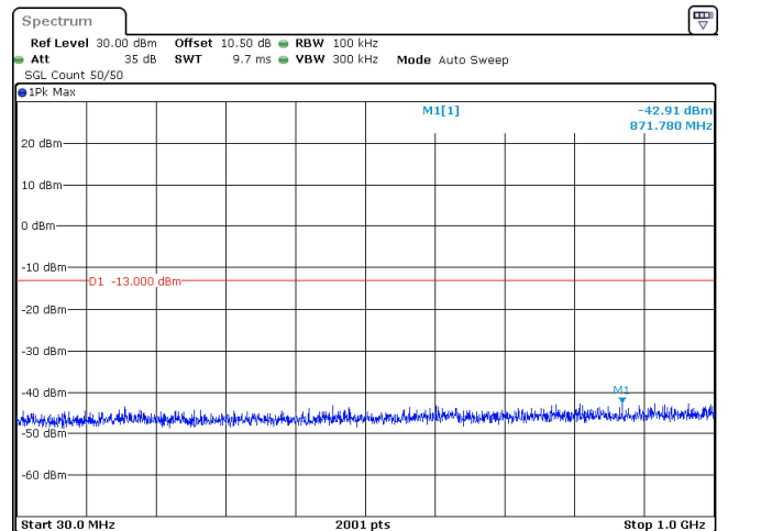
90MHz_30kHz_3500MHz_DFT-s-OFDM QPSK_RB243@0 -42.91 dBm
