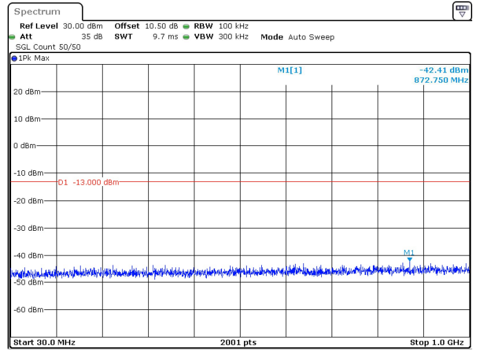
90MHz_30kHz_3505MHz_DFT-s-OFDM QPSK_RB1@0 -42.41 dBm
