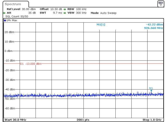
100MHz_30kHz_3500MHz_DFT-s-OFDM QPSK_RB1@272 -42.22 dBm
