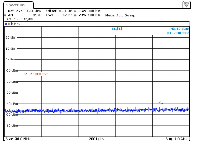
100MHz_30kHz_3500MHz_DFT-s-OFDM QPSK_RB270@0 -42.40 dBm
