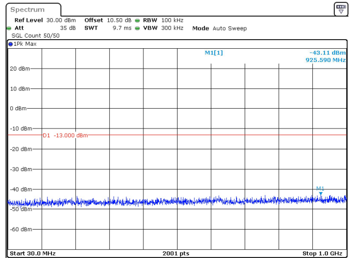
90MHz_30kHz_3500MHz_DFT-s-OFDM QPSK_RB1@0 -43.11 dBm
