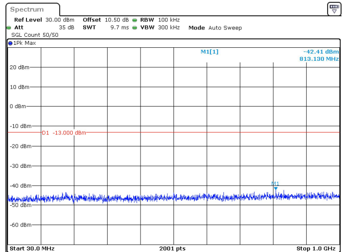
90MHz_30kHz_3500MHz_DFT-s-OFDM QPSK_RB1@244 -42.41 dBm
