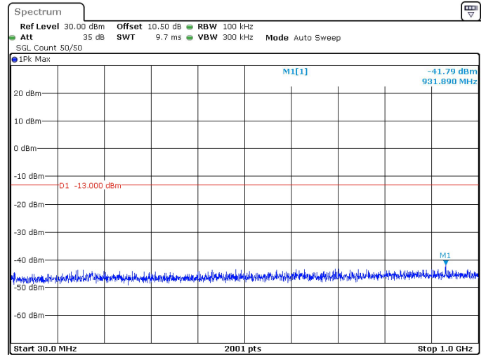
60MHz_30kHz_3480MHz_DFT-s-OFDM QPSK_RB1@161 -41.79 dBm
