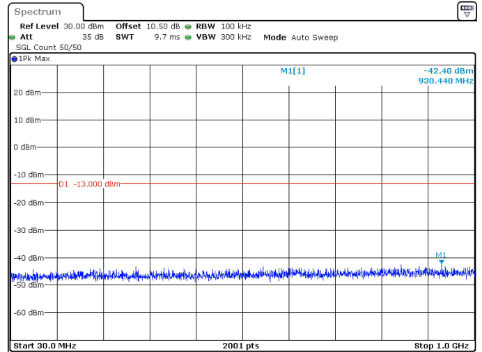
50MHz_30kHz_3500MHz_DFT-s-OFDM QPSK_RB1@0 -42.40 dBm
