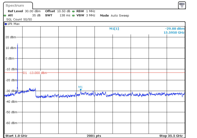
40MHz_30kHz_3530MHz_DFT-s-OFDM QPSK_RB100@0 -29.88 dBm
