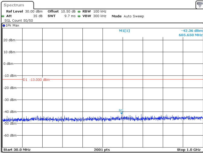
40MHz_30kHz_3530MHz_DFT-s-OFDM QPSK_RB100@0 -42.36 dBm
