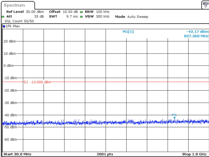
40MHz_30kHz_3530MHz_DFT-s-OFDM QPSK_RB1@0 -43.17 dBm
