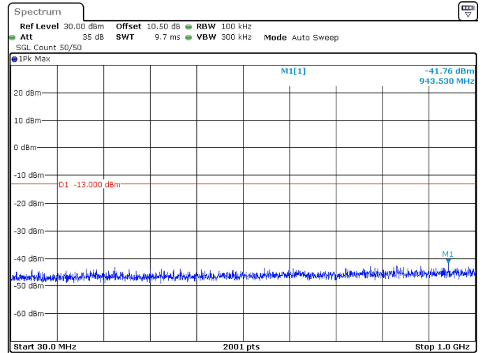
40MHz_30kHz_3500MHz_DFT-s-OFDM QPSK_RB1@0 -41.76 dBm
