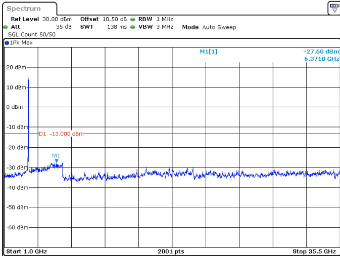
40MHz_15kHz_3470MHz_DFT-s-OFDM QPSK_RB216@0 -27.60 dBm
