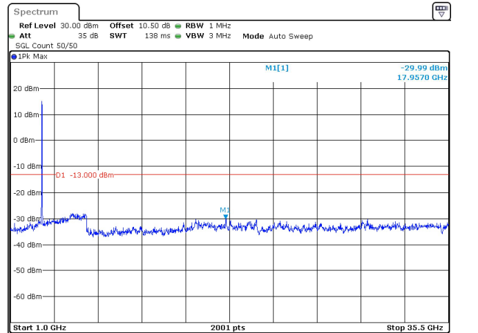
40MHz_30kHz_3470MHz_DFT-s-OFDM QPSK_RB100@0 -29.99 dBm
