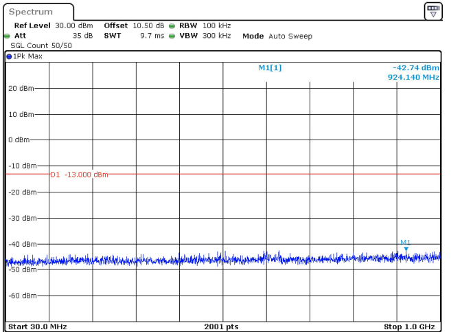
40MHz_30kHz_3470MHz_DFT-s-OFDM QPSK_RB1@105 -42.74 dBm
