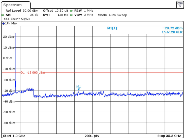
40MHz_15kHz_3530MHz_DFT-s-OFDM QPSK_RB1@215 -29.72 dBm
