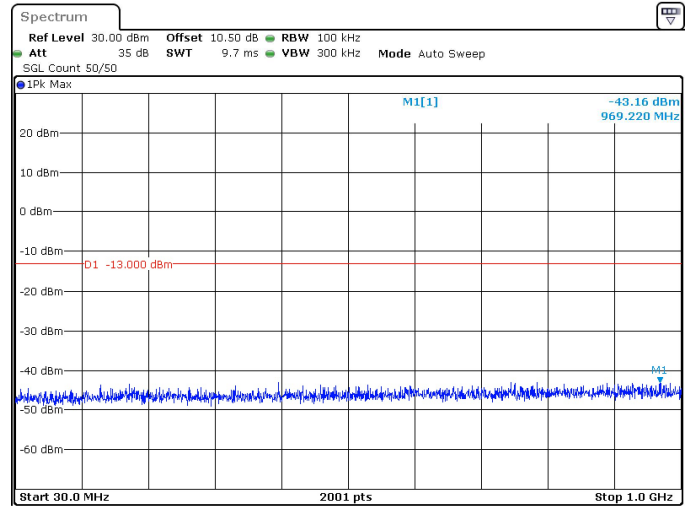
40MHz_15kHz_3530MHz_DFT-s-OFDM QPSK_RB1@215 -43.16 dBm
