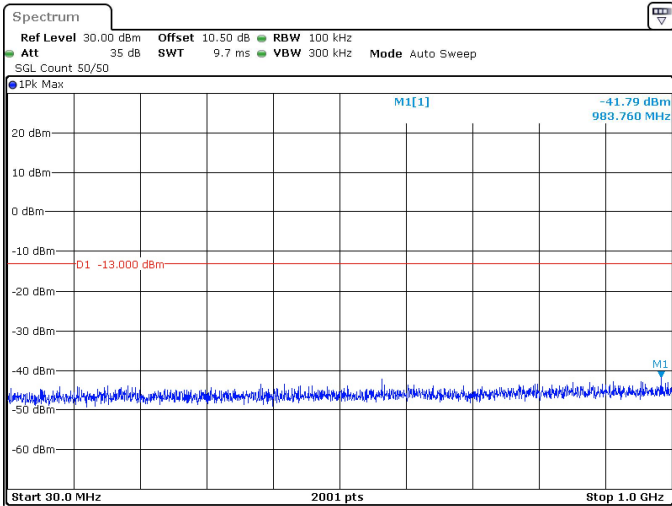
40MHz_15kHz_3470MHz_DFT-s-OFDM QPSK_RB1@0 -41.79 dBm
