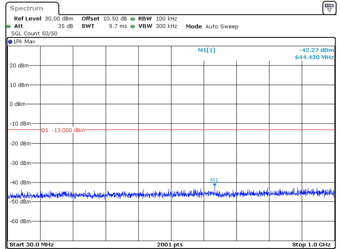
40MHz_15kHz_3470MHz_DFT-s-OFDM QPSK_RB1@215 -42.27 dBm
