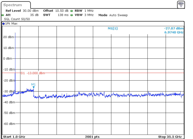
40MHz_15kHz_3470MHz_DFT-s-OFDM QPSK_RB1@215 -27.07 dBm
