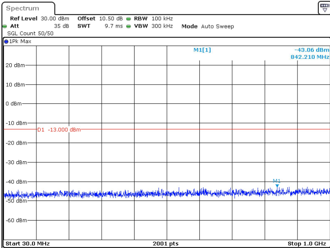
30MHz_15kHz_3535MHz_DFT-s-OFDM QPSK_RB1@0 -43.06 dBm
