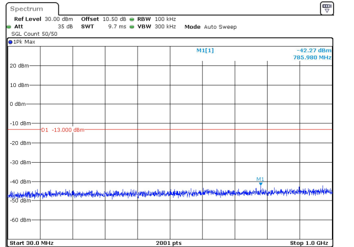
40MHz_15kHz_3470MHz_DFT-s-OFDM QPSK_RB216@0 -42.27 dBm
