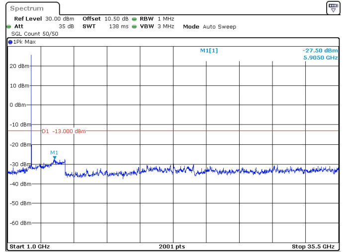
40MHz_15kHz_3470MHz_DFT-s-OFDM QPSK_RB1@0 -27.50 dBm
