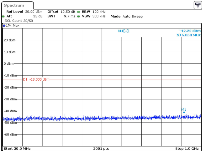
20MHz_30kHz_3460MHz_DFT-s-OFDM QPSK_RB1@50 -42.22 dBm
