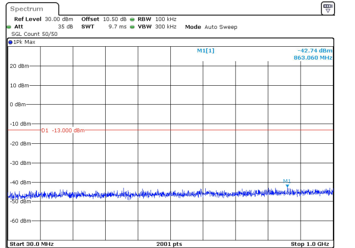
20MHz_15kHz_3500MHz_DFT-s-OFDM QPSK_RB100@0 -42.74 dBm
