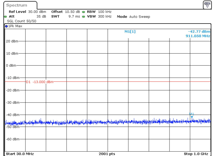
20MHz_15kHz_3500MHz_DFT-s-OFDM QPSK_RB1@105 -42.77 dBm
