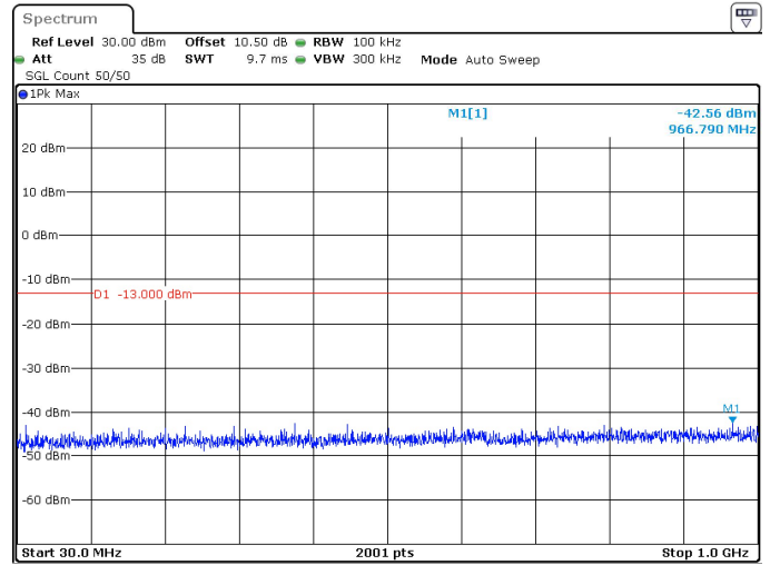
20MHz_30kHz_3460MHz_DFT-s-OFDM QPSK_RB1@0 -42.56 dBm
