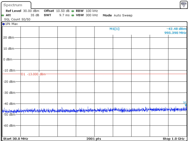
20MHz_15kHz_3460MHz_DFT-s-OFDM QPSK_RB1@105 -42.48 dBm
