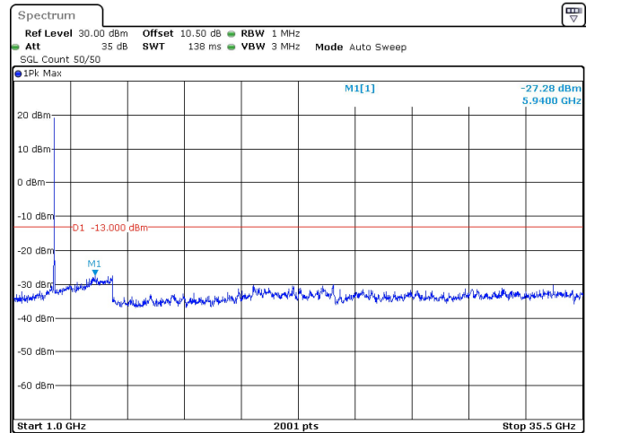
20MHz_15kHz_3460MHz_DFT-s-OFDM QPSK_RB100@0 -27.28 dBm
