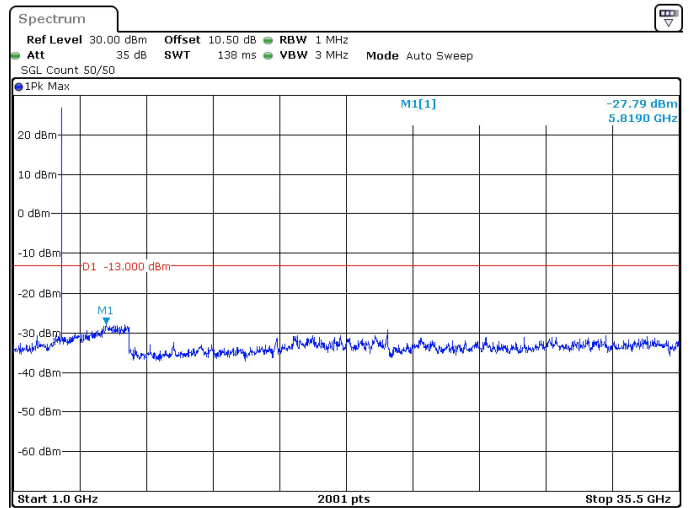
10MHz_30kHz_3500MHz_DFT-s-OFDM QPSK_RB1@0 -27.79 dBm
