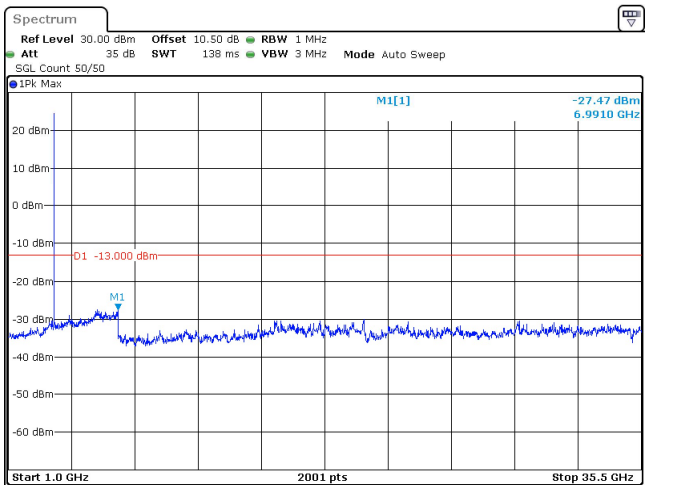
10MHz_30kHz_3500MHz_DFT-s-OFDM QPSK_RB1@23 -27.47 dBm
