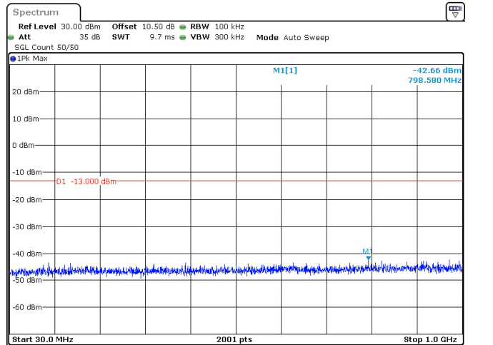
10MHz_30kHz_3545MHz_DFT-s-OFDM QPSK_RB24@0 -42.66 dBm
