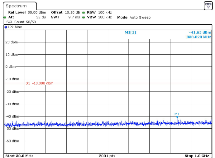
10MHz_30kHz_3500MHz_DFT-s-OFDM QPSK_RB1@23 -41.65 dBm
