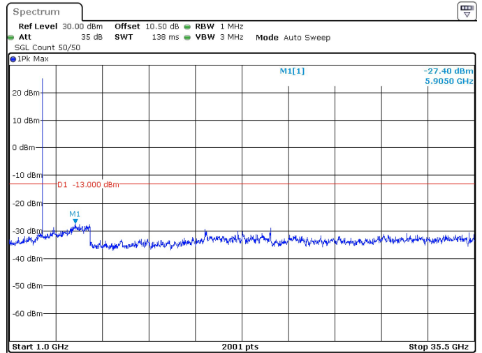
10MHz_30kHz_3455MHz_DFT-s-OFDM QPSK_RB1@23 -27.40 dBm
