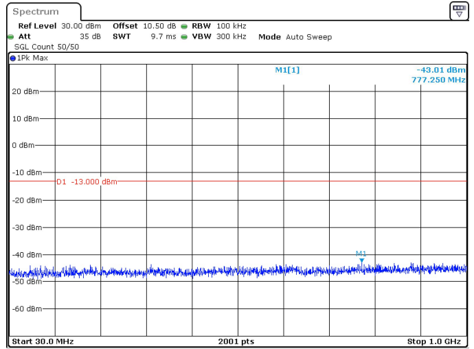
10MHz_30kHz_3455MHz_DFT-s-OFDM QPSK_RB1@0 -43.01 dBm
