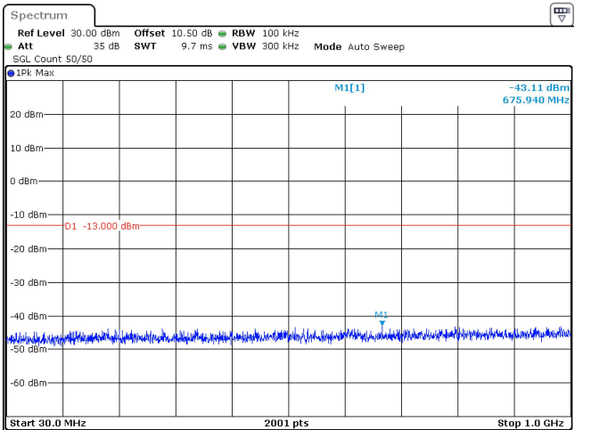
10MHz_30kHz_3455MHz_DFT-s-OFDM QPSK_RB1@23 -43.11 dBm
