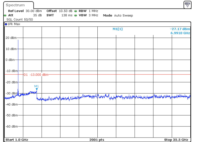
10MHz_15kHz_3545MHz_DFT-s-OFDM QPSK_RB50@0 -27.17 dBm
