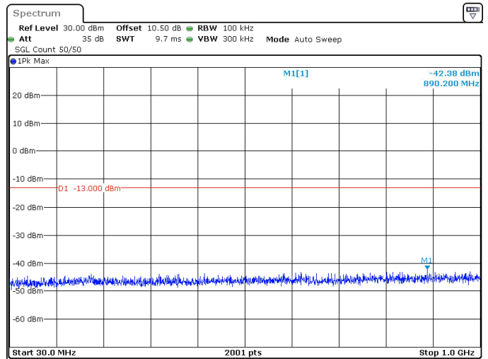
10MHz_15kHz_3500MHz_DFT-s-OFDM QPSK_RB1@0 -42.38 dBm
