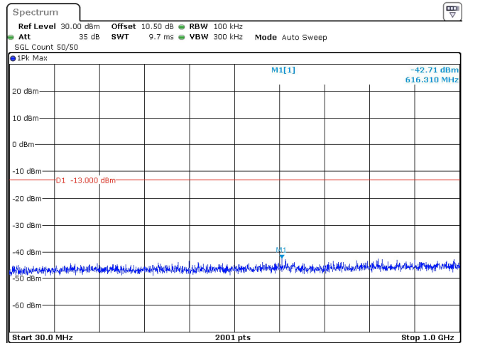
10MHz_30kHz_3455MHz_DFT-s-OFDM QPSK_RB24@0 -42.71 dBm
