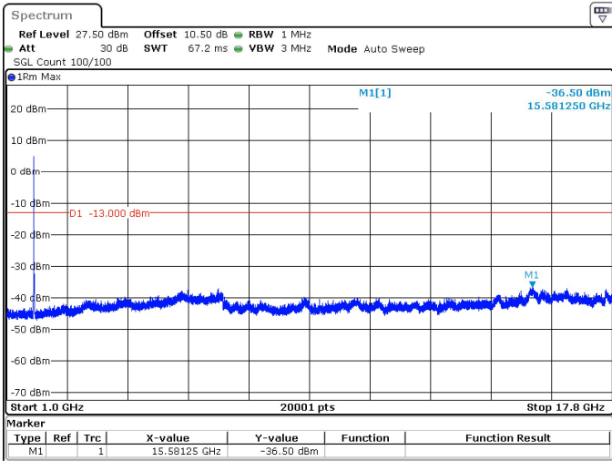
10MHz_15kHz_1745MHz_DFT-s-OFDM QPSK_RB50@0 -36.50 dBm
