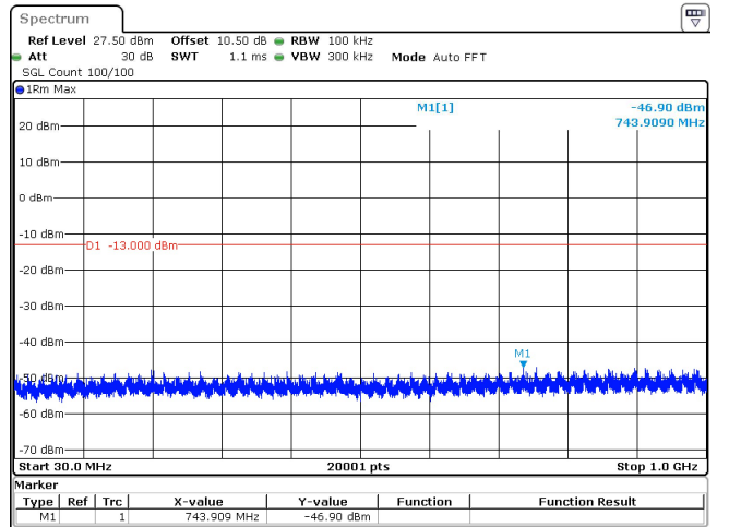
10MHz_15kHz_1745MHz_DFT-s-OFDM QPSK_RB50@0 -46.90 dBm
