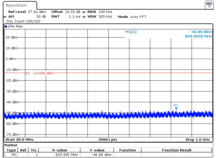
10MHz_15kHz_1745MHz_DFT-s-OFDM QPSK_RB1@0 -46.88 dBm
