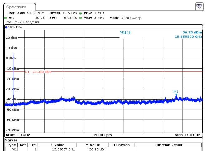
15MHz_15kHz_1717.5MHz_DFT-s-OFDM QPSK_RB75@0 -36.25 dBm
