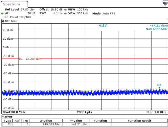
10MHz_15kHz_1715MHz_DFT-s-OFDM QPSK_RB50@0 -47.21 dBm
