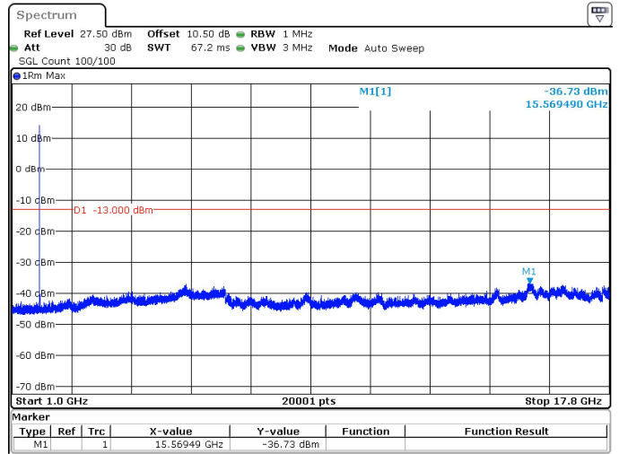
10MHz_15kHz_1775MHz_DFT-s-OFDM QPSK_RB1@0 -36.73 dBm
