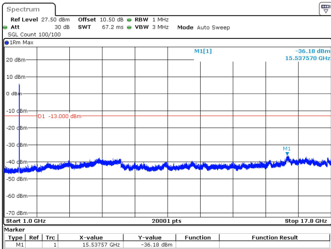
10MHz_15kHz_1775MHz_DFT-s-OFDM QPSK_RB50@0 -36.18 dBm
