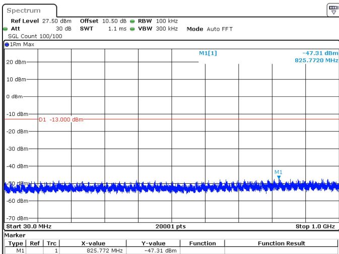
15MHz_15kHz_1717.5MHz_DFT-s-OFDM QPSK_RB1@0 -47.31 dBm
