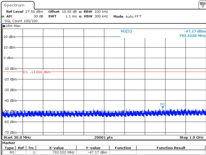
10MHz_15kHz_1775MHz_DFT-s-OFDM QPSK_RB1@0 -47.17 dBm
