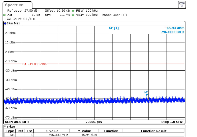
10MHz_15kHz_1775MHz_DFT-s-OFDM QPSK_RB50@0 -46.94 dBm
