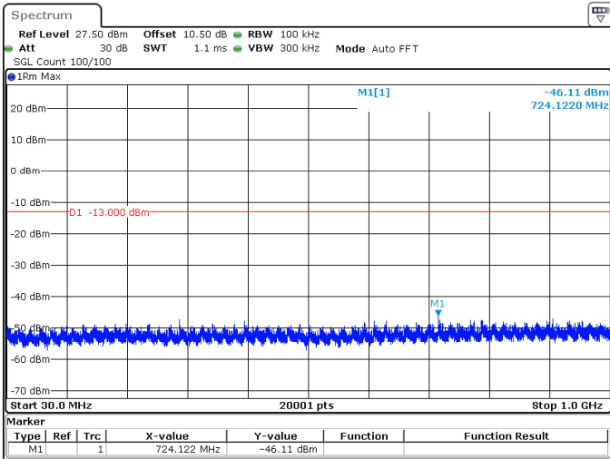
5MHz_15kHz_1745MHz_DFT-s-OFDM QPSK_RB25@0 -46.11 dBm
