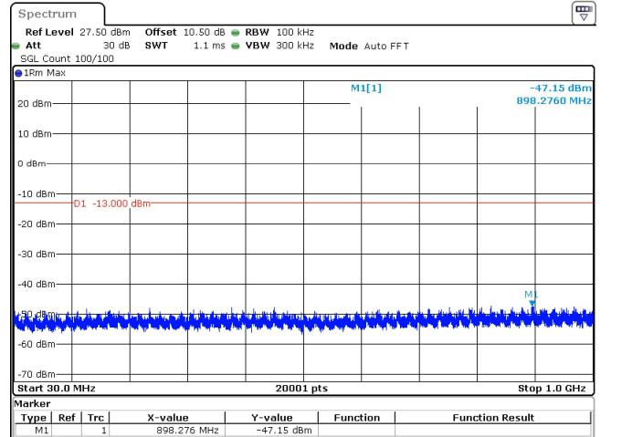
5MHz_15kHz_1777.5MHz_DFT-s-OFDM QPSK_RB25@0 -47.15 dBm
