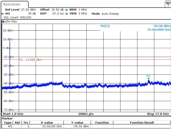
5MHz_15kHz_1777.5MHz_DFT-s-OFDM QPSK_RB25@0 -35.56 dBm
