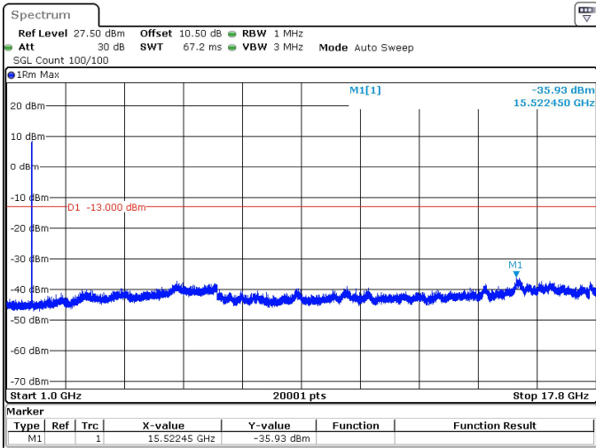
5MHz_15kHz_1712.5MHz_DFT-s-OFDM QPSK_RB25@0 -35.93 dBm
