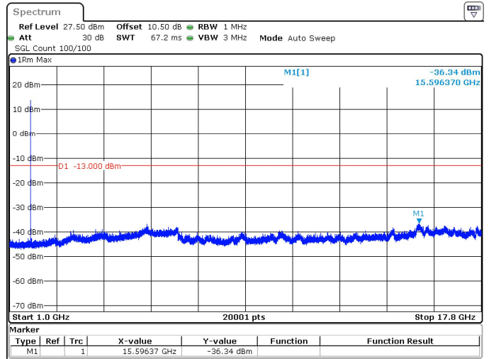
5MHz_15kHz_1745MHz_DFT-s-OFDM QPSK_RB1@0 -36.34 dBm
