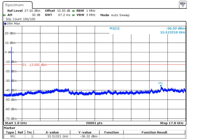
10MHz_15kHz_1715MHz_DFT-s-OFDM QPSK_RB50@0 -36.32 dBm
